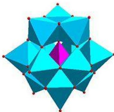
Figure I-1 : Structure de l'HPA de Keggin
