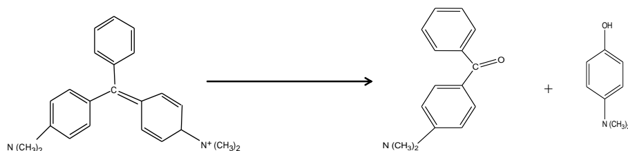
Figure V-16: Produits d'oxydation du vert de malachite après 2 h de réaction
