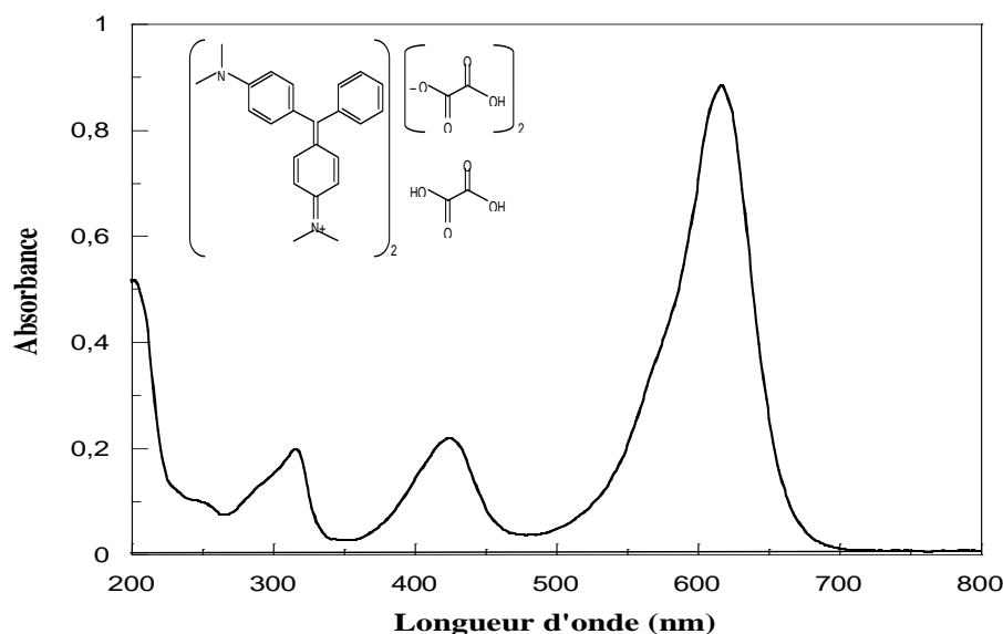
Figure V-2: Spectre d'absorption UV-visible du Vert de Malachite (VM) à pH = 3
