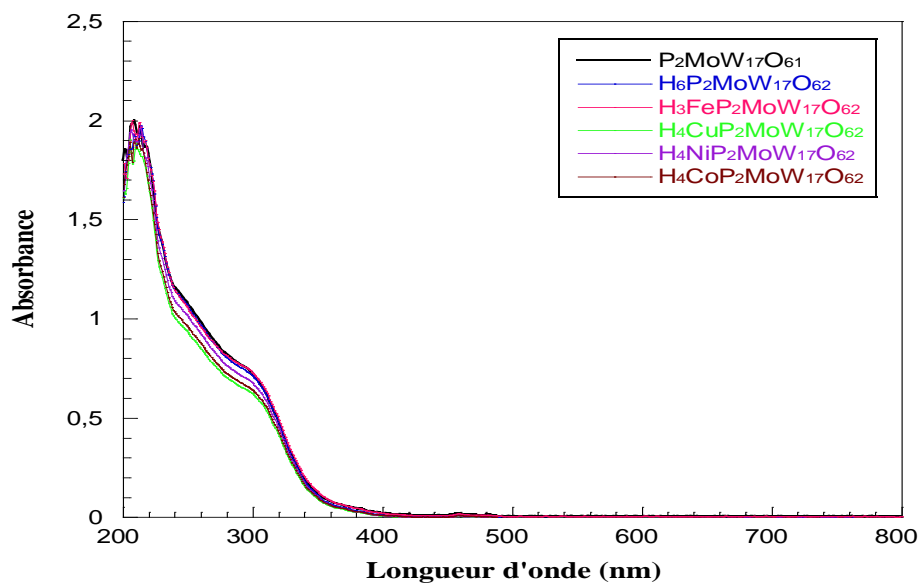
Figure IV-10: Spectre d'absorption UV-visible des composés synthétisés superposés à 0,03 \times 10^{-3} \text{ mmol.L}^{-1} : \alpha_2P_2MoW_{17}O_{61} , \alpha_2H_6P_2MoW_{17}O_{62} , \alpha_2H_3FeP_2MoW_{17}O_{62} , \alpha_2H_4CuP_2MoW_{17}O_{62} , \alpha_2H_4NiP_2MoW_{17}O_{62} et \alpha_2H_4CoP_2MoW_{17}O_{62} .
