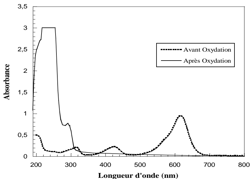
Figure V-14: Spectre d'absorption UV-visible du Vert de Malachite (VM) avant et après oxydation
