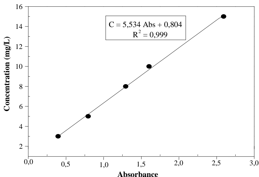
Figure V-5: Courbe d'étalonnage du Vert de Malachite
