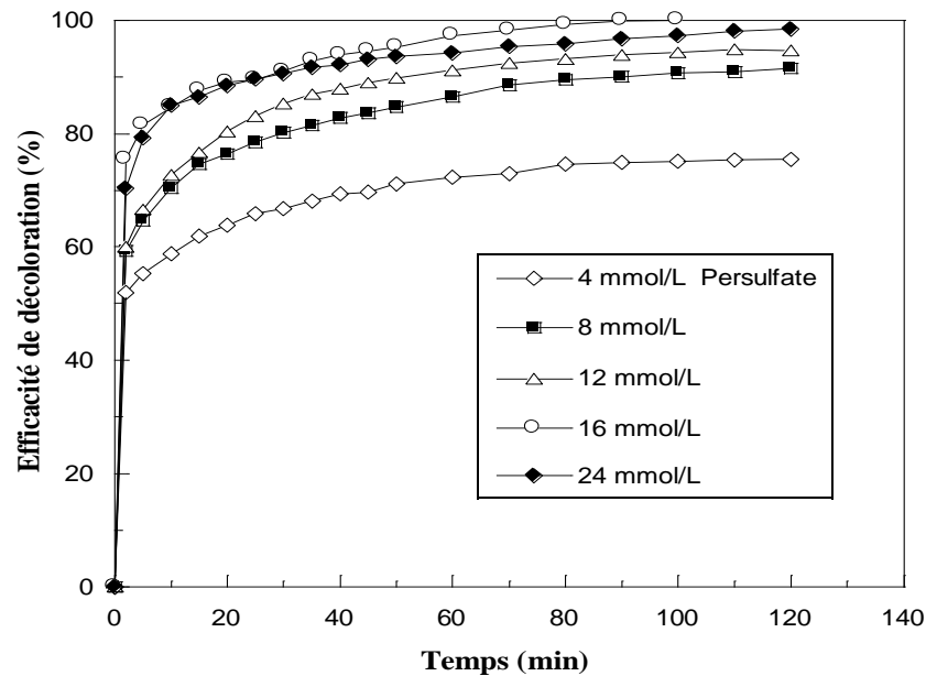
Figure V-32 : Décoloration de l'Écarlate solophényl BNLE par différentes concentrations de \text{S}_2\text{O}_8^{2-} dans le système \text{S}_2\text{O}_8^{2-}/\text{H}_3\text{FeP}_2\text{MoW}_{17}\text{O}_{62} (Conditions : V_R = 100 \text{ mL} , T = 20 \text{ °C} [\text{RS}]_0 = 4,25 \times 10^{-2} \text{ mol.L}^{-1} , \text{pH} = 3 , [\text{H}_3\text{FeP}_2\text{MoW}_{17}\text{O}_{62}] = 0,1 \text{ mol.L}^{-1} , [\text{S}_2\text{O}_8^{2-}] = 4, 8, 12, 16 et 24 \text{ mmol.L}^{-1} )
