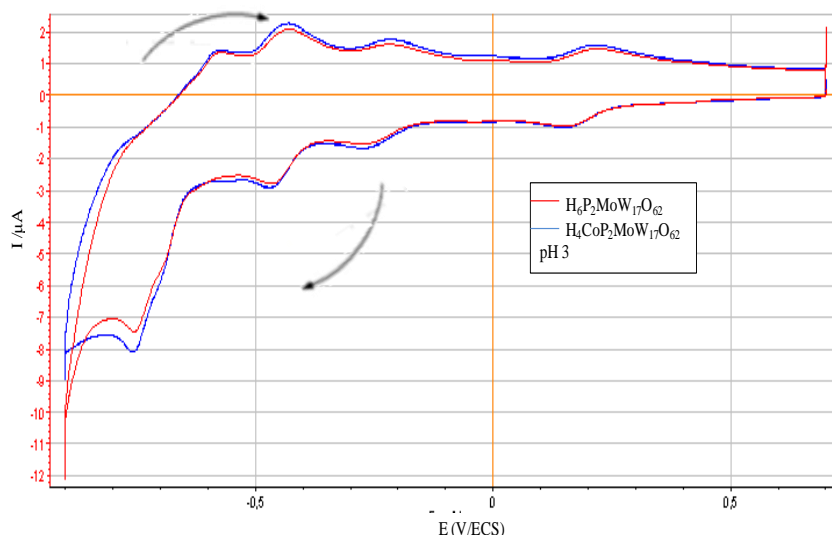
Figure IV-15 : Voltammogramme cyclique du \alpha_2\text{H}_4\text{CoP}_2\text{MoW}_{17}\text{O}_{62} et du \alpha_2\text{H}_6\text{P}_2\text{MoW}_{17}\text{O}_{62}
