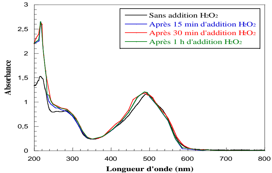
Figure V-21 : Effet de \text{H}_2\text{O}_2 ( 1 \text{ mmol.L}^{-1} ) sur l'Écarlate Solophényl ( 5 \times 10^{-3} \text{ mmol.L}^{-1} )
