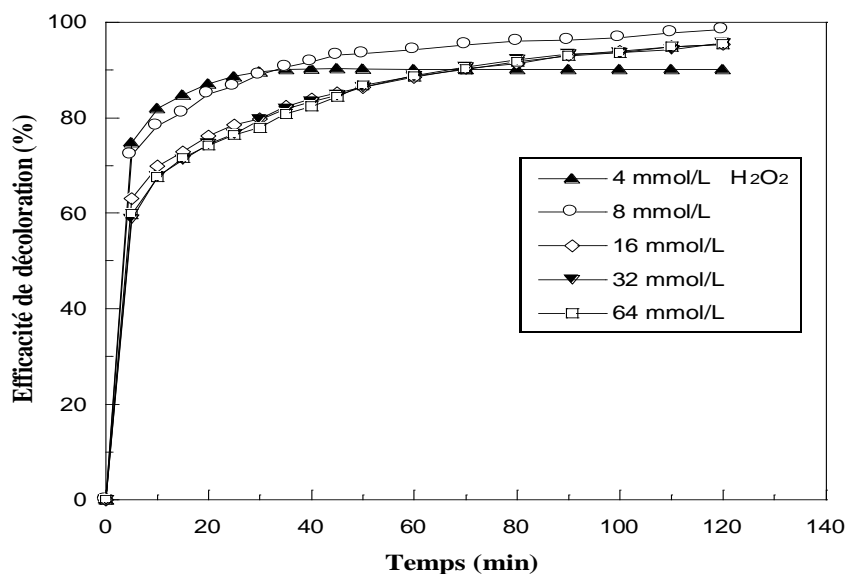
Figure V-26 : Décoloration de l'Écarlate solophényl BNLE à différentes concentrations en \text{H}_2\text{O}_2 dans le système \text{H}_2\text{O}_2/\text{H}_3\text{FeP}_2\text{MoW}_{17}\text{O}_{62} (Conditions : V_R = 100 \text{ mL} , [\text{RS}]_0 = 4,25 \times 10^{-2} \text{ mol.L}^{-1} , \text{pH} = 3 , T = 20 \text{ }^\circ\text{C} , [\text{H}_3\text{FeP}_2\text{MoW}_{17}\text{O}_{62}] = 0,1 \text{ mol.L}^{-1} , [\text{H}_2\text{O}_2] = 4, 8, 16, 24 \text{ et } 64 \text{ mmol.L}^{-1} )
