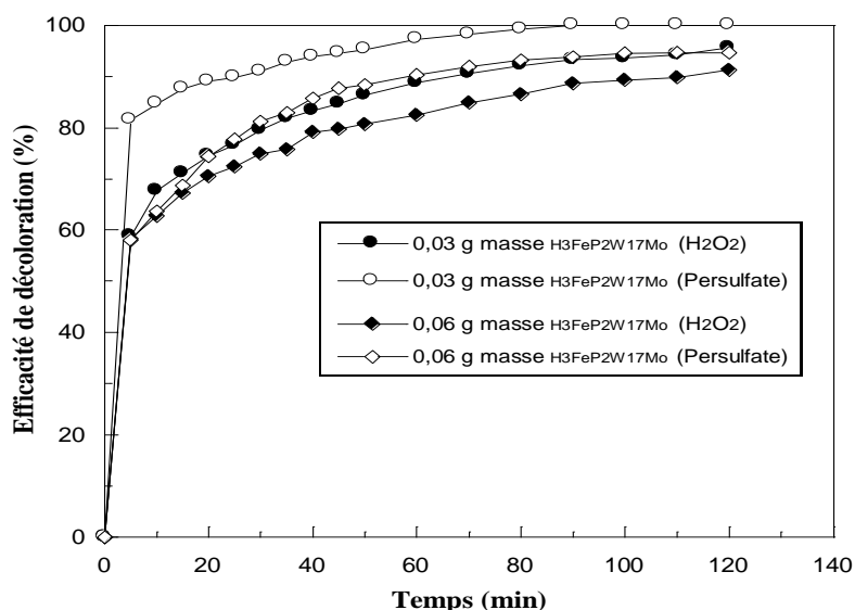
Figure V-38 : Comparaison de l'efficacité des deux systèmes \text{H}_2\text{O}_2/\text{H}_3\text{FeP}_2\text{MoW}_{17}\text{O}_{62} et \text{S}_2\text{O}_8^{2-}/\text{H}_3\text{FeP}_2\text{MoW}_{17}\text{O}_{62} à la décoloration du RS à différentes masses de catalyseurs
