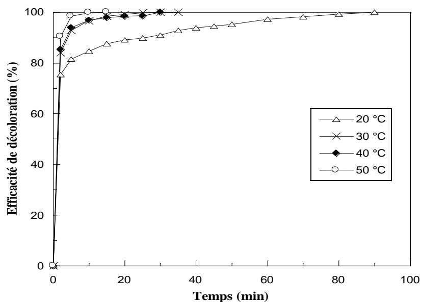
Figure V-34 : Décoloration de l'Écarlate solophényl BNLE à différentes températures dans le système \text{S}_2\text{O}_8^{2-}/\text{H}_3\text{FeP}_2\text{MoW}_{17}\text{O}_{62} (Conditions : V_R = 100 \text{ mL} , [\text{RS}]_0 = 4,25 \times 10^{-2} \text{ mol.L}^{-1} , \text{pH} = 3 , [\text{S}_2\text{O}_8^{2-}] = 16 \text{ mmol.L}^{-1} , [\text{H}_3\text{FeP}_2\text{MoW}_{17}\text{O}_{62}] = 0,1 \text{ mol.L}^{-1} , T = 20, 30, 40 \text{ et } 50 \text{ °C} )
