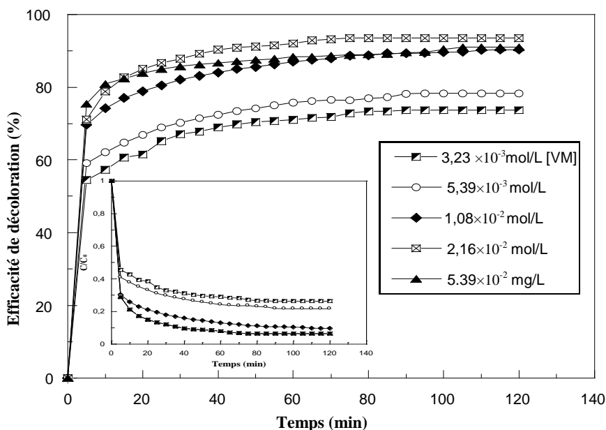
Figure V-11: Décoloration du vert de malachite à différentes concentration initiale du colorant par le système catalytique Fenton-like (Condition : V_R = 100 mL, T = 30 °C, pH = 3 , [H_2O_2] = 0,31 mol.L -1 , [H_3FeP_2MoW_{17}O_{62}] = 0,1 mol.L -1 , [VM]_0 = 3,23 \times 10^{-3} , 5,39 \times 10^{-3} , 1,08 \times 10^{-2} , 2,16 \times 10^{-2} et 5,39 \times 10^{-2} mol.L -1 )
