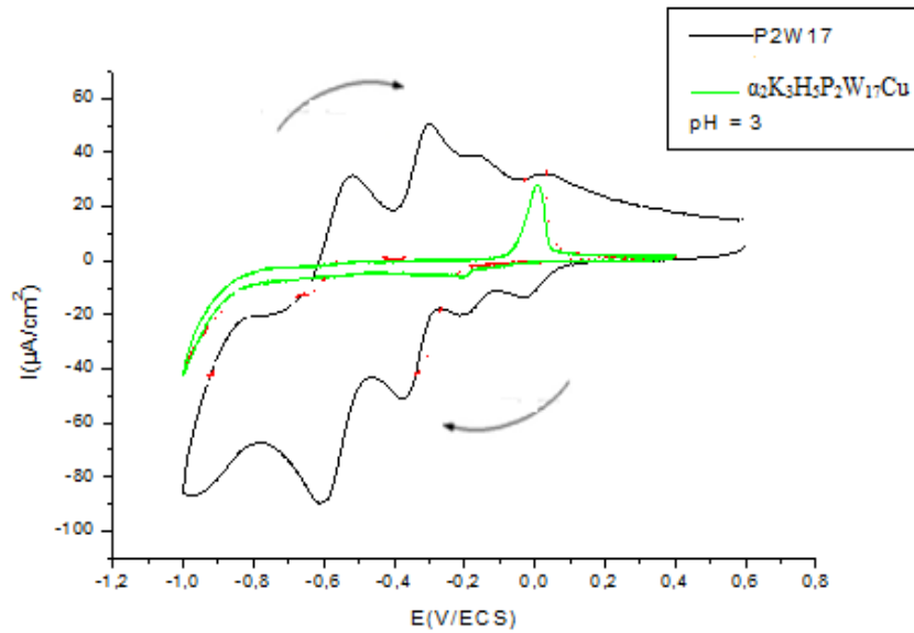
Figure IV-16: Voltamogramme cyclique du [(\alpha_2\text{H}_5\text{P}_2\text{W}_{17}\text{O}_{61})\text{Cu}]^{3-} et du \alpha_2\text{P}_2\text{W}_{17}\text{O}_{61}
