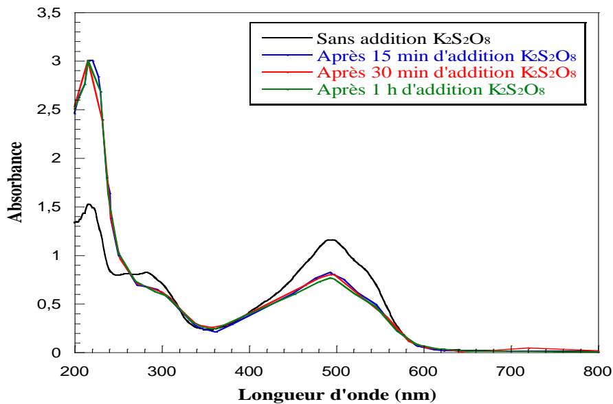
Figure V-22 : Effet de \text{K}_2\text{S}_2\text{O}_8 ( 1 \text{ mmol.L}^{-1} ) sur l'Écarlate Solophényl ( 5 \times 10^{-3} \text{ mmol.L}^{-1} )
