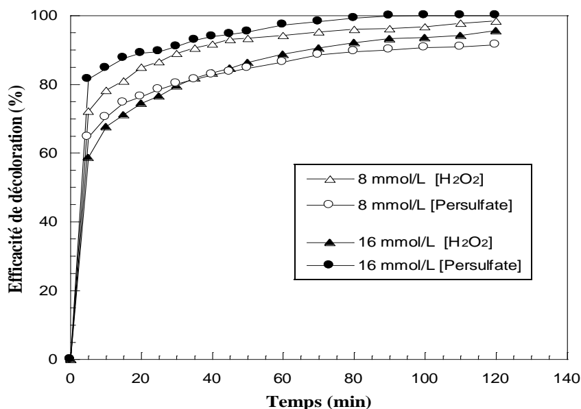
Figure V-36 : Comparaison de la décoloration du RS, par les deux systèmes
