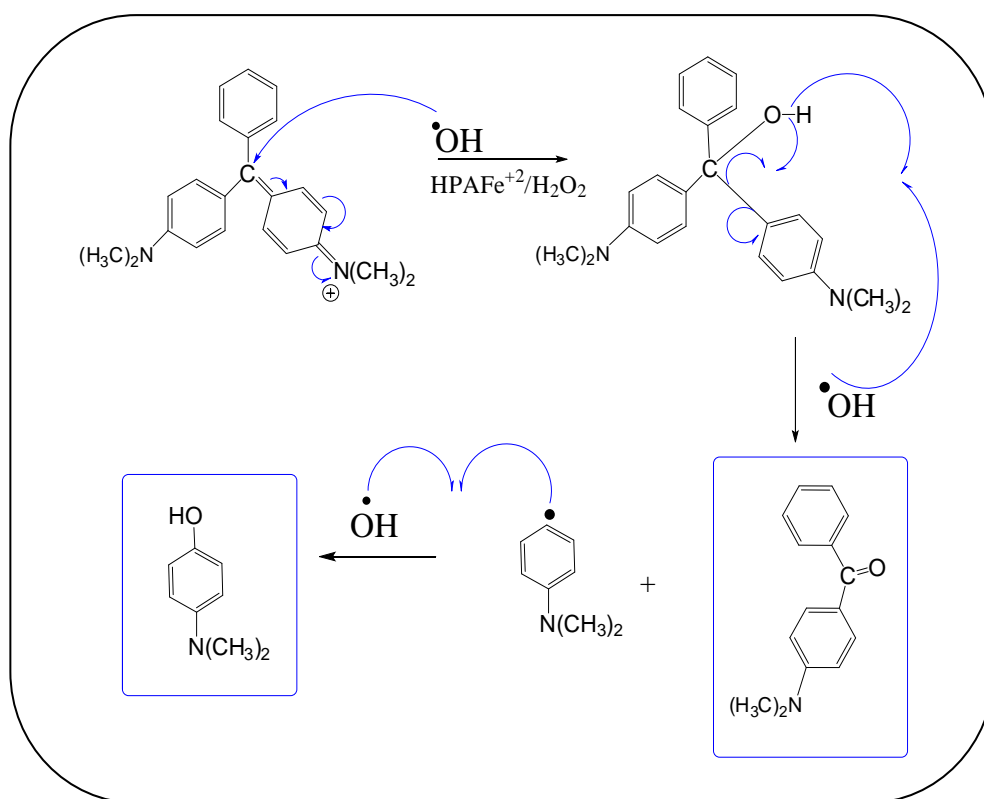
Figure V-17: Mécanisme de dégradation du vert de malachite après 2 h de réaction
