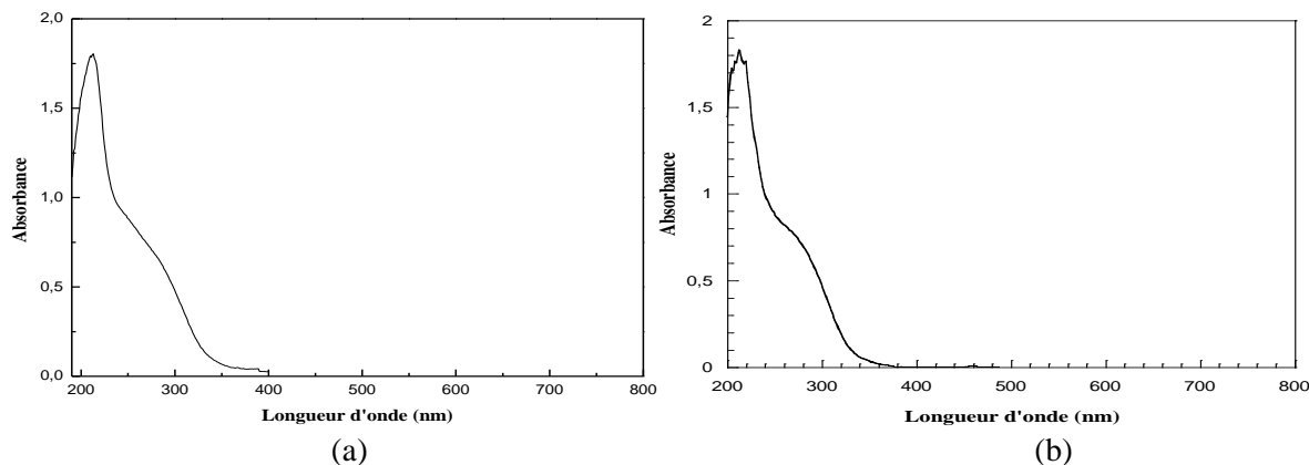
Figure IV-9: Spectre d'absorption UV-visible du composé à 0,03 \times 10^{-3} \text{ mmol.L}^{-1} de (a) \alpha P_2W_{18}O_{62} et (b) \alpha_2P_2W_{17}O_{61} .
