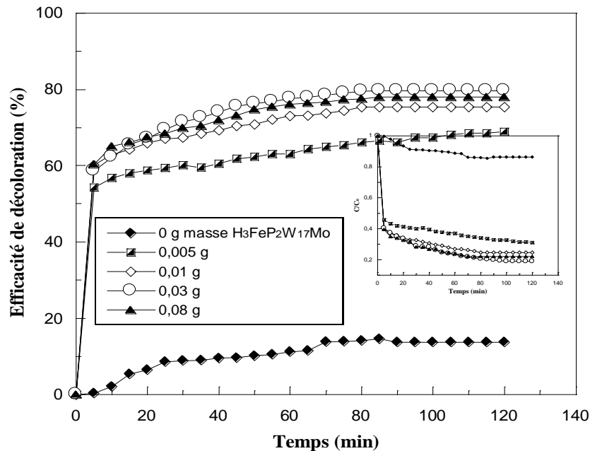
Figure V-8: Décoloration du vert de malachite à différentes masse du catalyseur par le système catalytique Fenton-like (Condition : V_R = 100 \text{ mL} , [\text{VM}]_0 = 5,39 \times 10^{-3} \text{ mol.L}^{-1} , pH = 3, T = 25 \text{ }^\circ\text{C} , [\text{H}_2\text{O}_2] = 0,08 \text{ mol.L}^{-1} , m_{\text{H}_3\text{FeP}_2\text{MoW}_{17}\text{O}_{62}} = 0, 0,005; 0,01; 0,03 \text{ et } 0,08 \text{ g} )
