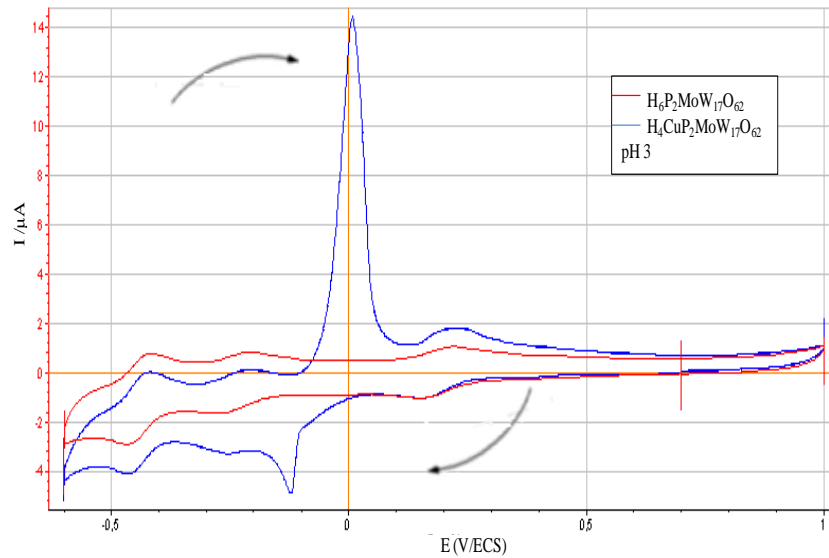
Figure IV-13: Voltamogramme cyclique du \alpha_2\text{H}_4\text{CuP}_2\text{MoW}_{17}\text{O}_{62} et du \alpha_2\text{H}_6\text{P}_2\text{MoW}_{17}\text{O}_{62}
