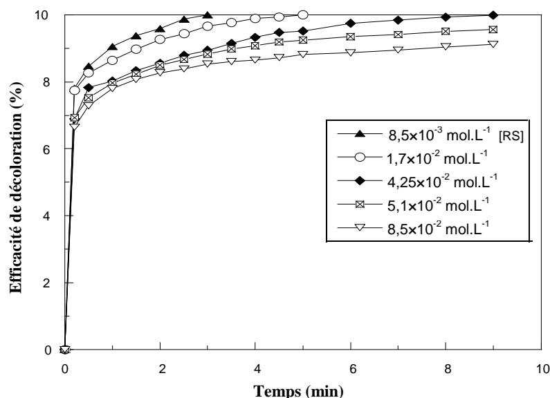
Figure V-33 : Décoloration du rouge solophényl BNLE à différentes concentrations initiales du colorant dans le système S_2O_8^{2-}/H_3FeP_2MoW_{17}O_{62} (Conditions : V_R = 100 \text{ mL} , pH = 3 , T = 20 \text{ }^\circ\text{C} , [S_2O_8^{2-}] = 16 \text{ mmol.L}^{-1} , [H_3FeP_2MoW_{17}O_{62}] = 0,1 \text{ mol.L}^{-1} , [RS]_0 = 8,5 \times 10^{-3} , 1,7 \times 10^{-2} , 4,25 \times 10^{-2} , 5,1 \times 10^{-2} et 8,5 \times 10^{-2} \text{ mol.L}^{-1} )
