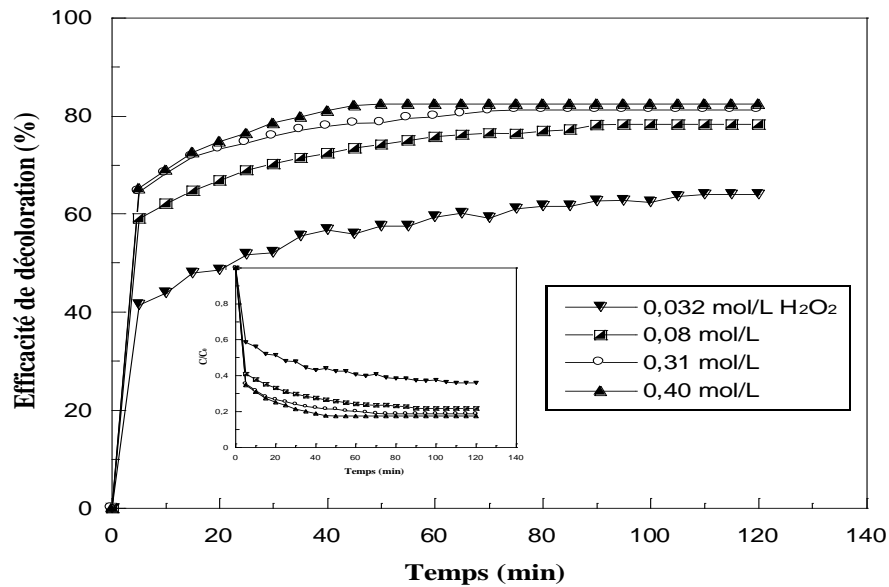
Figure V-9: Décoloration du vert de malachite à différentes concentration en \text{H}_2\text{O}_2 par le système catalytique Fenton-like (Condition : V_R = 100 \text{ mL} , [\text{VM}]_0 = 5,39 \times 10^{-3} \text{ mol.L}^{-1} , \text{pH} = 3 , T = 25 \text{ }^\circ\text{C} , [\text{H}_3\text{FeP}_2\text{MoW}_{17}\text{O}_{62}] = 0,1 \text{ mol.L}^{-1} , [\text{H}_2\text{O}_2] = 0,032; 0,08; 0,31 et 0,40 \text{ mol.L}^{-1} )
