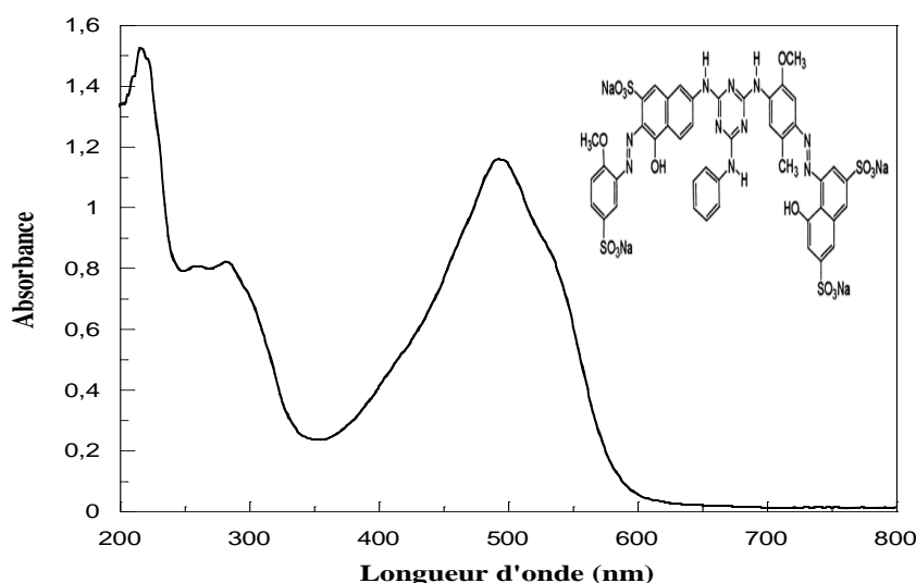
Figure V-19 : Spectre d'absorption UV-visible de l'Écarlate Solophényle BNLE (RS)
