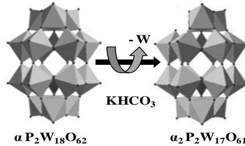
Figure IV-2: Synthèse de [\alpha_2\text{P}_2\text{W}_{17}\text{O}_{61}]^{10-}
