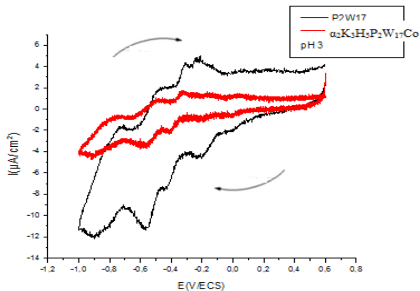
Figure IV-17: Voltamogramme cyclique du [(\alpha_2\text{H}_5\text{P}_2\text{W}_{17}\text{O}_{61})\text{Co}]^{3-} et du \alpha_2\text{P}_2\text{W}_{17}\text{O}_{61}
