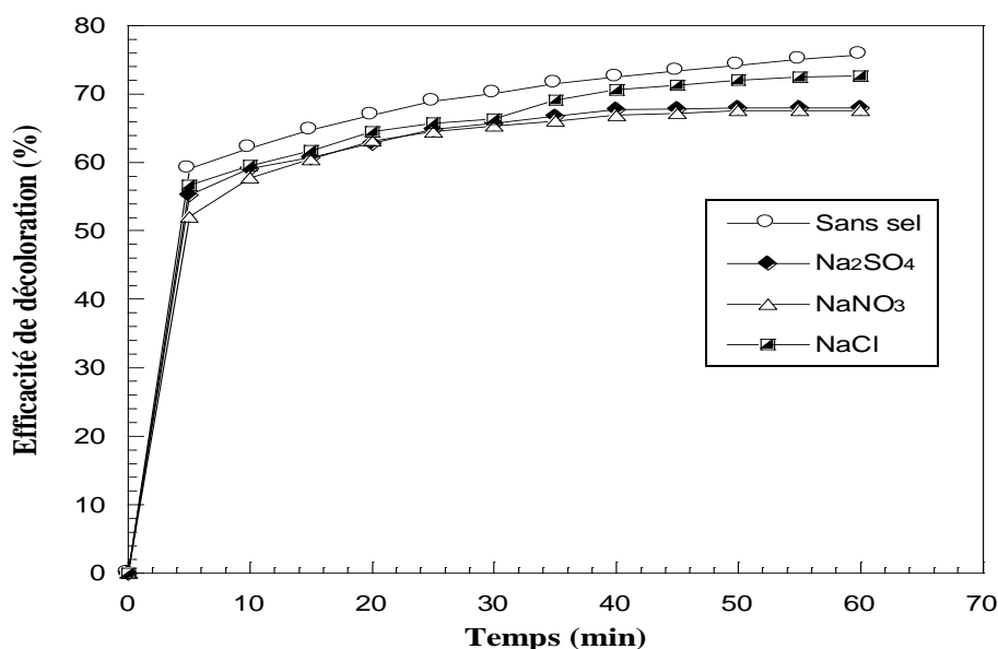
Figure V-13: Décoloration du vert de malachite en présence de différents anions inorganiques par le système catalytique Fenton-like (Condition : V_R = 100 \text{ mL} , \text{pH} = 3 , T = 30 \text{ }^\circ\text{C} , [\text{VM}]_0 = 5,39 \text{ mg.L}^{-1} , [\text{H}_2\text{O}_2] = 0,31 \text{ mol.L}^{-1} , [\text{H}_3\text{FeP}_2\text{MoW}_{17}\text{O}_{62}] = 0,1 \text{ mol.L}^{-1} ,
