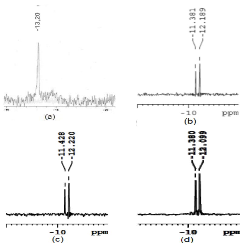
Figure IV-7: Spectres RMN du ^{31}\text{P} des HPAs: (a) \alpha_2\text{H}_3\text{FeP}_2\text{MoW}_{17}\text{O}_{62} , (b) \alpha_2\text{H}_4\text{CuP}_2\text{MoW}_{17}\text{O}_{62} , (c) \alpha_2\text{H}_4\text{NiP}_2\text{MoW}_{17}\text{O}_{62} , (d) \alpha_2\text{H}_4\text{CoP}_2\text{MoW}_{17}\text{O}_{62} .
