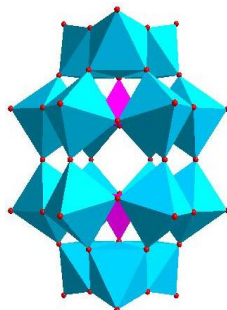
Figure I-3 : Structure de l'HPA de Dawson
