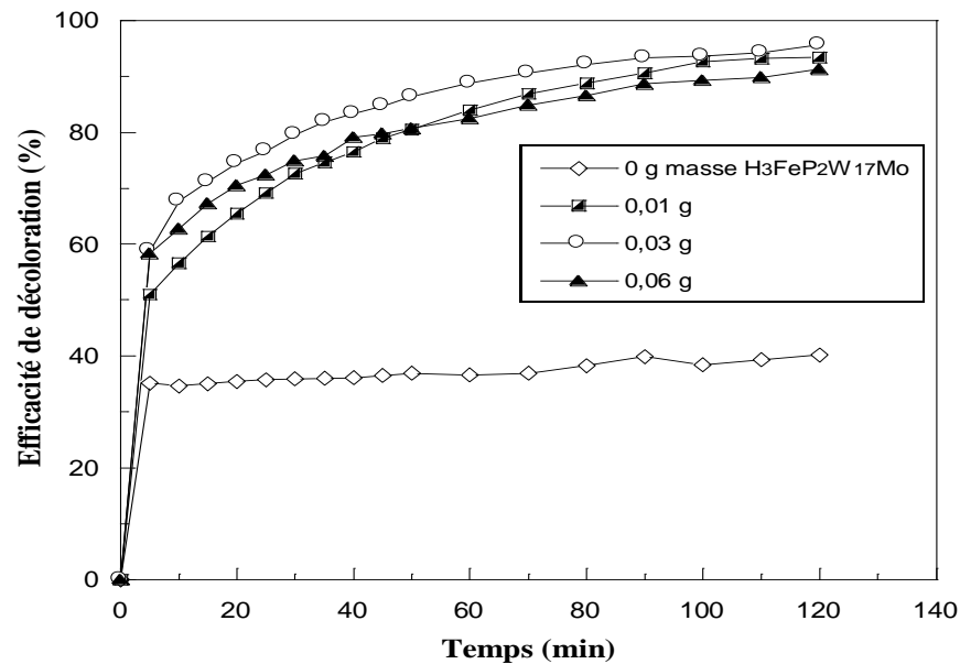
Figure V-25 : Décoloration de l'Écarlate solophényl BNLE à différentes masses du catalyseur dans le système \text{H}_2\text{O}_2/\text{H}_3\text{FeP}_2\text{MoW}_{17}\text{O}_{62} (Conditions : V_R = 100 \text{ mL} , [\text{RS}]_0 = 4,25 \times 10^{-2} \text{ mol.L}^{-1} , \text{pH} = 3 , T = 20 \text{ }^\circ\text{C} , [\text{H}_2\text{O}_2] = 16 \text{ mmol.L}^{-1} , m_{\text{H}_3\text{FeP}_2\text{MoW}_{17}\text{O}_{62}} = 0, 0,01, 0,03 \text{ et } 0,06 \text{ g} )
