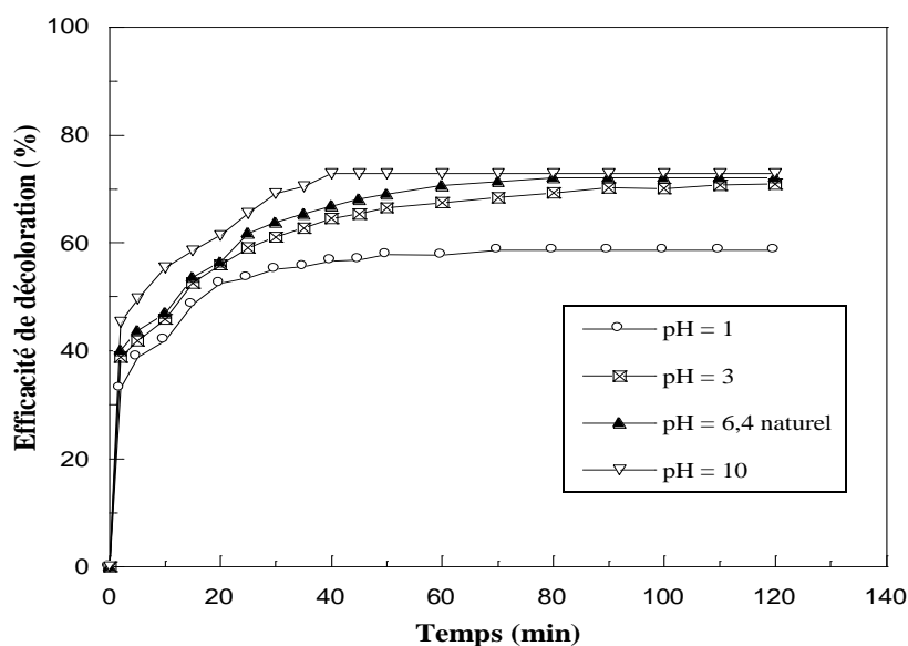
Figure V-30 : Décoloration de l'Écarlate solophényl BNLE à différents pH dans le système \text{S}_2\text{O}_8^{2-}/\text{H}_3\text{FeP}_2\text{MoW}_{17}\text{O}_{62} (Conditions: V_R = 100 \text{ mL} , [\text{RS}]_0 = 4,25 \times 10^{-2} \text{ mol.L}^{-1} , T = 20 \text{ }^\circ\text{C} , m_{\text{H}_3\text{FeP}_2\text{MoW}_{17}\text{O}_{62}} = 0,01 \text{ g} , [\text{S}_2\text{O}_8^{2-}] = 8 \text{ mmol.L}^{-1} , pH = 1 ; 3 ; 6,4 naturel ; 10)
