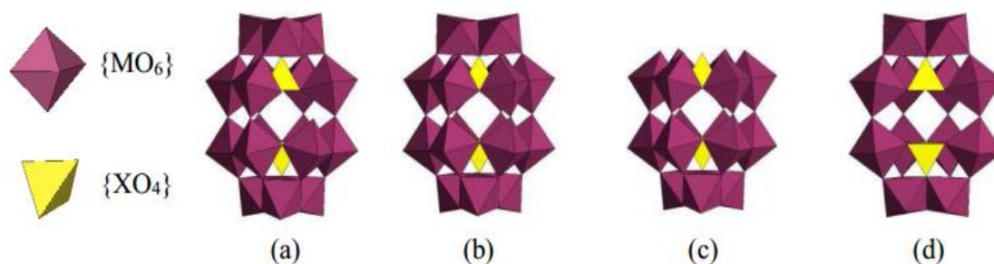
Figure I-4 : Les dérivés lacunaires de la structure de l'HPA de Dawson : (a) \alpha_1 P_2W_{17} , (b) \alpha_2 P_2W_{17} , (c) \alpha P_2W_{15} , (d) \alpha P_2W_{12} .
