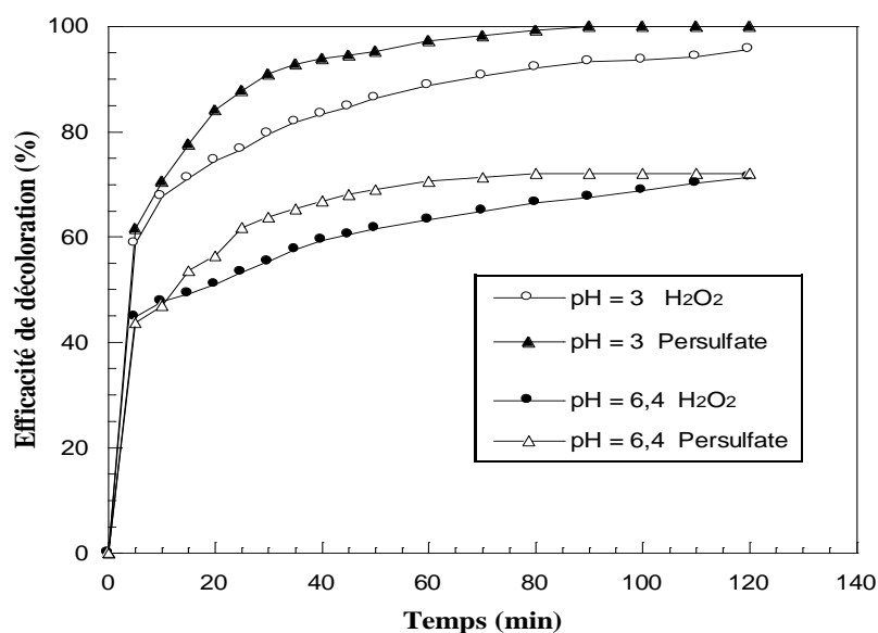
Figure V-37 : Comparaison de l'efficacité des deux systèmes \text{H}_2\text{O}_2/\text{H}_3\text{FeP}_2\text{MoW}_{17}\text{O}_{62} et \text{S}_2\text{O}_8^{2-}/\text{H}_3\text{FeP}_2\text{MoW}_{17}\text{O}_{62} à la décoloration du RS à pH 3 et pH naturel
