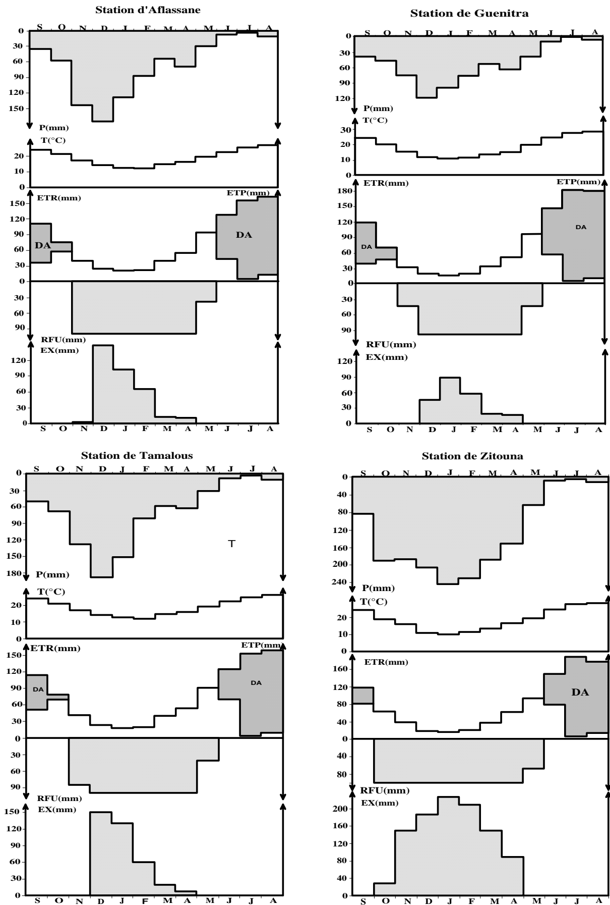
Figure 4.21. Représentation graphique du bilan de Thornthwaite.
