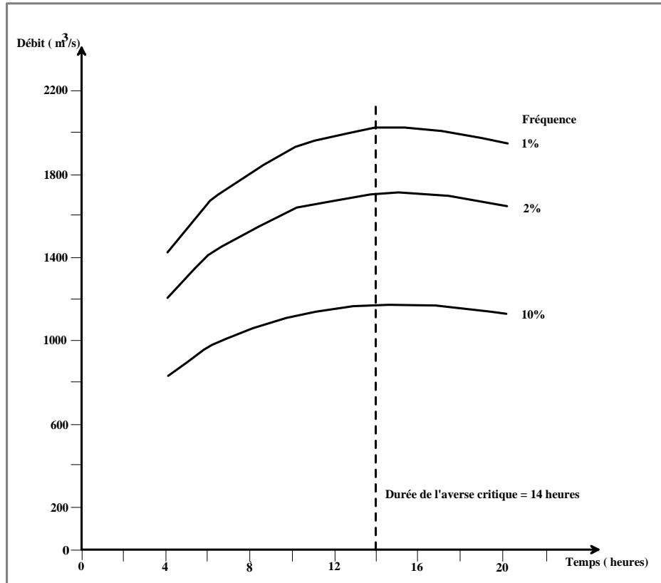
Figure 4.26. Choix de l'averse critique par la méthode de l'hydrogramme unitaire de l'Oued Guebli embouchure (d'après L'ANRH)
