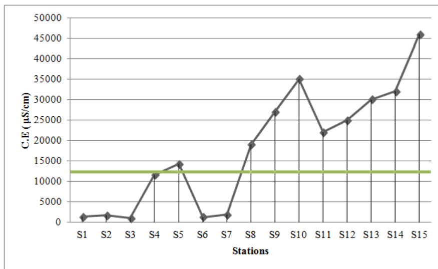
Figure 5.39. Courbe de la qualité des eaux de surface en fonction de la conductivité.
