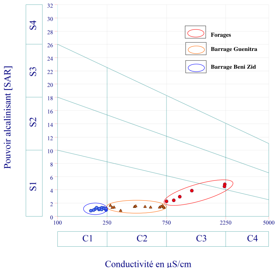
Figure.8.9. Classification des eaux des forages et des barrages du Guebli d'après le diagramme de Richards.
