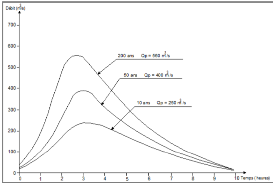
Figure 4.30. Hydrogrammes des crues de projet adoptées d’après les études de Ukrguidrovodkhoz.
