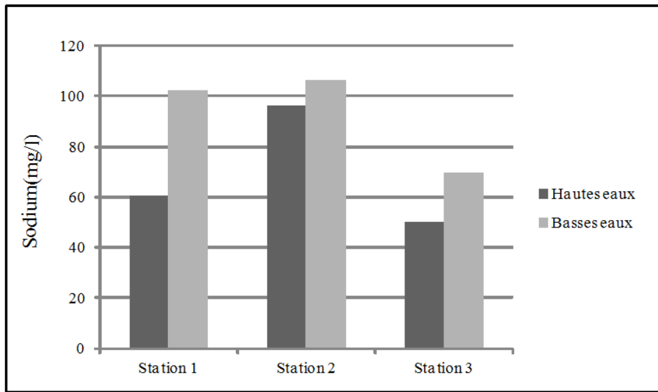
Figure 5.5. Concentrations du sodium dans les eaux de surface en amont du Guebli.
