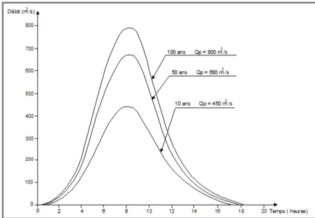
Figure 4.29. Hydrogrammes des crues de projet adoptées d'après les études de Acres -Tractionnel et de DEMRH.
