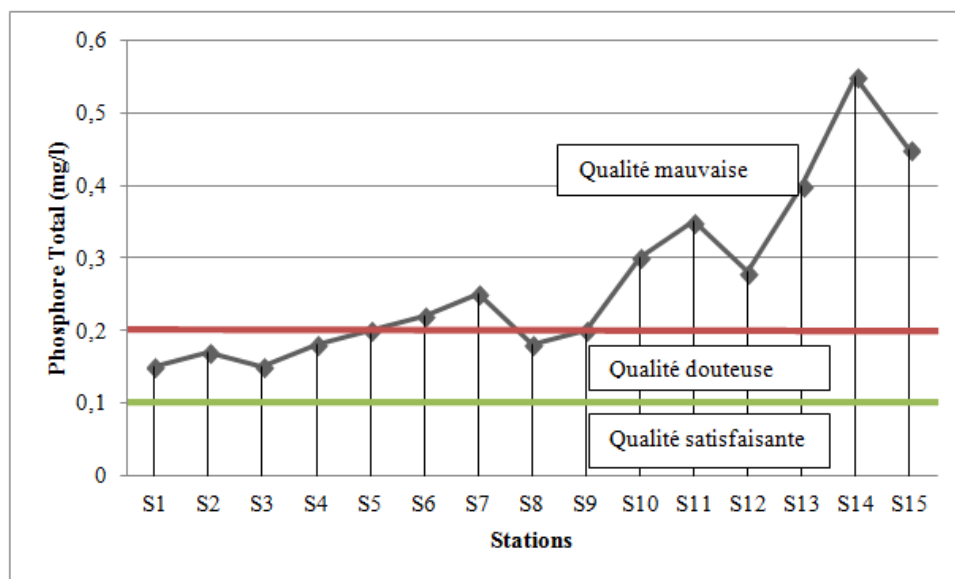
Figure 5.45. Courbe de la qualité des eaux du Guebli aval en fonction de Phosphore total.
