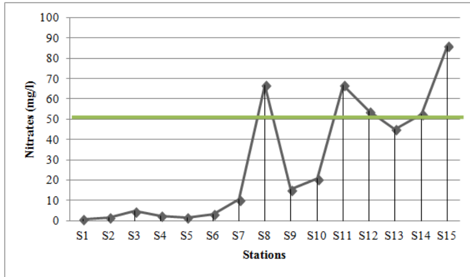
Figure 5.44. Courbe de la qualité des eaux du Guebli aval en fonction des nitrates.
