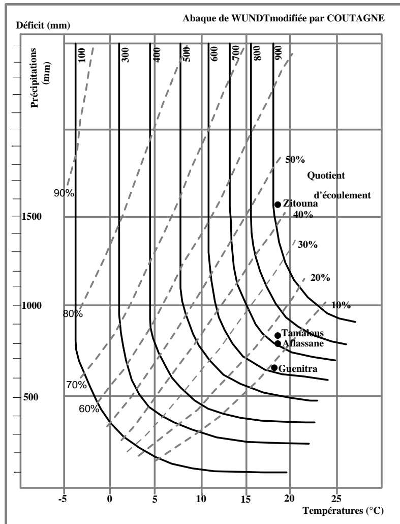
Figure 4.20. Évaluation de l'écoulement et du déficit d'écoulement en fonction des Températures moyennes et des précipitations
