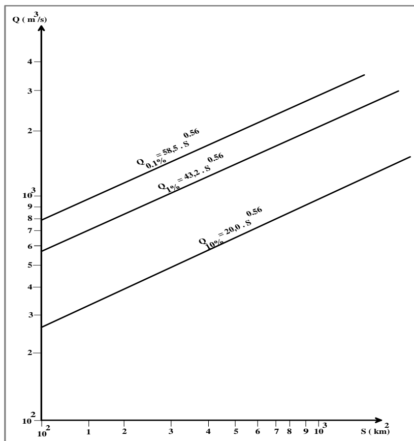
Figure 4.27. Application de la formule de Coutagne (d'après l'A.N.R.H)
