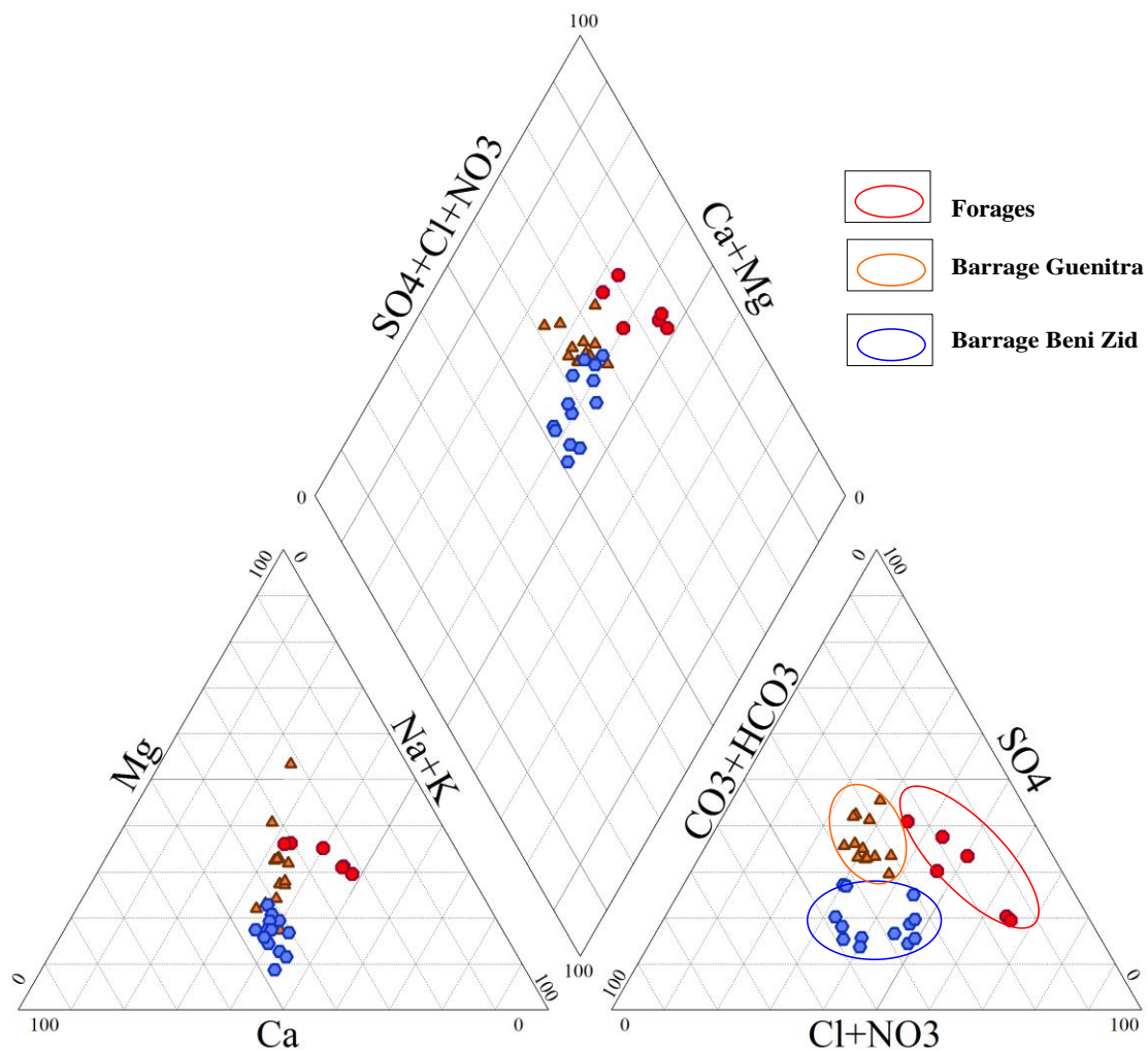
Figure 8.8. Faciès chimiques des eaux pour les forages et barrages du Guebli.
