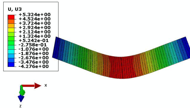
e) Cas de 12 plis [-75°/-60°/-45°/-30°/-15°/0°/15°/30°/45°/60°/ 75°/90°]
