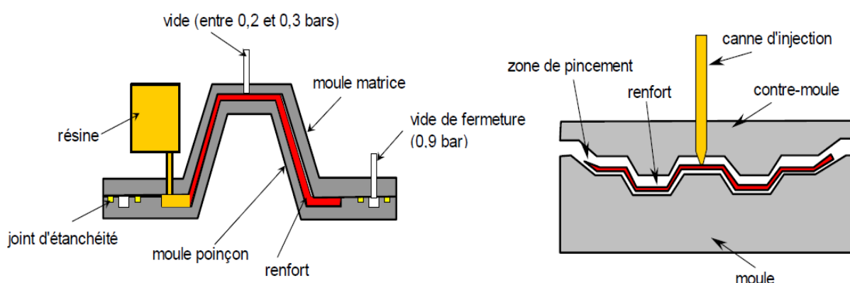
Fig. 1.10 : Moulage par RTM
