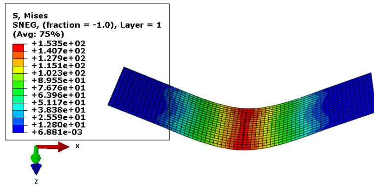
a) Cas de 3 plis [-60°/0°/60°]
