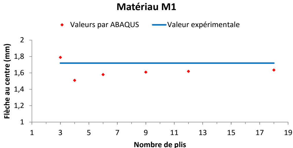
Fig. 4.27 : Comparaison des flèches au centre obtenues par ABAQUS et par l'expérimental pour le matériau M1
