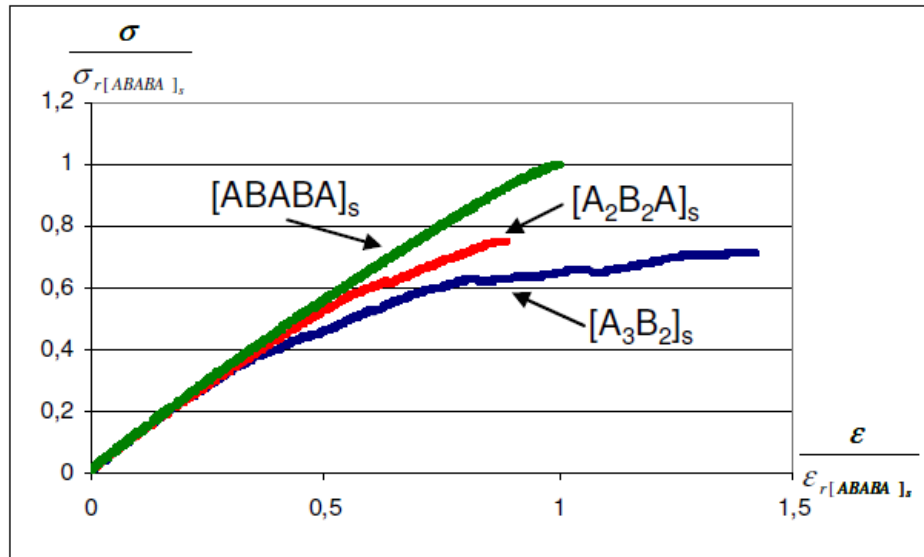
Fig. 1.19 : Courbes contraintes – déformations des essais de traction quasi-statique à rupture sur les multicouches polymère/composite avec trois drapages différents [29].
