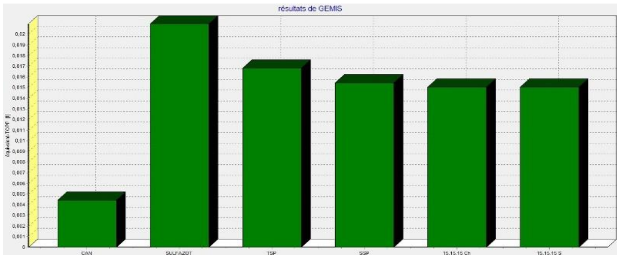
Fig. C. Présentation graphique de PPOT pour tous les fertilisants en COVNM eq
