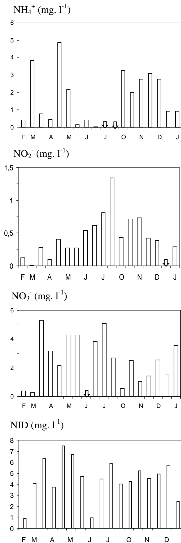
Figure 5 : Variations saisonnières des teneurs de l'azote ammoniacal, des nitrites et des nitrates dans la Seybouse durant l'année 2005. ↓ : pas de données.
