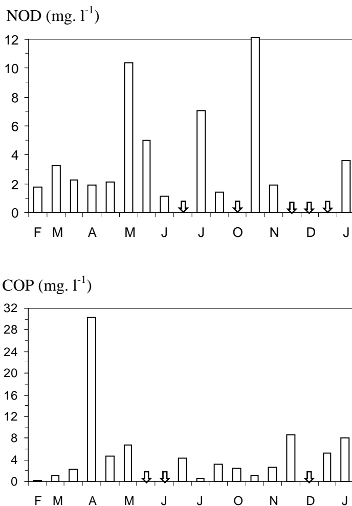
Figure 8 : Variations saisonnières des teneurs de l'azote organique dissous (NOD) et du carbone organique particulaire (COP) dans oued Seybouse en 2005. ↓ : pas de données.
