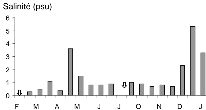
Figure 4 : Variations saisonnières de la salinité des eaux dans à l’embouchure de Seybouse en 2005. ↓ : pas de données.
