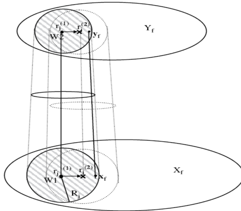
Figure 2.8 L'apprentissage adaptatif dans EFuNN: un neurone de règle représente une association de deux hypersphères de l'espace d'entrée floue et de l'espace de sortie floue; Le neurone de règle r_j 'se déplace' d'une position r_j^{(1)} à r_j^{(2)} pour accommoder le nouvel exemple d'entrée-sortie (x_f, y_f) [KAS 07].
