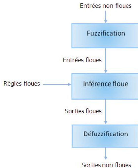
Figure 1.7 : Fonctionnement d'un Système Flou
