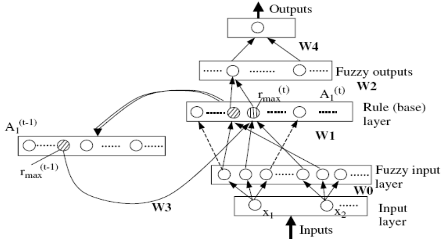
Figure 2.7 Un exemple d'EFuNN avec une mémoire à court terme réalisée en tant que connexion de rétroaction [KAS 01b].
