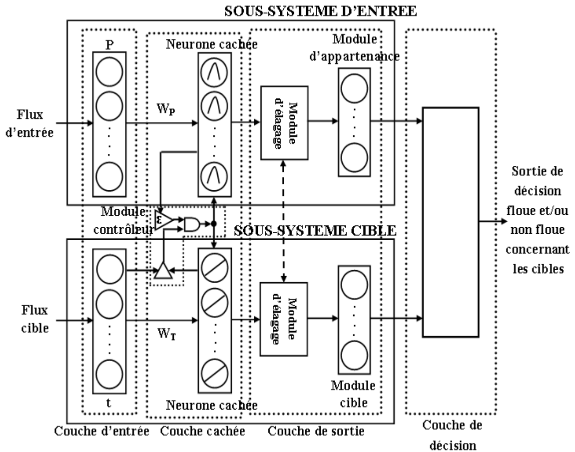
Figure 2.3 : Architecture du réseau du classifieur ILFN dans le mode d'apprentissage [YEN 99]
