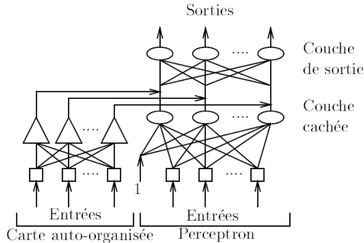
Figure 2.5 : Architecture hybride du réseau PAO
