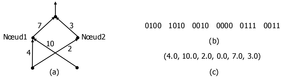
Figure 1.10 : (a) Un RNA avec poids de connexion montré; (b) Une représentation binaire des poids, supposant que chaque poids est représenté par quatre bits, le poids 0000 n'indique aucune connexion entre deux nœuds. (c) Une représentation en nombres réels des poids
