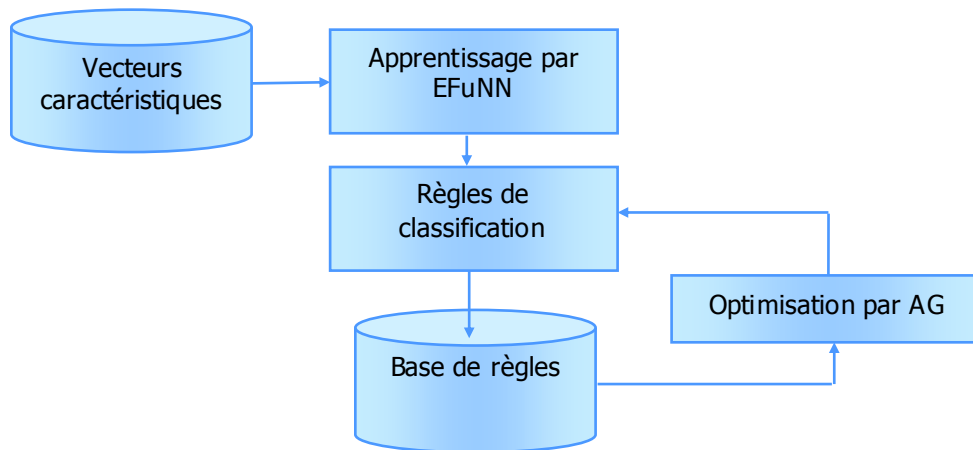
Figure 3.1 : Architecture du système proposé
