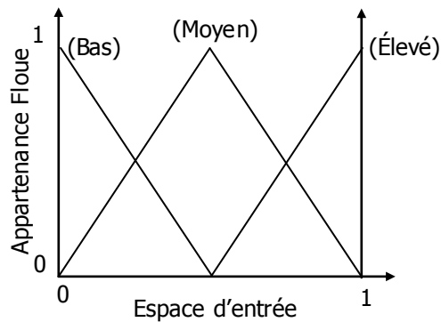
Figure 3.2 : Ensemble des trois fonctions d'appartenance floue ainsi que leur correspondance linguistique.
