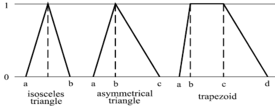
Figure 1.9 : Différentes fonctions d'appartenance avec des points caractéristiques [RUT 08]
