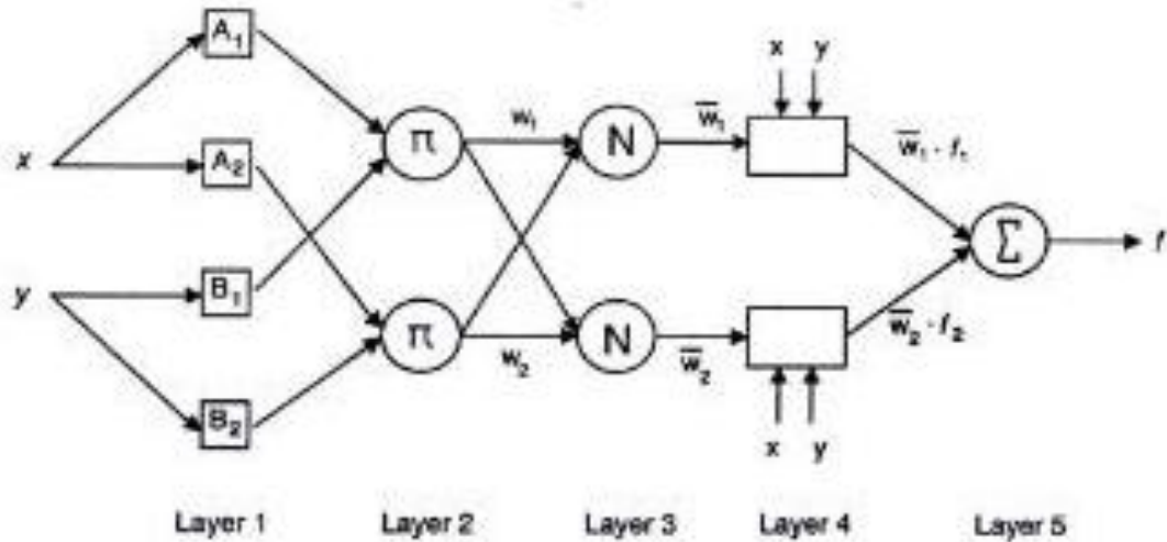
Figure 1.15 : Architecture ANFIS correspondant à un modèle Sugeno flou premier-ordre de deux-entrées avec deux règles
