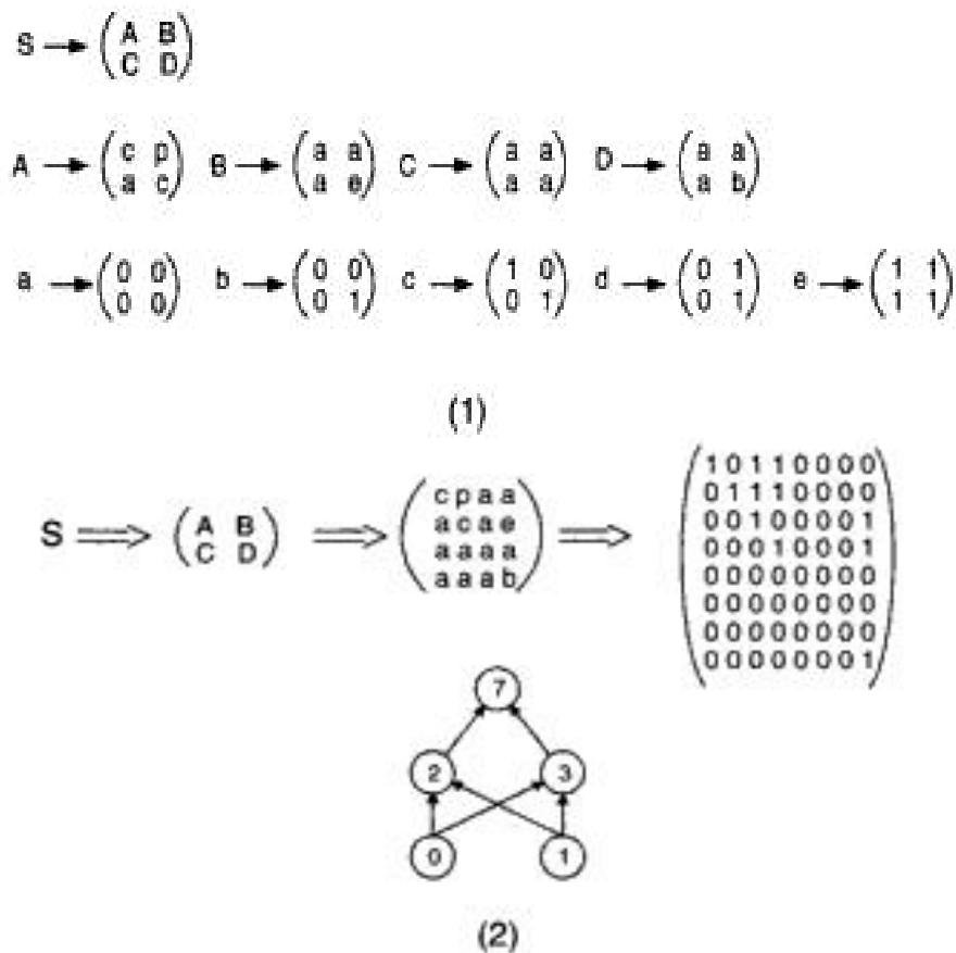
Figure 1. 11 : Exemple d'utilisation des règles de production de génération de graphe pour le développement d'un réseau feedforward ou-exclusif. La grammaire est représentée dans la partie (1). La partie (2) de la figure montre l'application consécutive des règles de la grammaire commençant par le symbole S et produisant un réseau pour le calcul de la fonction Booléenne ou-exclusif.
