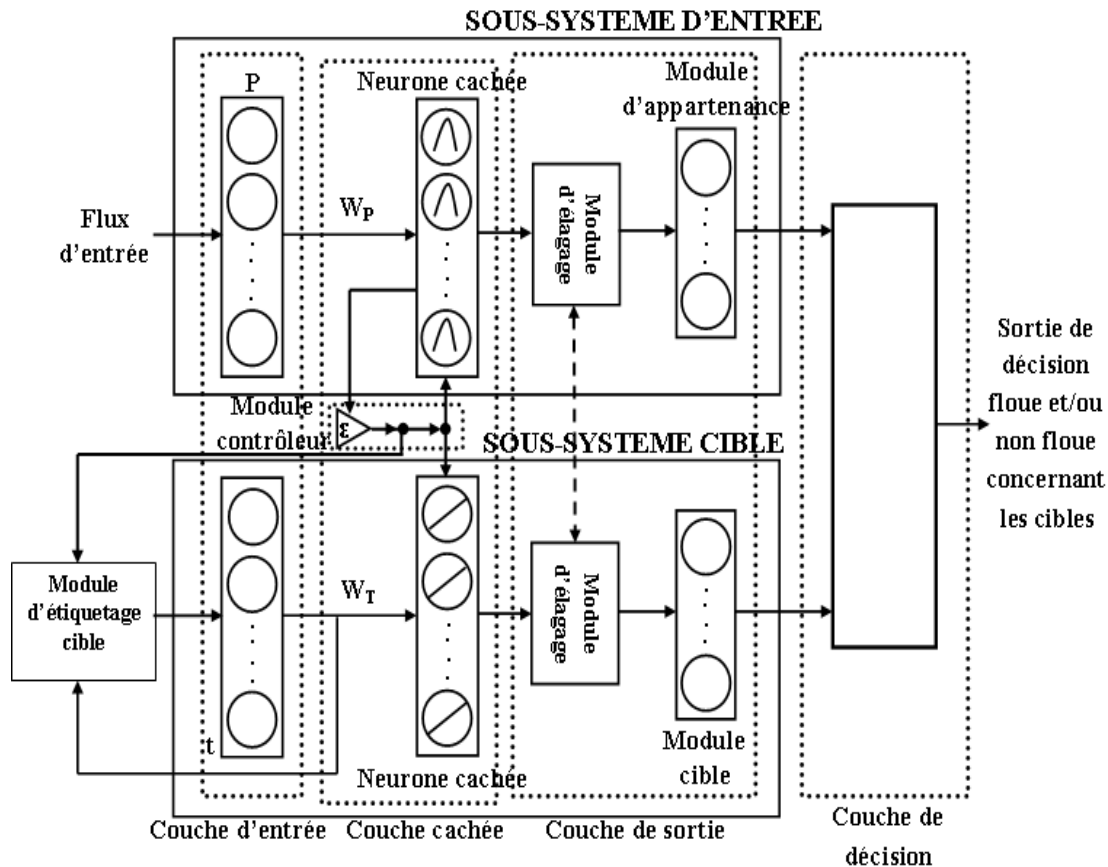
Figure 2.4 : Architecture de réseau du classifieur ILFN dans le mode d'exploitation [YEN 99]
