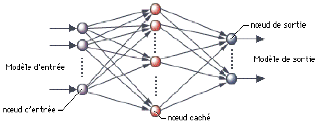
Figure 1.3 : Un réseau de neurones artificiel
