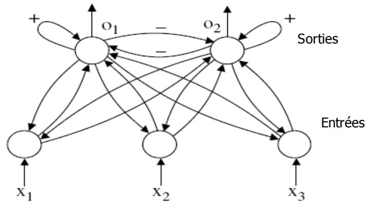
Figure 2.1 : Un diagramme schématique d'ART1 [KAS 07]
