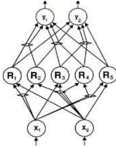
Figure 1.14 : Architecture schématique d'un système NEFPROX. Les connexions passant par les petits losanges sont liées c.-à-d., elles partagent le même poids
