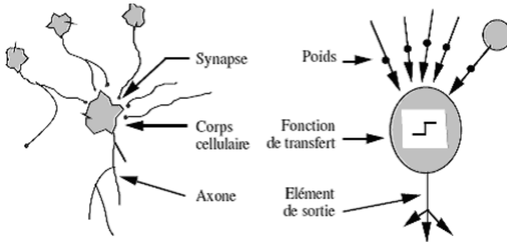
Figure 1.2 : Correspondance entre neurone biologique et neurone artificiel
