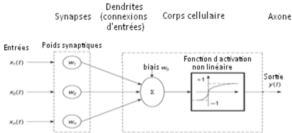
Figure 1.4 : Neurone Artificiel – Analogue électrique du neurone biologique [KAR 04]
