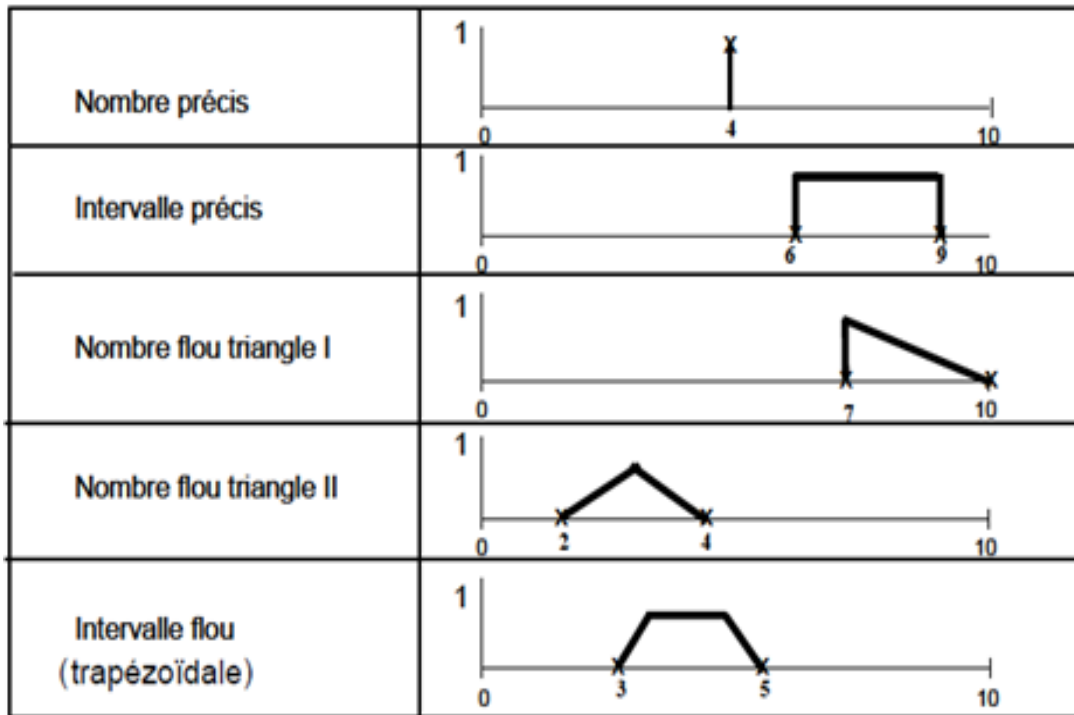
Figure 1.6 : Différentes distributions de possibilité
