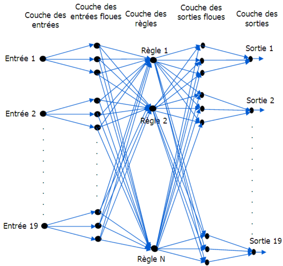
Figure 3.3 : Architecture du réseau de neurone flou évolutif EFuNN pour la classification d'images de la base « Image Segmentation » de l'UCI.
