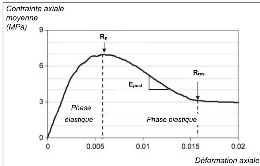
Figure II.18. Comportement typique d'un pilier de charbon d'après Jaiswal et Shrivastva (2009). Notons que la phase dite « élastique » ne l'est pas à proprement parler puisque la courbe y est non-linéaire à proximité du pic de résistance.
