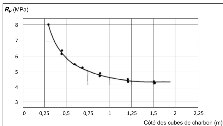
Figure II.21 Résistance des cubes de charbon testés par Bieniawski (1968) en fonction de leurs dimensions.
