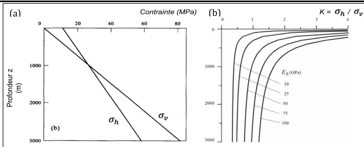
Figure II.3 : a) Répartition théorique des contraintes verticales et horizontales dans la partie supérieure de la croûte terrestre, et b) Répartition du coefficient K en fonction de la profondeur (Sheorey, 1994).
