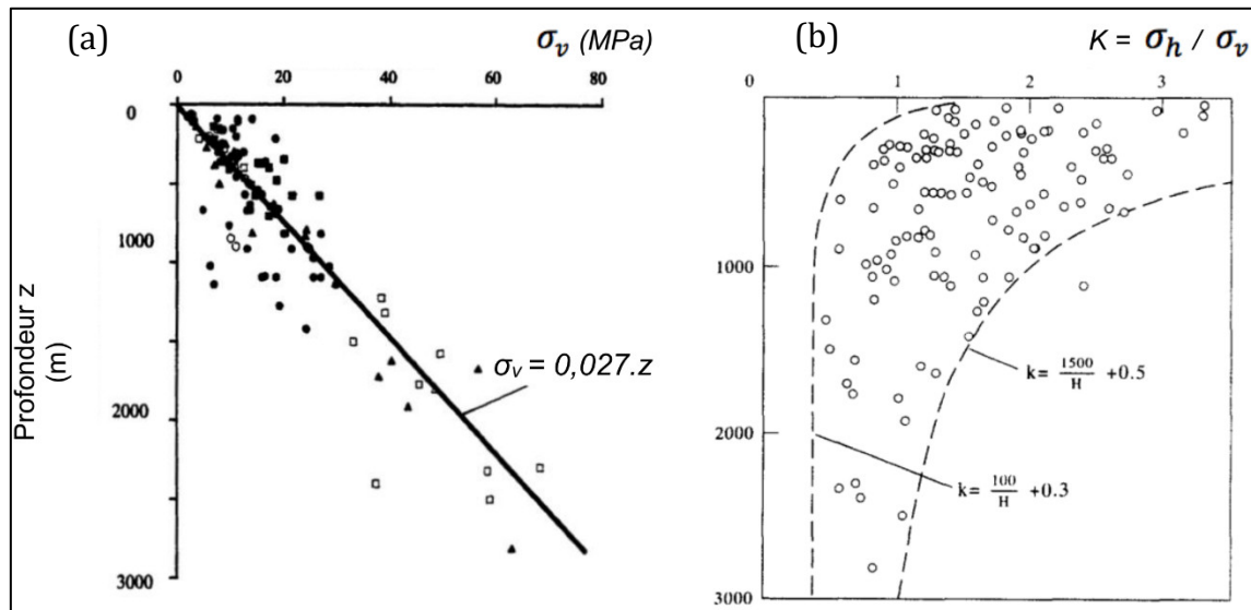
Figure II.2 : a) Mesures de contrainte verticale dans différentes régions du Monde et ajustement d'une relation linéaire avec la profondeur (Hoek et al., 2000); b) valeurs du coefficient K mesurées sur différents continents, en fonction de la profondeur (Hoek et Brown, 1980).
