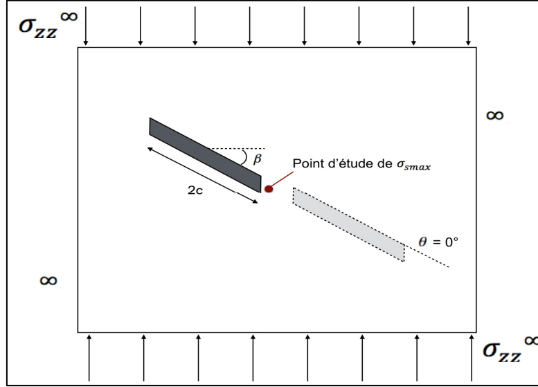
Figure II.8 : Schéma du système considéré représentant une galerie inclinée par rapport à la contrainte verticale in situ \sigma_{zz}^\infty .
