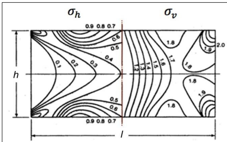
Figure II.5 : Isovaleurs des contraintes horizontales et verticales à l'intérieur d'un pilier de rapport de forme l/h = 2 soumis à un état de contrainte lithostatique (d'après Jeremic, 1985).
