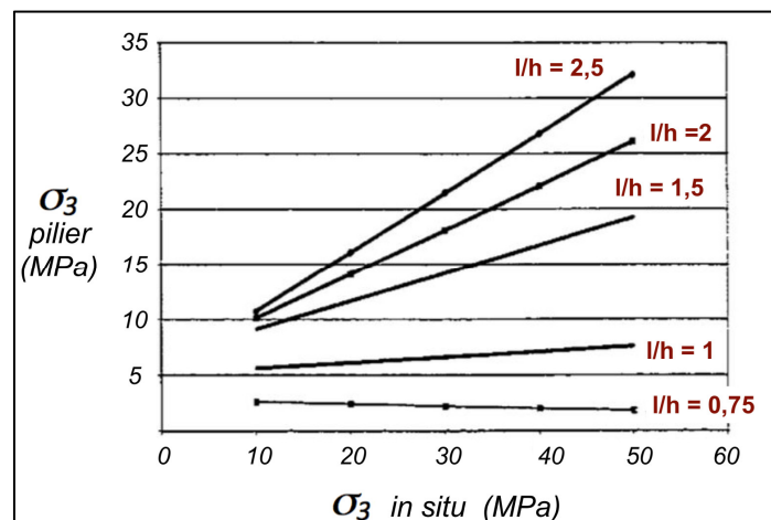
Figure II.10 : Résultats numériques de calculs de contrainte de confinement à l'intérieur de piliers de différents rapports l/h et pour différentes valeurs in situ de \sigma_3 (modifié et traduit de l'anglais au français d'après Maybee, 2000).
