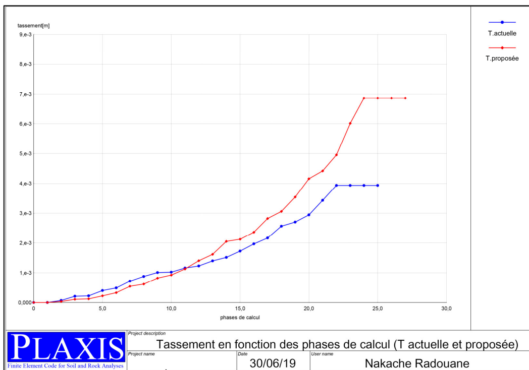
Figure IV.13. Tassements à l'entrée du massif en fonction des phases de calcul (technique actuelle et proposée).
