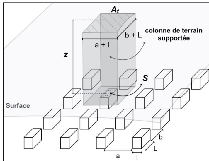
Figure II.12 : Schéma de principe de la théorie de l'aire tributaire tiré de Hauquin et al. (2016).
