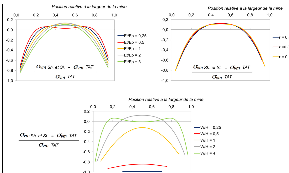
Figure II.14 : Comparaison des contraintes verticales moyennes obtenues avec la méthode de Sheorey (Eqs II.17 à II.21), en considérant des conditions d'appuis de type rotule, à celles obtenues par la méthode de l'aire tributaire (Eqs II.14 à II.16) pour différentes configurations géométriques et mécaniques (Thomas .H. 2016).
