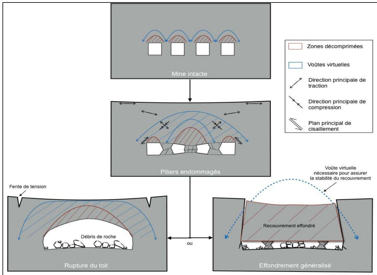
Figure I.14 : Schéma conceptuel du fonctionnement mécanique d'un ensemble de piliers en interaction avec leur recouvrement à différents niveaux d'endommagement. Inspiré de « l'effet domino » tel que décrit par Ma et al. (2012).
