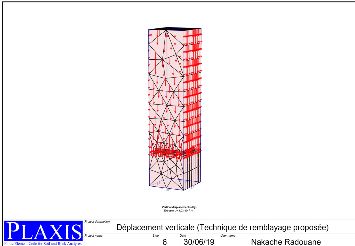
Figure IV.17. Déplacements verticaux de la technique de remblayage
