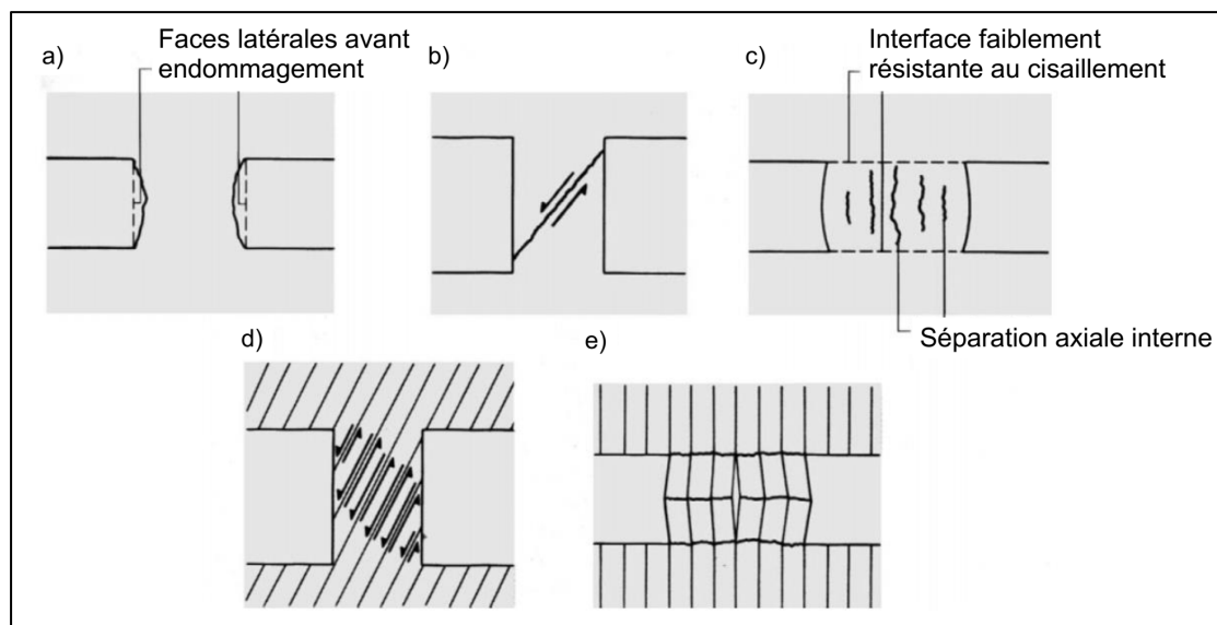
Figure I.7 : Modes de rupture des piliers de mine en fonction des conditions géomécaniques dans lesquelles ils se trouvent (traduit de l'anglais au français, d'après Brady et Brown, 2004).
