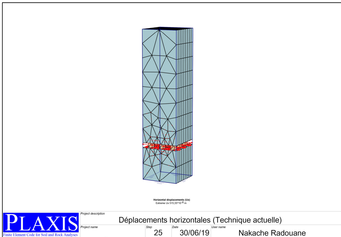
Figure IV.11 Déplacements verticaux et horizontaux de la technique actuelle
