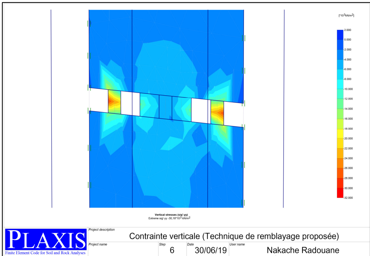
Figure IV.15. Distribution des contraintes verticales après remblayage
