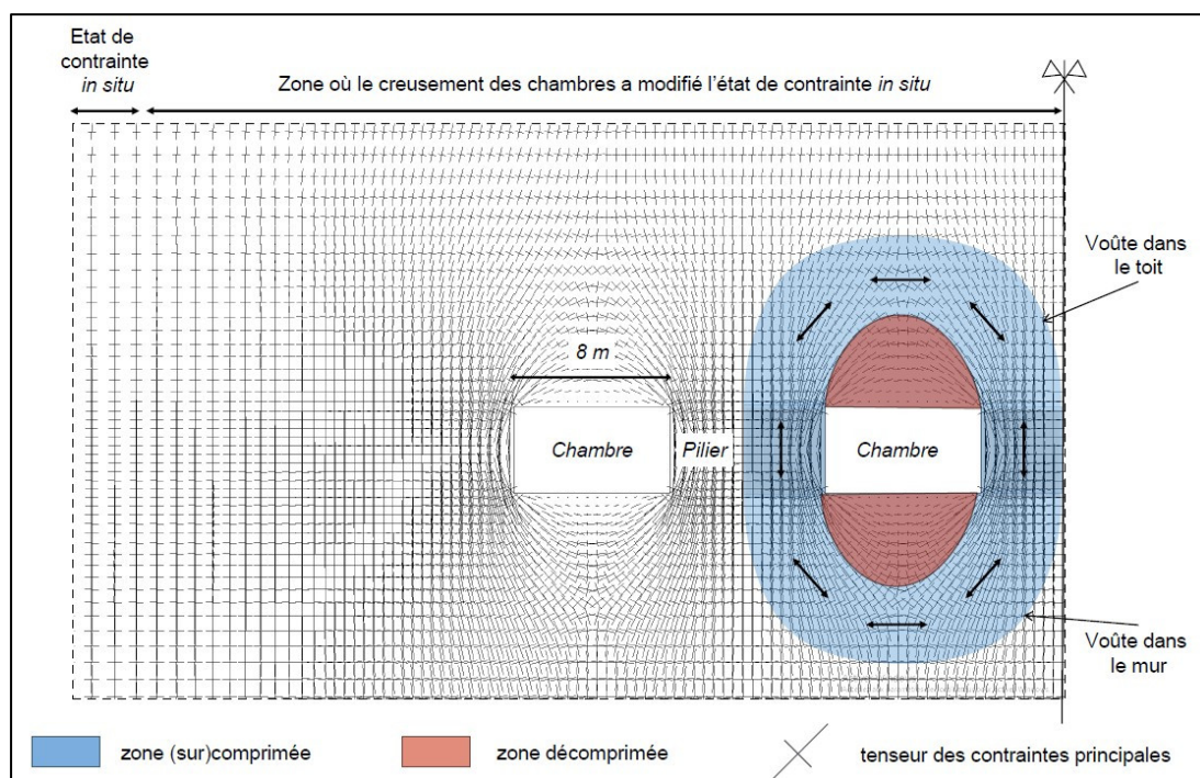
Figure I.6 : Modification de l'état de contrainte induite par le creusement de chambres d'après des résultats de modélisation numérique 2D en milieu continu (FLAC) (Thomas 2016).
