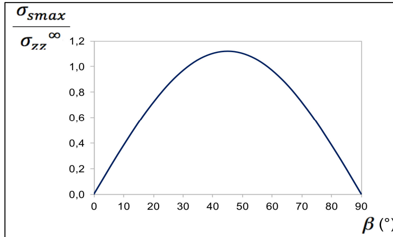
Figure II.9 : Effet de l'inclinaison d'une galerie par rapport aux contraintes principales in situ sur la contrainte de cisaillement maximale aux bords de la galerie.
