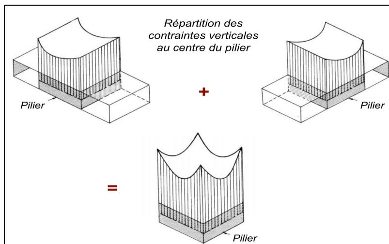
Figure II.6 : Représentation de la contrainte verticale au centre d'un pilier de section carrée (3D) par superposition des contraintes verticales dans deux piliers infiniment allongés (2D) et orientés perpendiculairement l'un par rapport à l'autre.
