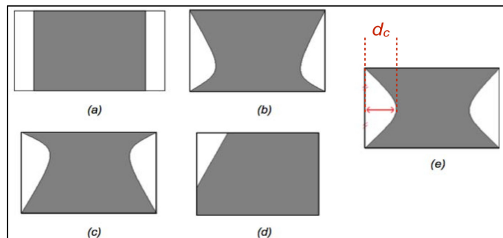
Figure II.22. Illustration des cinq types d'écaillage des piliers observés par Van der Merwe (2003b) dans les mines de charbon sud-africaines.
