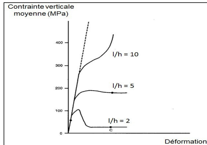
Figure II.20 : Illustration du comportement des piliers typiques des mines de « roche dure » sud-africaines en fonction de leur rapport de forme l/h , d'après Ozbay et al. (1995).
