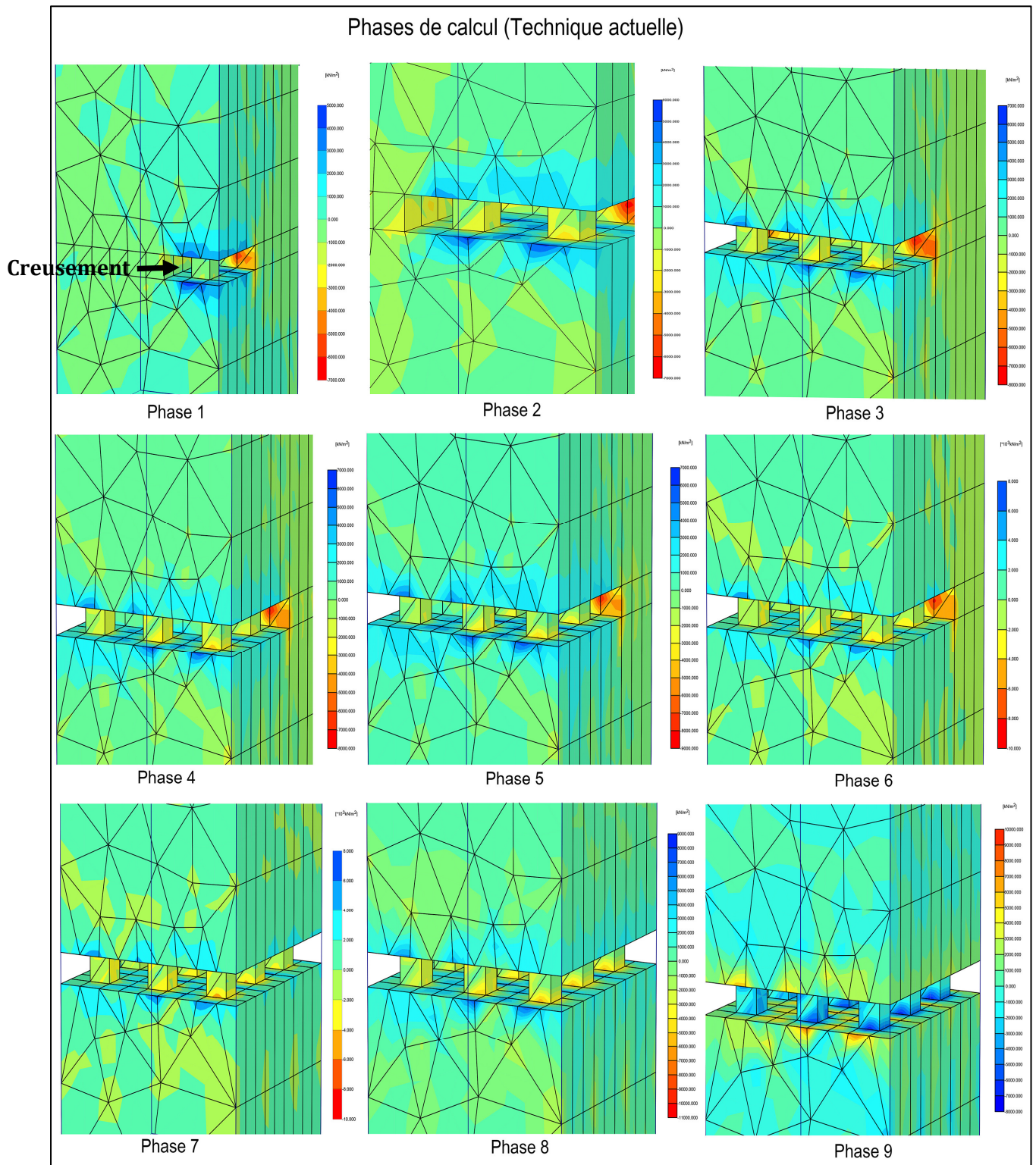
Figure IV.5 Phases de calcul (Technique actuelle)
