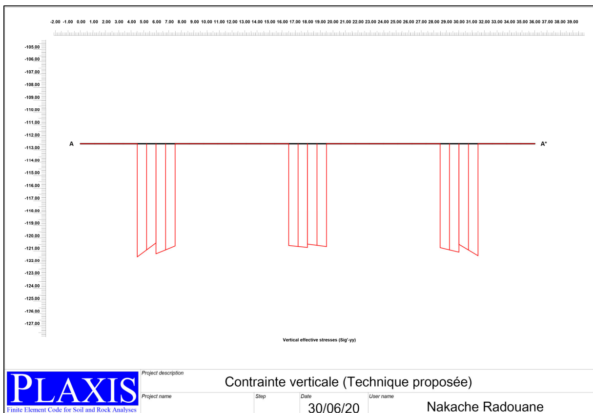
Figure IV.10. Concentration de contrainte verticale à l'intérieur du piler coupe A-A' (technique proposée)
