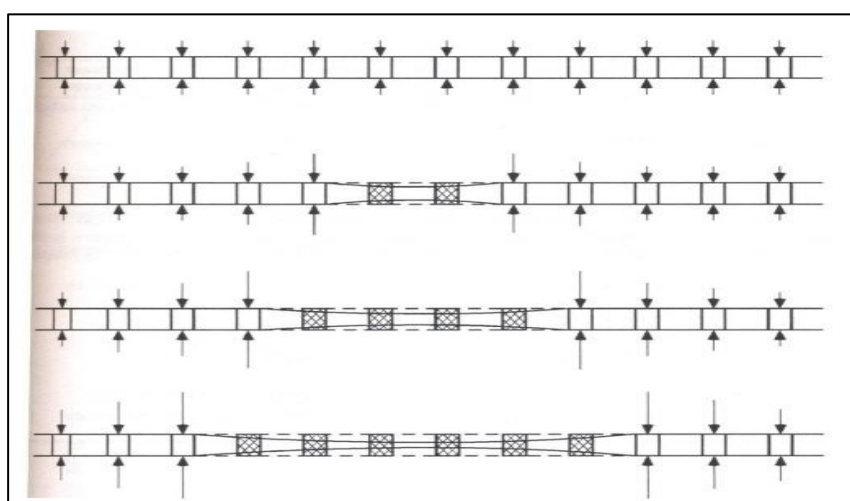
Figure I.13 : Mécanisme de rupture en cascade de piliers tels que représenté par Zipf (2001). Les flèches verticales symbolisent l'intensité de la contrainte verticale agissant sur les piliers sains à mesure que le nombre de piliers endommagés augmente.
