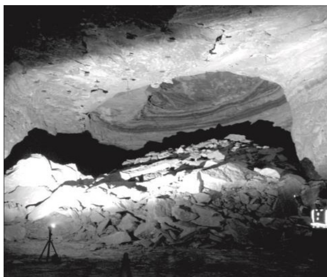
Figure I.10 : Cloche d'effondrement du toit d'une chambre photographiée par Esterhuizen et al. (2011) dans des carrières de calcaire américaines.
