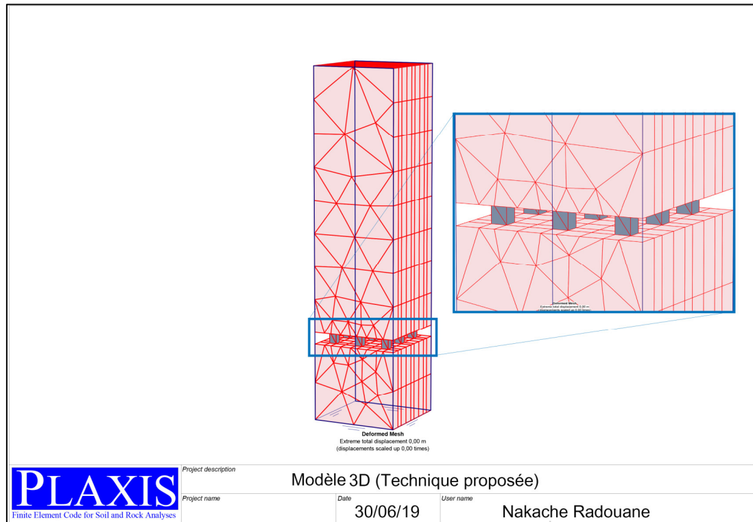
Figure IV.4. Modèle 3D pour les deux techniques (a) T actuelle et b) T proposée)
