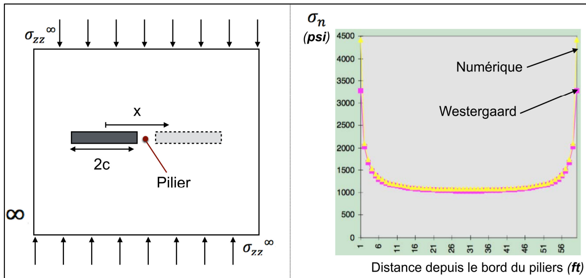
Figure II.7 : Comparaison de la solution de Westergaard appliquée à un pilier, à des résultats de modélisation numérique en milieu élastique homogène isotrope (Hoch et al., 1991).
