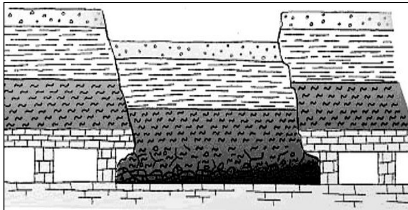
Figure I.12 : Schéma conceptuel d'un effondrement brutal
