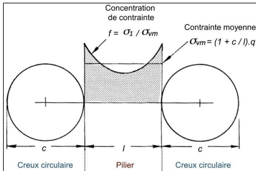
Figure II.4 : Répartition des contraintes verticales élastiques entre deux creux circulaires (d'après Hoek et Brown, 1980, sur la base des résultats d'Obert et Duvall, 1967).
