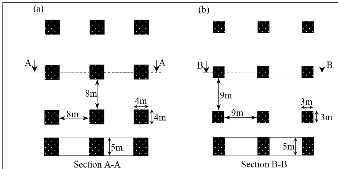
Figure IV.3 Méthode de chambres et piliers, (a-technique actuelle, b-technique proposée)
