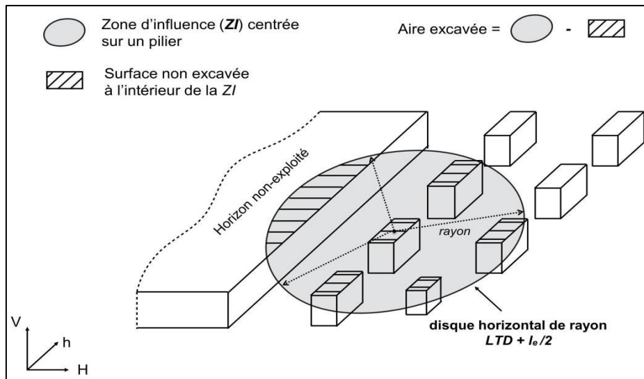
Figure II.15 : Schéma de principe de la théorie de la « voûte de contrainte » (PAT, Poulsen, 2010) tiré de Hauquin et al. (2016).
