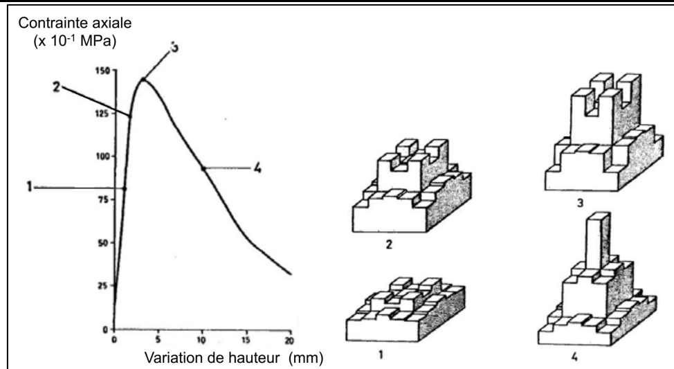
Figure II.16 : Résultat d'un essai de compression sur un pilier de charbon de 2 m de largeur par 1 m de hauteur et répartition de la contrainte axiale durant le chargement, d'après Wagner (1980).
