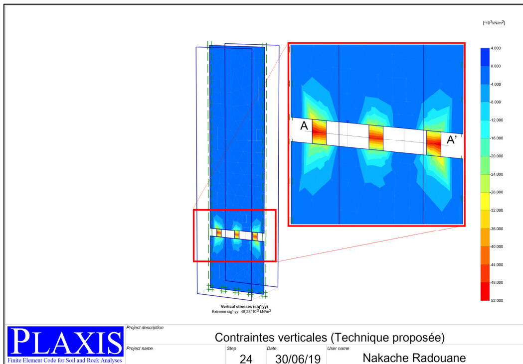
Figure IV.9. Distribution des contraintes verticales après dépilage et l'illustration des contours de l'air tributaire locale des piliers adjacents (technique proposée)
