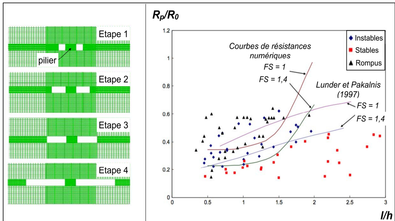
Figure II.24 : Vue sur les différentes phases des modèles 2D réalisés par Mortazavi et al. (2009) pour modéliser la rupture d'un pilier (gauche). Graphique de stabilité (droite) superposant l'équation de résistance obtenue à partir des résultats de modélisation à la base de données de piliers de roche dure utilisée par Lunder et Pakalnis (1997).
