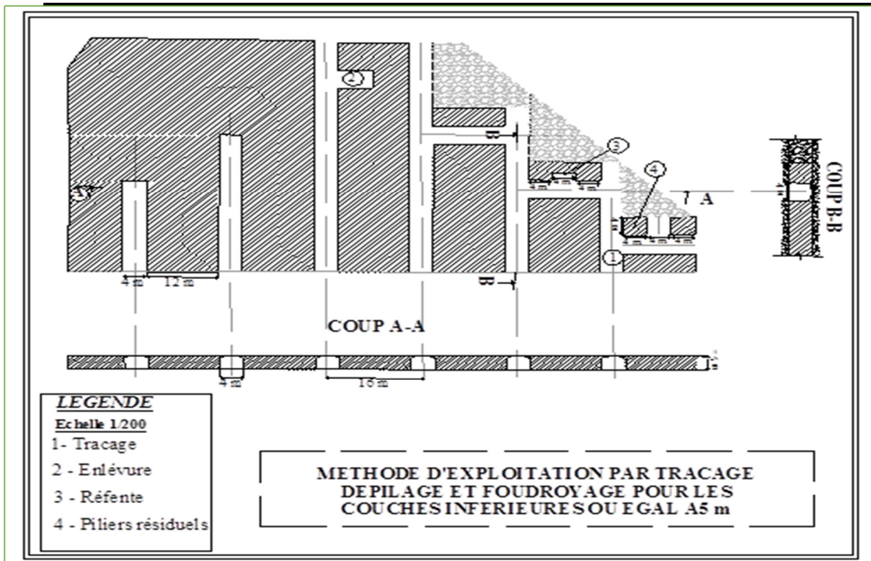
Figure III.8 Méthode de traçage et dépilage
