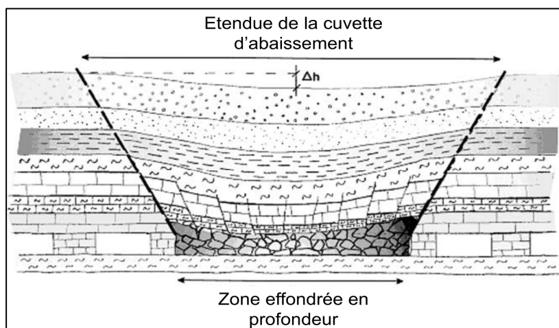
Figure I.11 : Schéma conceptuel d'un affaissement continu progressif
