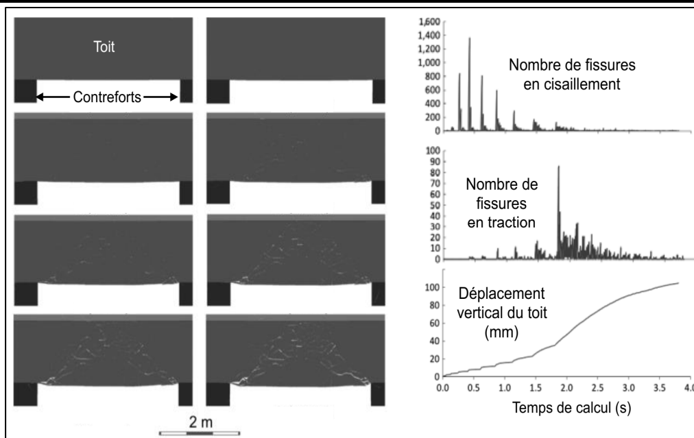
Figure I.9 : Rupture progressive du toit au-dessus d'une galerie étroite (5 m) obtenue numériquement par Gao et al. (2014).
