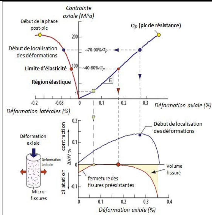
Figure II.1 : Résultats typiques d'un essai de compression simple sur un échantillon de granite, d'après Martin et Chandler (1994).
