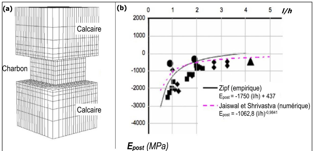
Figure II.25. a) Maillage d'un des modèles 3D de pilier réalisés par Jaiswal et Shrivastva (2009) pour modéliser des essais de compression.
