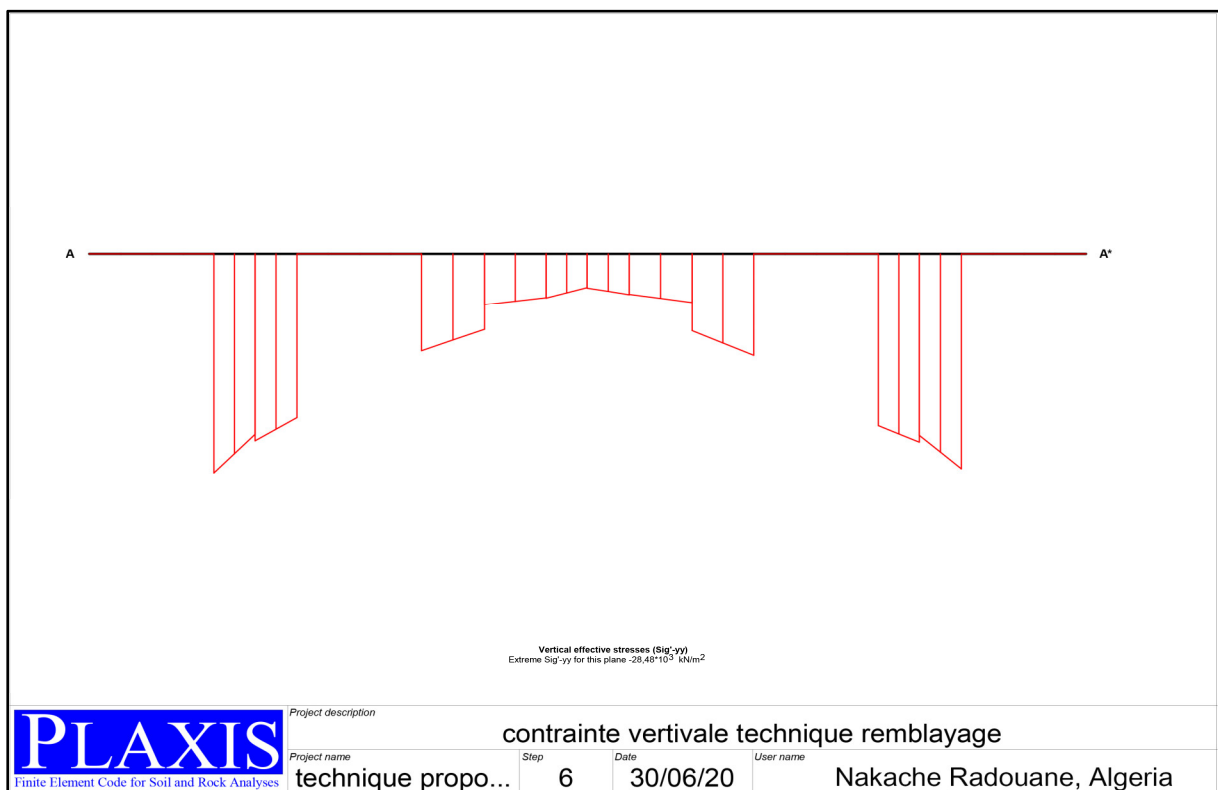
Figure IV.16. Concentration de contrainte verticale à l'intérieur de la zone du remblai coupe A-A'
