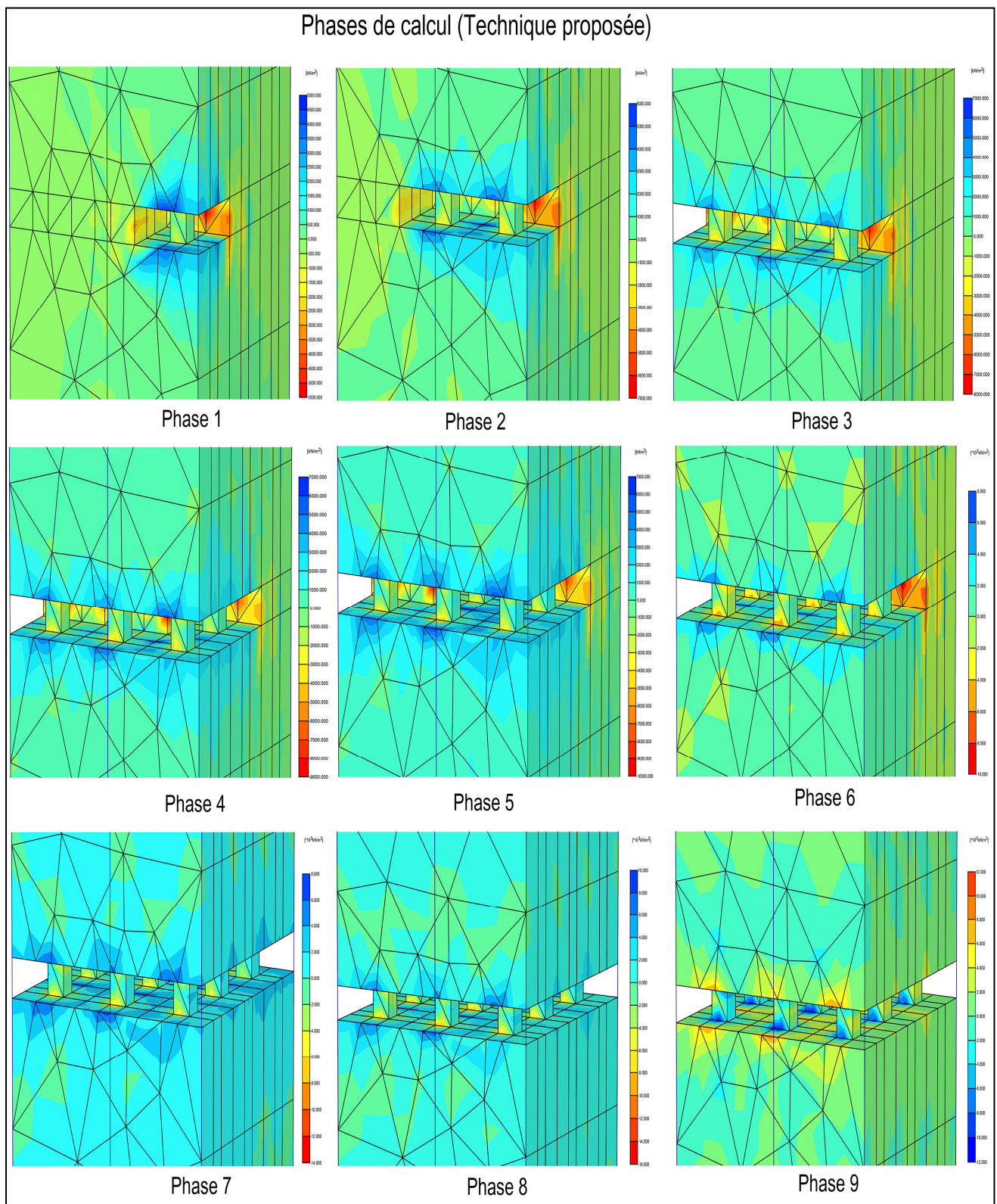
Figure IV.6. Phases de calcul (Technique proposée)
