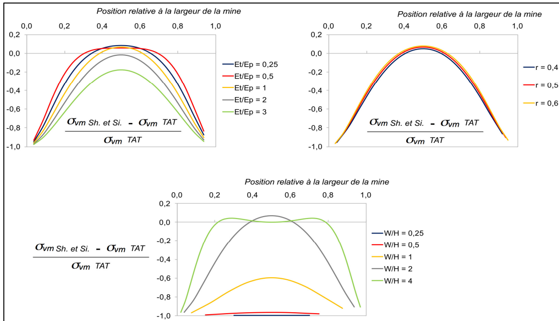
Figure II.13 : Comparaison des contraintes verticales moyennes obtenues avec la méthode de Sheorey (Eqs II.17 à II.21), en considérant des conditions d'appuis encastrés, à celles obtenues par la méthode de l'aire tributaire (Eqs II.14 à II.16) pour différentes configurations géométriques et mécaniques (Thomas .H. 2016).
