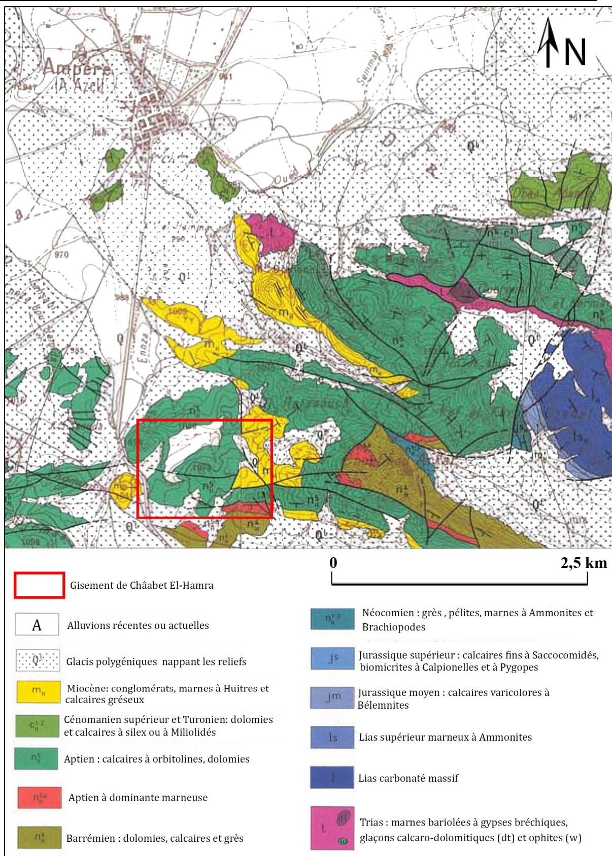
Figure III.1. Carte géologique des environs de la mine de Châabet El-Hamra (D'après Carte géologique au 1/50.000 d'Ain Azel, Sonatrach, 1977)
