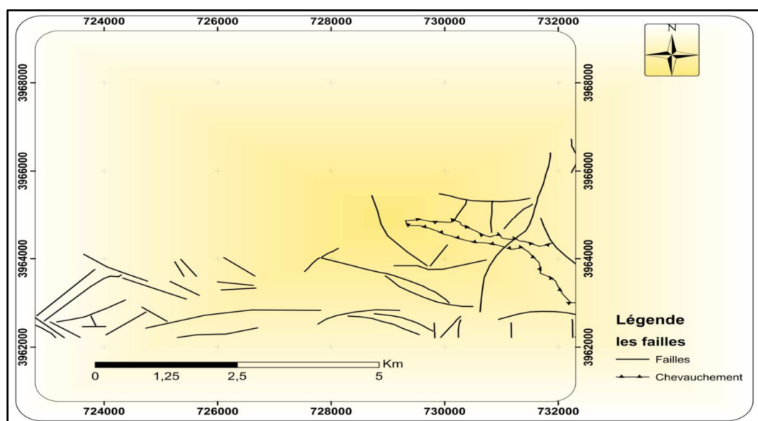
Figure III.4 Carte linéaments du secteur d'étude
