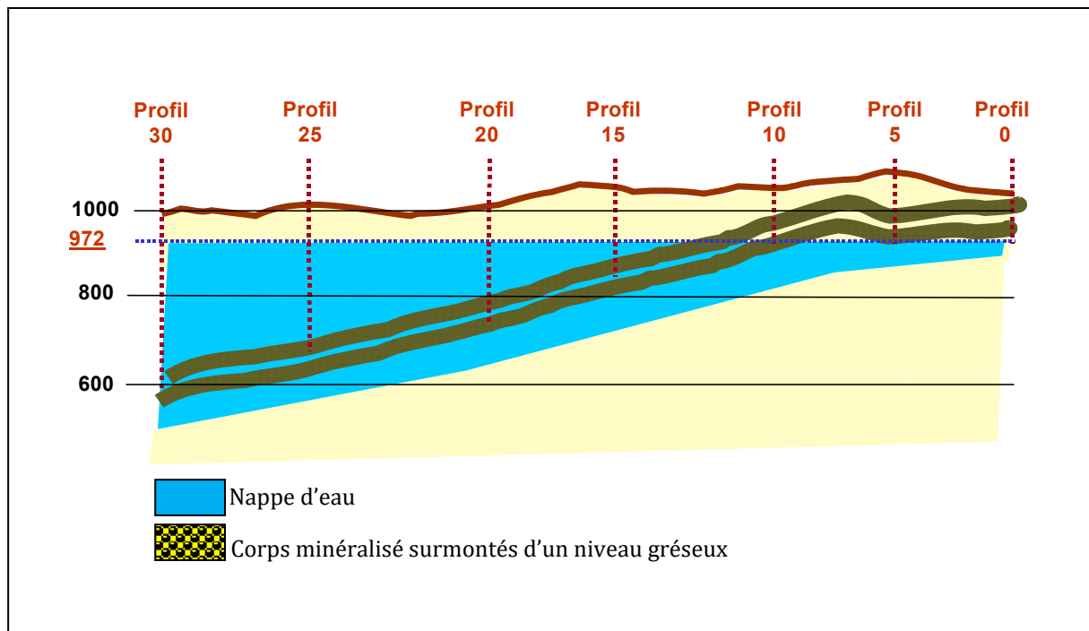
Figure III.6. Coupe hydrogéologique Profil 0 – Profil 30 (D'après ENOF 2003)
