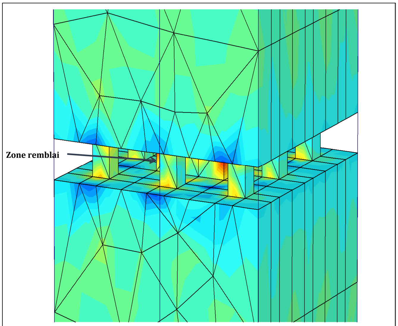
Figure IV.14. Phase de calcul de la Technique de remblayage
