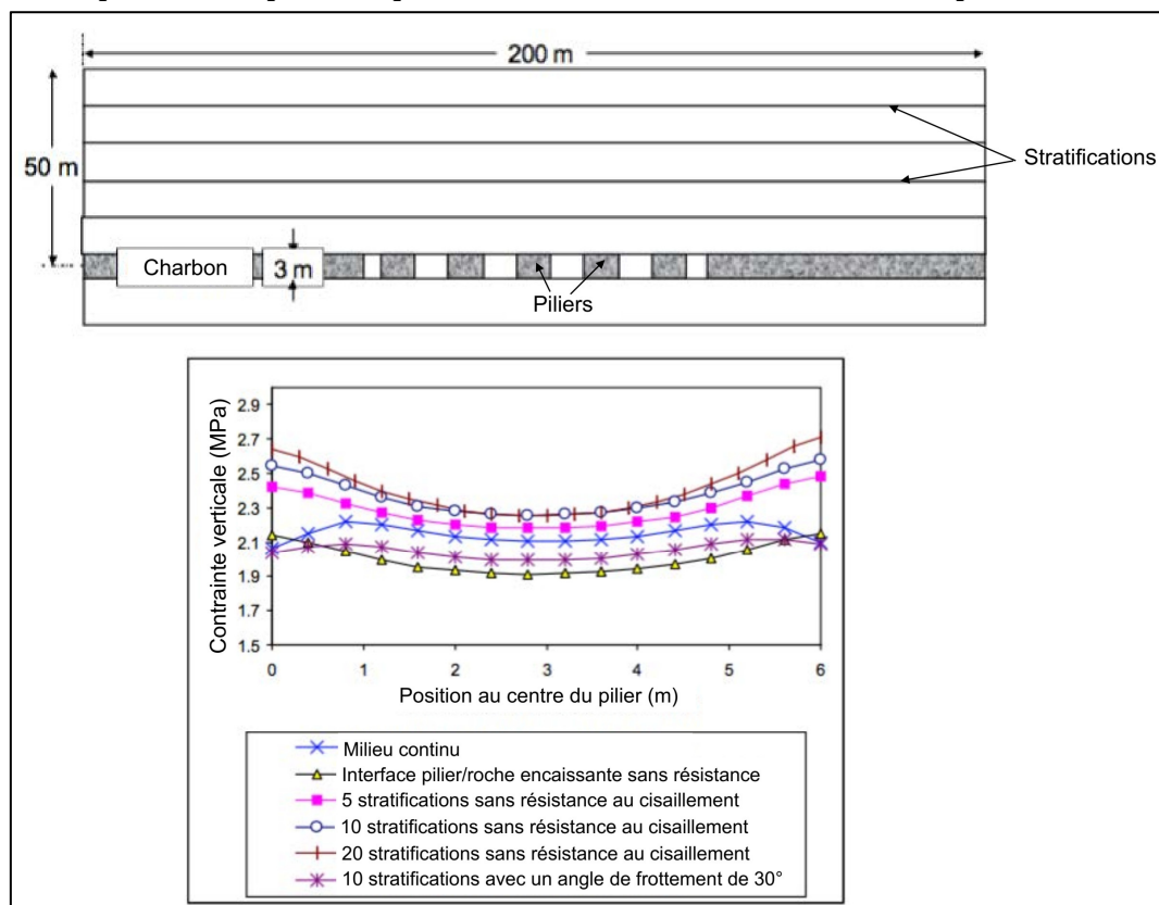
Figure II.11 : Effet de la présence des discontinuités dans le recouvrement sur la contrainte verticale au centre d'un pilier infiniment long de 6 m de largeur par 3 m de hauteur, situé à 50 m de profondeur avec un taux de défrutement de 0,5, d'après Roberts et al. (2002).
