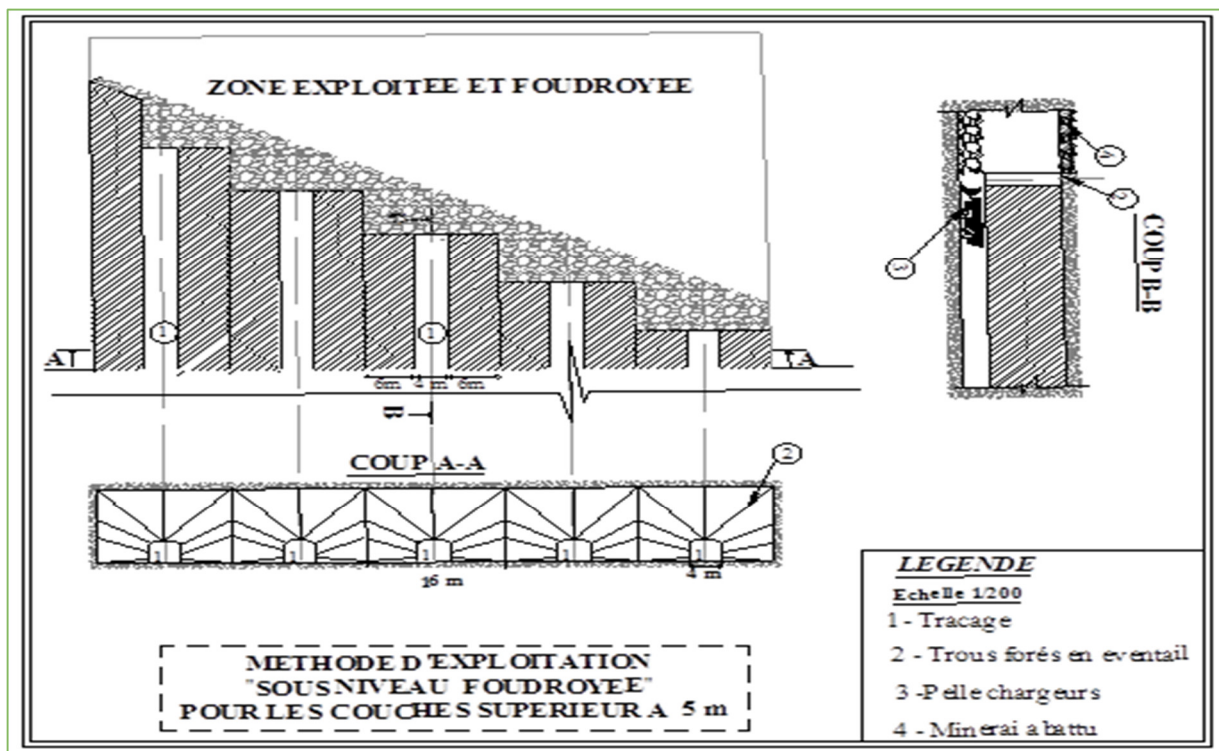
Figure III.9 Méthode des sous-niveaux foudroyés
