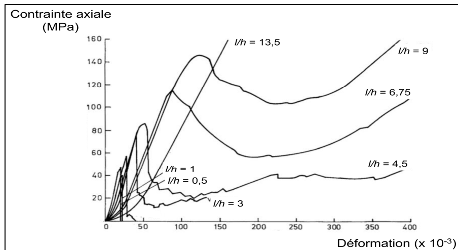
Figure II.19 : Résultats d'essais de compression réalisés par Das (1986) sur des échantillons de marbre de 5,4 cm de diamètre l et de différents rapports de forme l/h .
