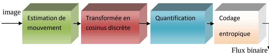
Figure I.11 Schéma du codage INTER
