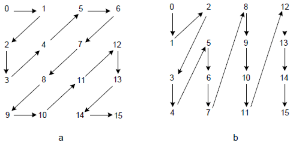
Figure II.7 Ordre de balayage des coefficients (a) en mode frame (b) en mode champ (field)
