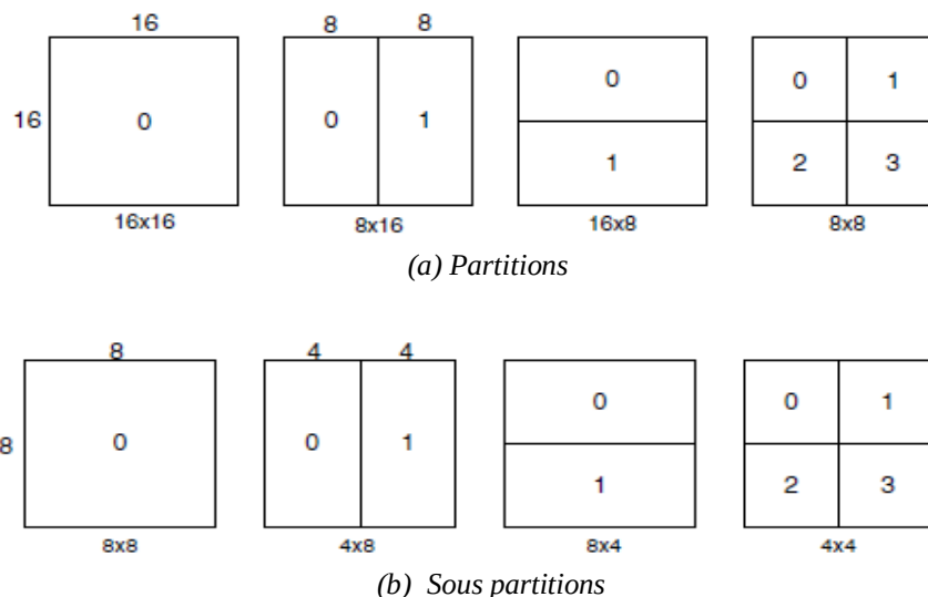
Figure II.10 Exemple de partition avec blocs à taille variable.
