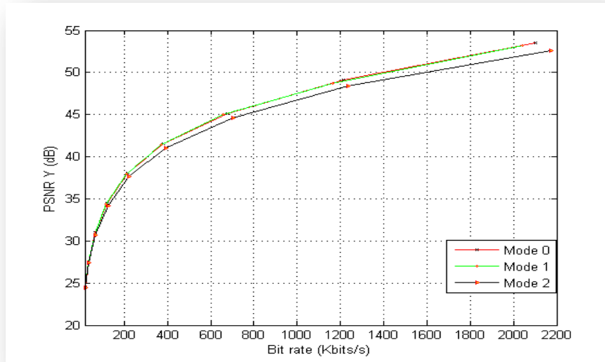
Figure IV.15.a Courbe débit-distorsion
