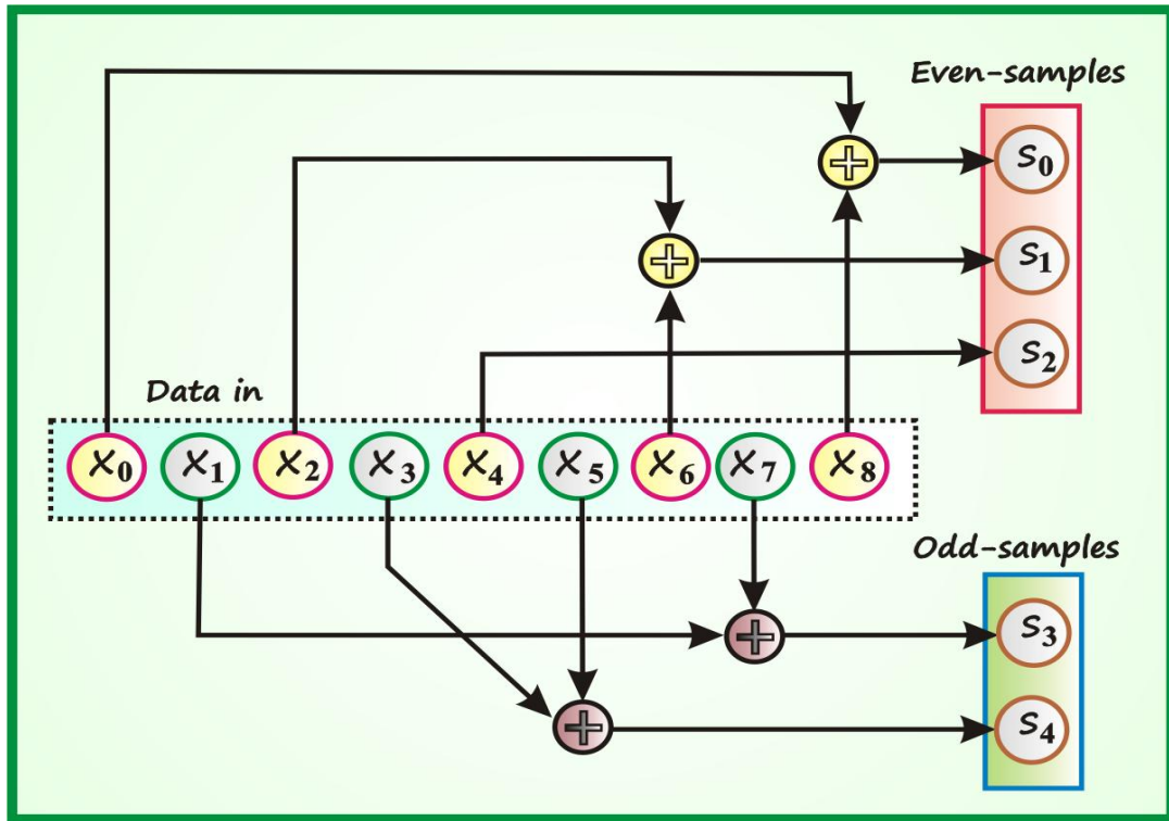
Figure V.7 Génération des adresses paires et impaires. (cas du filtre passe bas à 9 coefficients)
