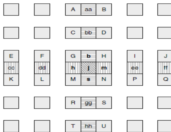
Figure II.13 Interpolation des échantillons demi-pixel
