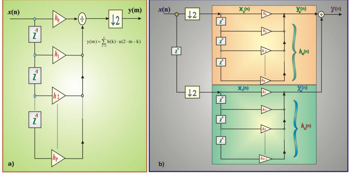
Figure V.4 (a) structure transversale suivie d'un décimateur , (b) structure polyphase.
