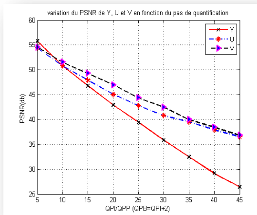
Figure IV.5(a) PSNR de Y, U et V en fonction de QP.
