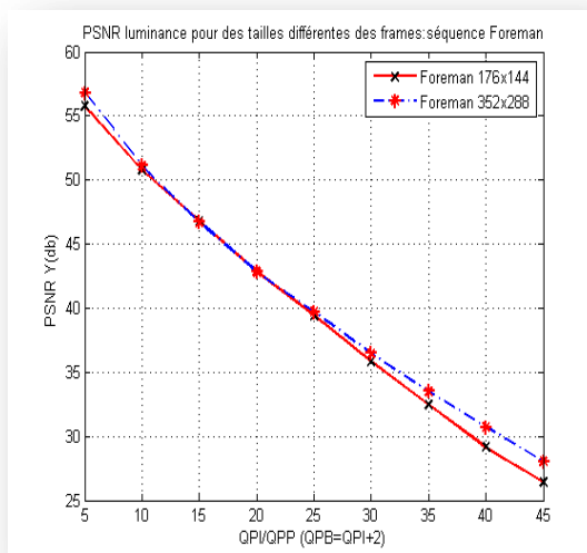
Figure IV.13(a) Influence du format sur le PSNR
