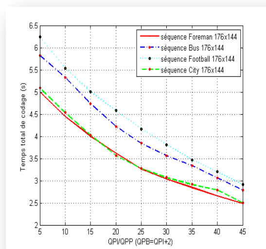
Figure IV.14(c) Temps de codage de différentes séquences vidéo
