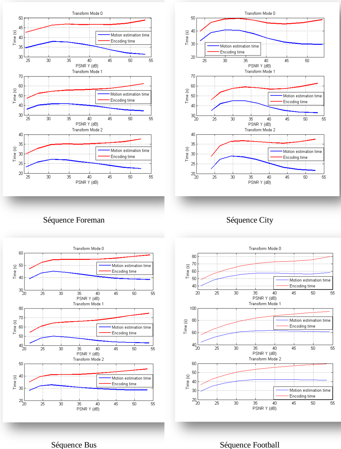
Figure IV.19 Variation du temps de codage et du temps d'estimation du mouvement en fonction de la séquence vidéo et du mode de transformation.
