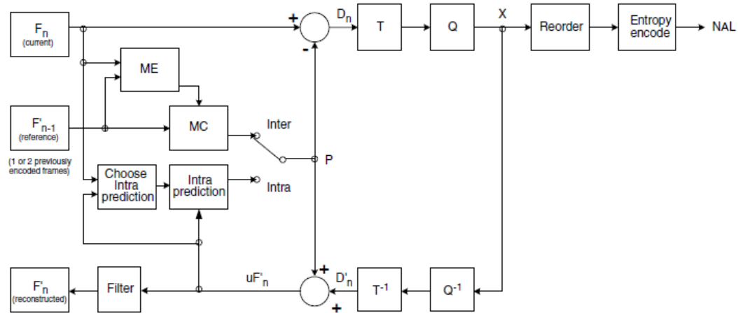
Figure II.1: Schéma fonctionnel d'un codeur vidéo H.264 [47]
