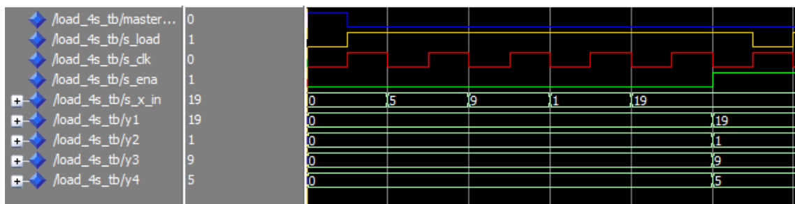
Figure V.20.b Simulation du circuit de chargement et conversion de 4 données.
