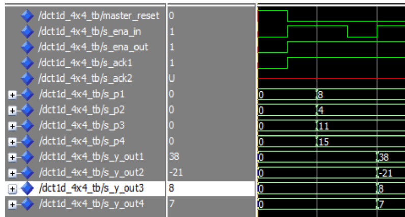
Figure V.21.b Résultat de la simulation du circuit DCT1D_4x4
