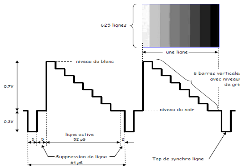
Figure I.5 Le signal vidéo monochrome
