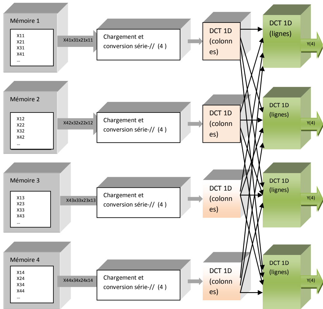
Figure V.16.b Schéma synoptique de la DCT entière 4x4 (version 2)
