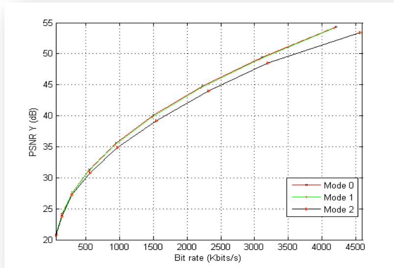
Figure IV.16.a Courbe débit-distorsion
