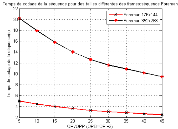
Figure IV.13(c) Influence du format sur le temps de codage.
