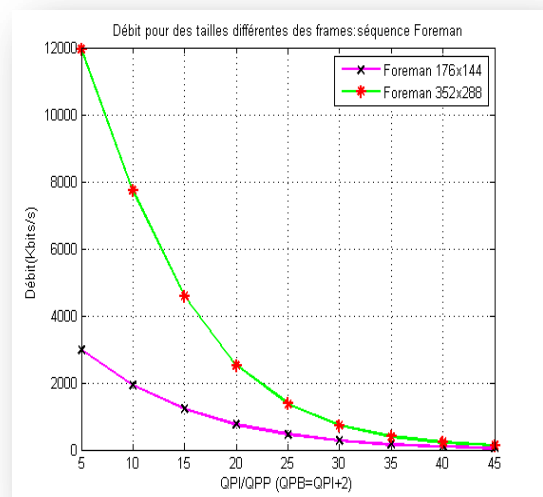
Figure IV.13(b) Influence du format sur le débit.
