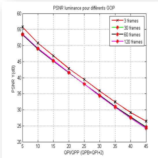
Figure IV.12(a) PSNR Y en fonction du pas de quantification pour différents GOP.
