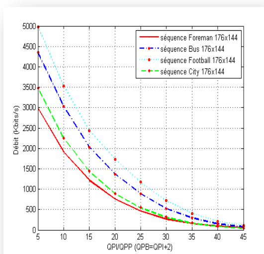
Figure IV.14(b) Débits de différentes séquences vidéo
