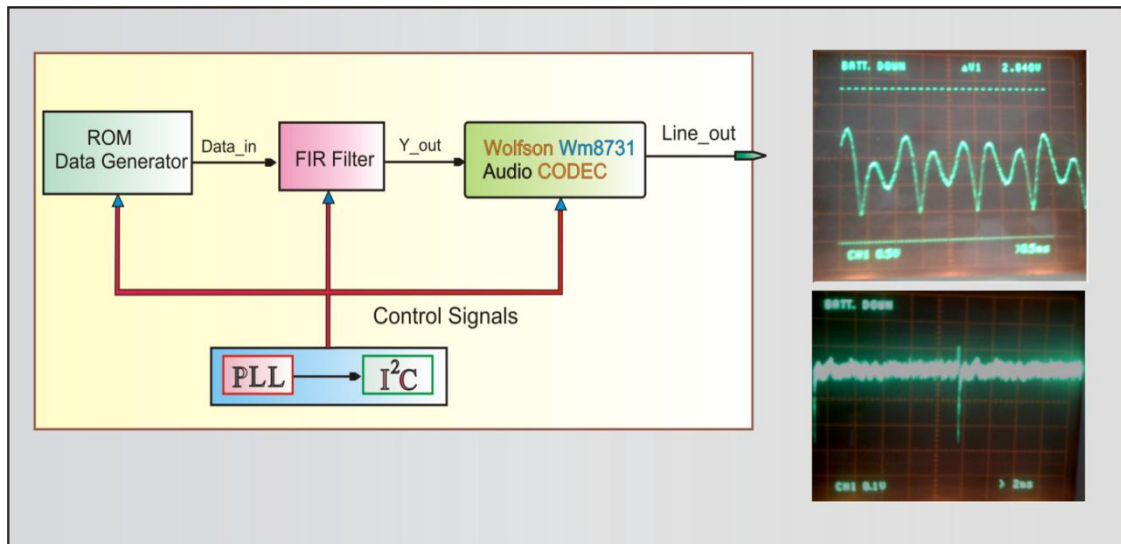
Figure V.14 Schéma synoptique de la configuration de test de l'implémentation hardware.
