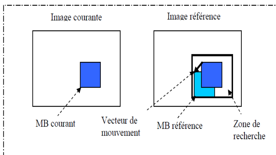
Figure II. 9 Principe de l'estimation de mouvement.
