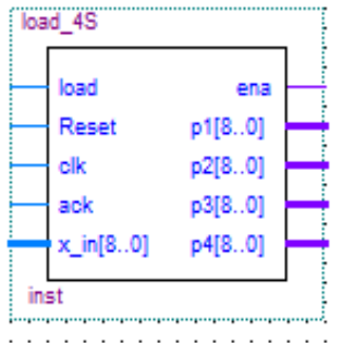
Figure V.19.b Symbole du circuit de chargement et conversion de 4 données.
