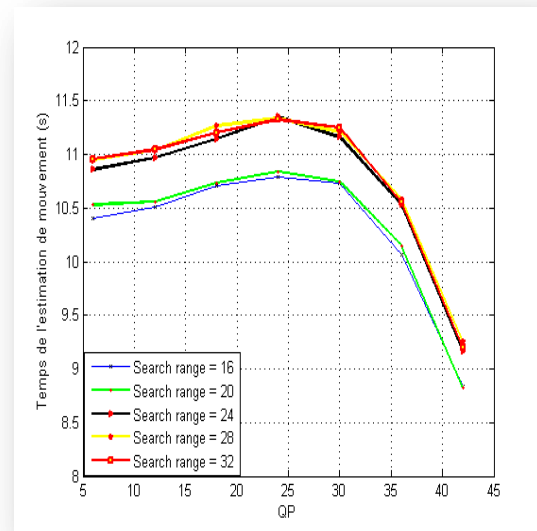
Figure IV.11(d) Temps d'estimation du mouvement pour différents search range (séquence Football)
