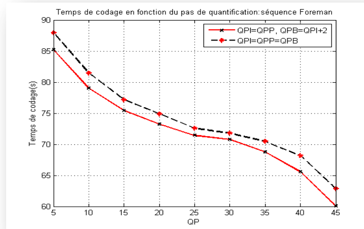
Figure IV.8(c) Temps de codage pour QPI=QPP=QPB et QPI=QPP \neq QPB (30 frames).
