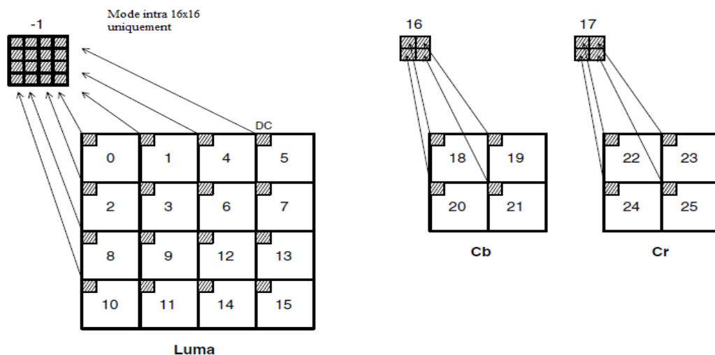
Figure III.4. Ordre de parcours des blocs résiduels d'un macrobloc.
