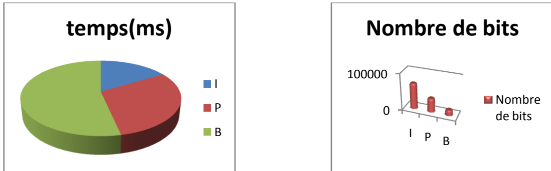
Figure IV.6(a) Temps de codage des frames I, P et B. Figure IV.6(b) Nombre de bits des frames I, P et B.
