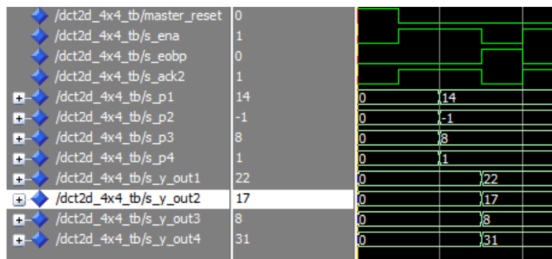
Figure V.22.b Résultat de la simulation du circuit DCT2D_4x4
