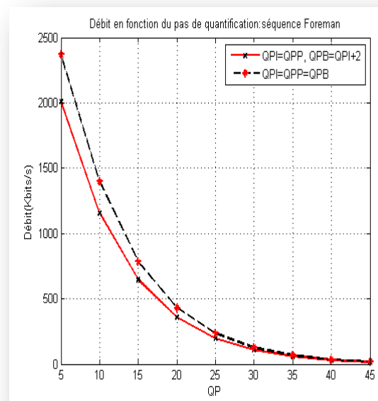
Figure IV.8(b) Débit pour QPI=QPP \neq QPB et QPI=QPP=QPB (cas de 30 frames)
