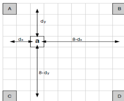
Figure II.15 Interpolation des positions huitième de pixel (composante de chrominance)
