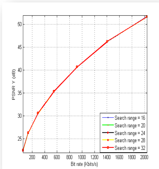
Figure IV.11(a) Courbes R-D pour différents search range (séquence Football)
