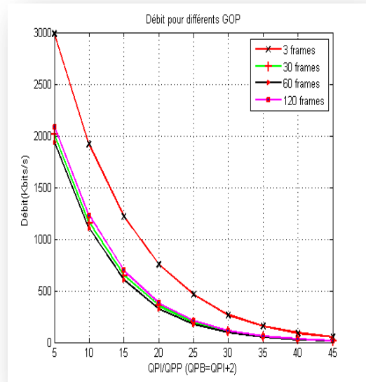
Figure IV.12(b) Débit en fonction du pas de quantification pour différents GOP.
