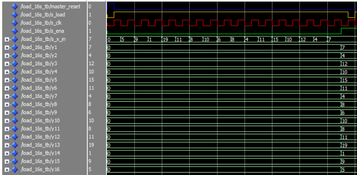
Figure V.20.a Simulation du circuit de chargement et conversion de 16 données.
