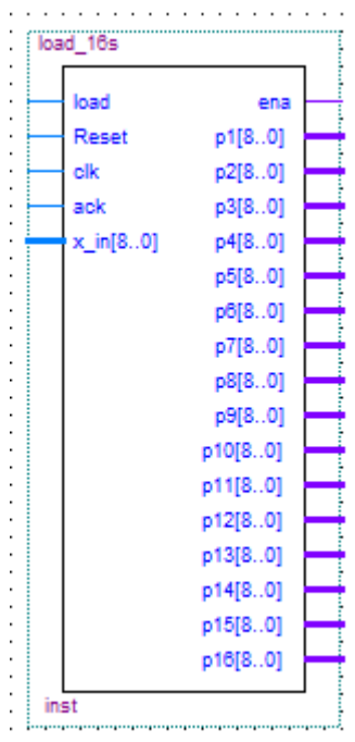
Figure V. 19.a Symbole du circuit de chargement et conversion de 16 données.
