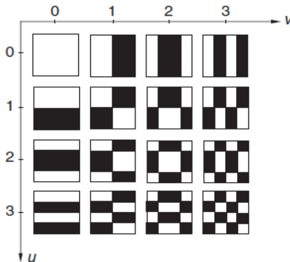
Figure III.1 Ensemble des 16 images de base de la DHT (N=4)
