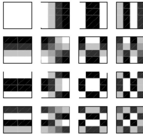
Figure III.2 Les images de base de la DCT 4x4.
