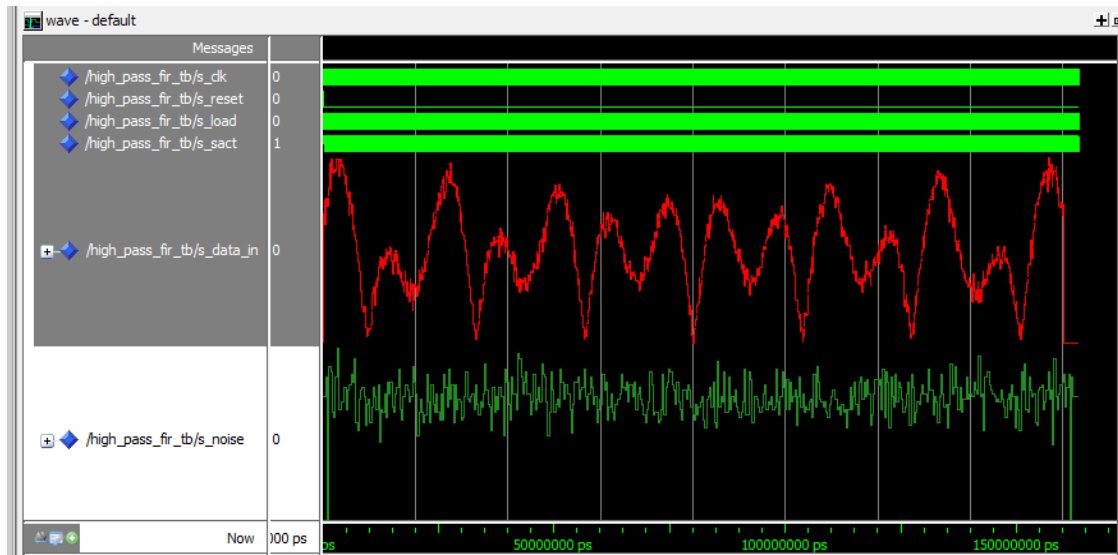
Figure V.13 Résultat de simulation avec Modelsim. Signal bruité (en haut), bruit ou détails (en bas).
