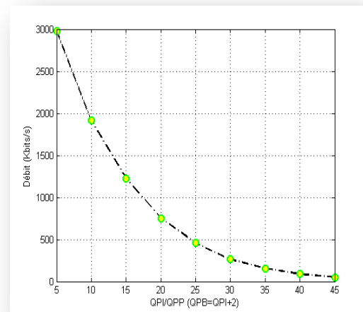
Figure IV.5 (b) Débit en fonction de QP.
