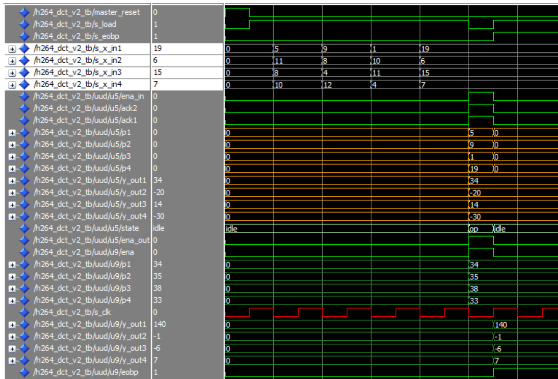
Figure V.23.a Résultat de la simulation de la DCT 2D entière 4x4 (pour 4 échantillons)
