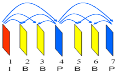
Figure I.12 Ensemble d'images (Groupe of Pictures)
