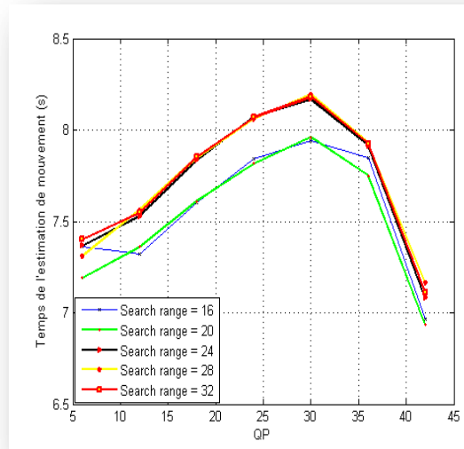
Figure IV.10(d) Temps d'estimation du mouvement pour différents search range (séquence Foreman)
