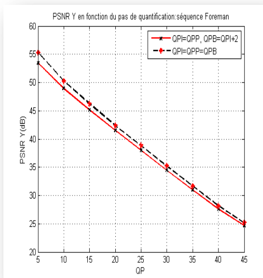
Figure IV.8(a) PSNR Y pour QPI=QPP \neq QPB et QPI=QPP=QPB (cas de 30 frames)
