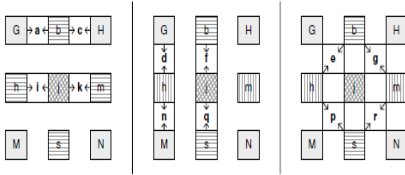
Figure II.14 Interpolation des échantillons quart de pixel.
