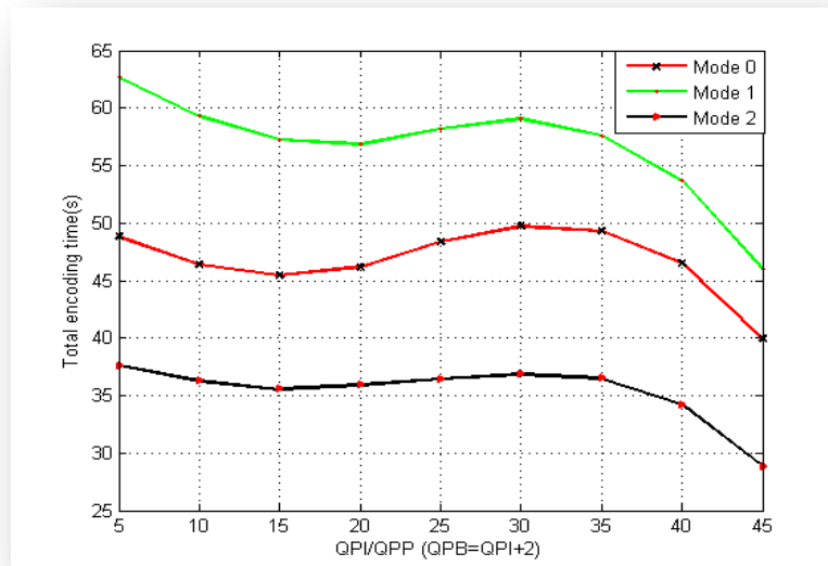
Figure IV.17.b Temps de codage
