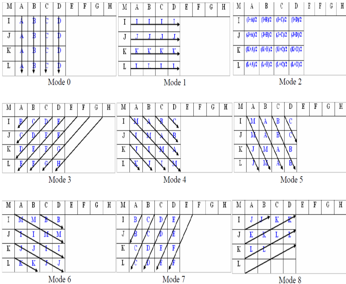
Figure II.5 : Prédiction d'un bloc 4x4 en mode intra
