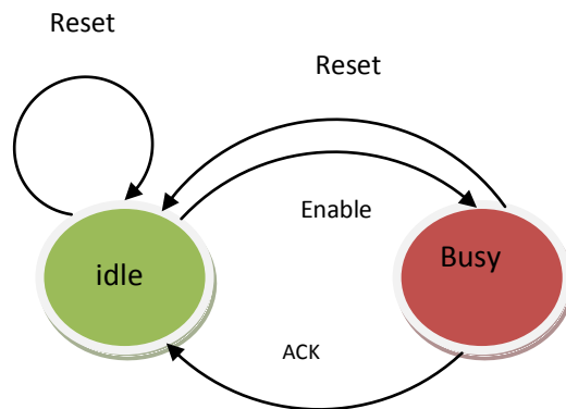
Figure V.18 Diagramme d'état du composant DCT 1D 4x4
