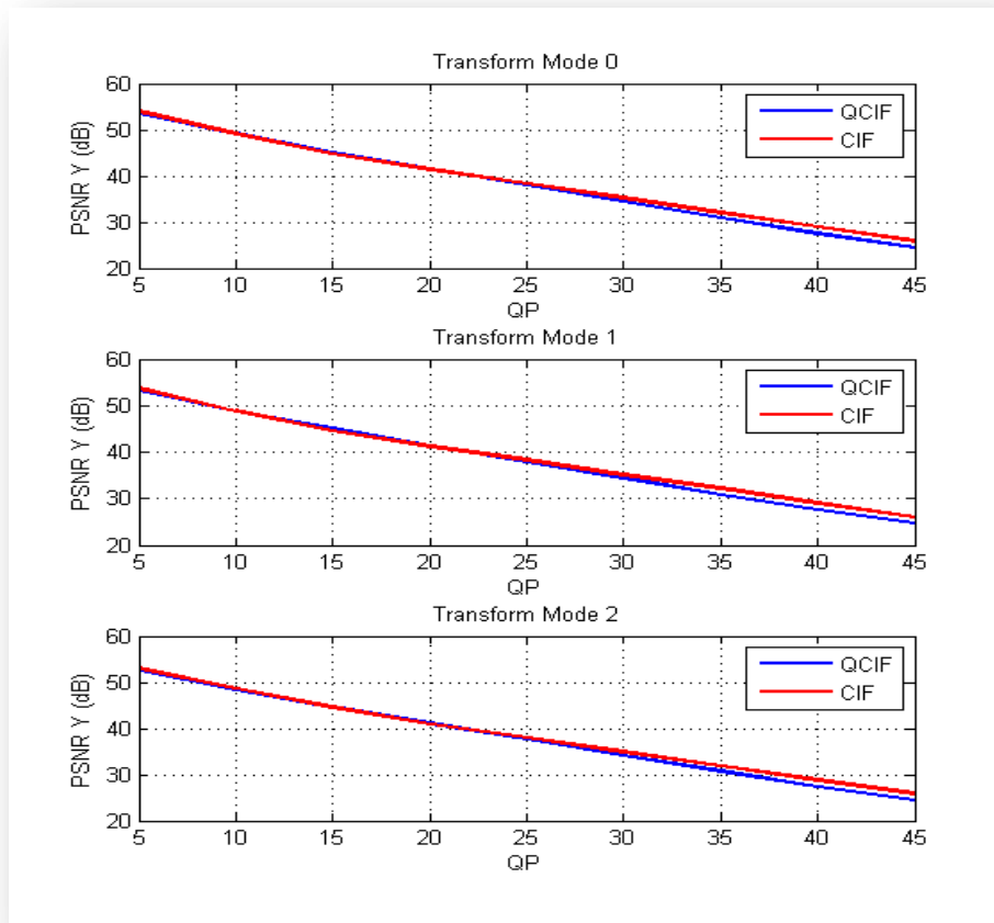
Figure IV.22 Comparaison de la qualité obtenue avec le format QCIF et CIF selon les 3 modes de transformation spatiale
