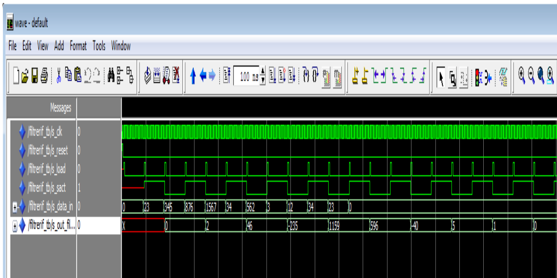
Figure V.11 Données filtrées par le filtre passe haut à 7 coefficients et 12 bits de résolution.
