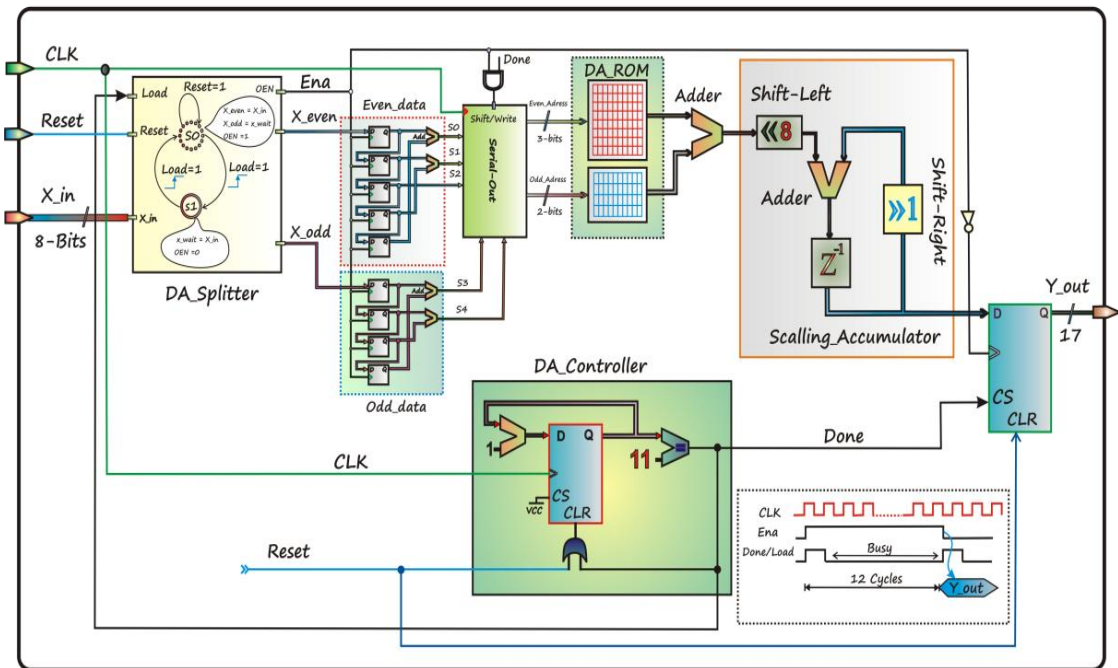
Figure V.8 Schéma synoptique de l'implémentation du filtre passé bas à 9 coefficients et une résolution de 8 bits.
