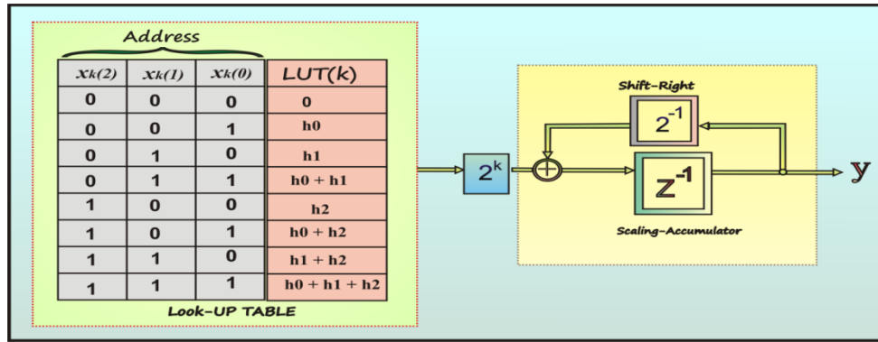
Figure V.6 Implémentation de la technique d'AD à base de LUT.
