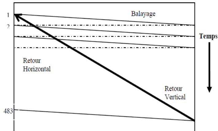
Figure I.4 Principe de balayage utilisé pour la vidéo et la télévision
