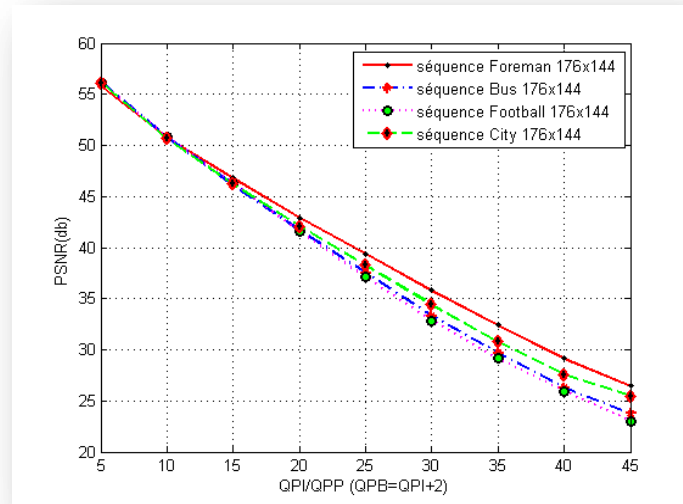
Figure IV.14(a) PSNR de différentes séquences vidéo.
