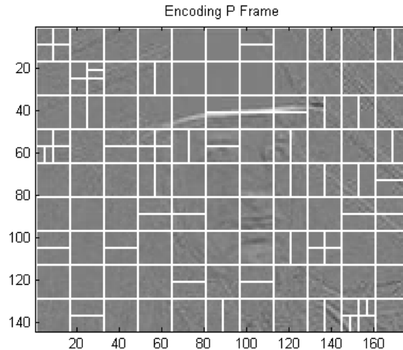
Figure II.11 Codage d'une image (frame) en utilisant différentes partitions.
