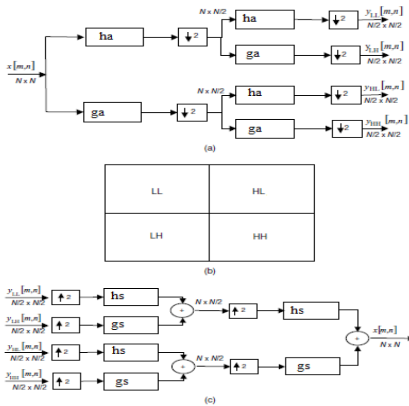
Figure III.6 Un niveau de DWT 2D. (a) 2D DWT décomposition, (b) emplacement des approximations et des détails, (c) 2D DWT reconstruction.
