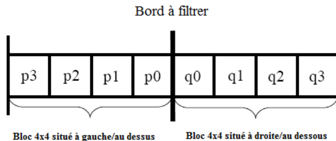
Figure II.18 Convention de nomination des pixels des bords des blocs impliqués dans l'opération de filtrage.
