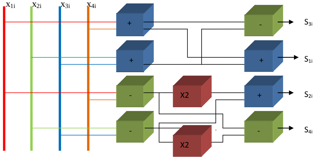
Figure V.15 Diagramme de calcul de la DCT entière 1D 4x4
