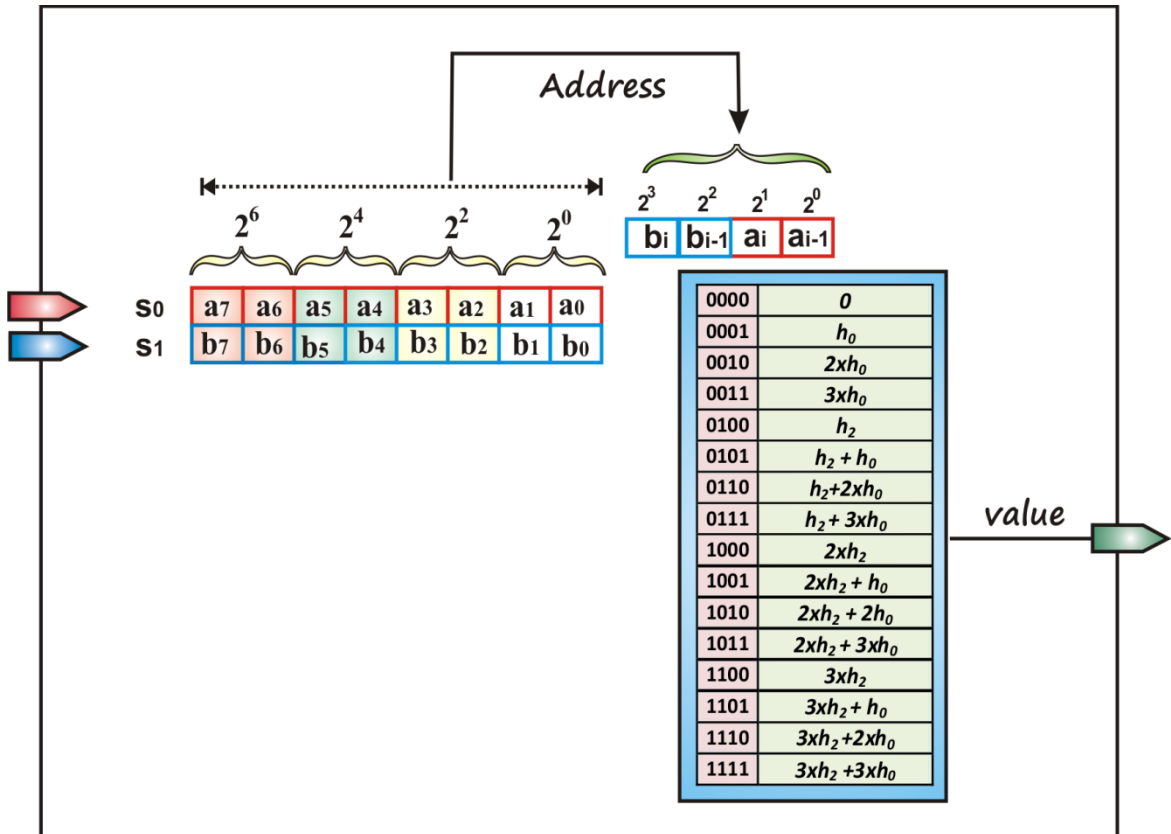
Figure V.9 La partie MDA LUT paire.
