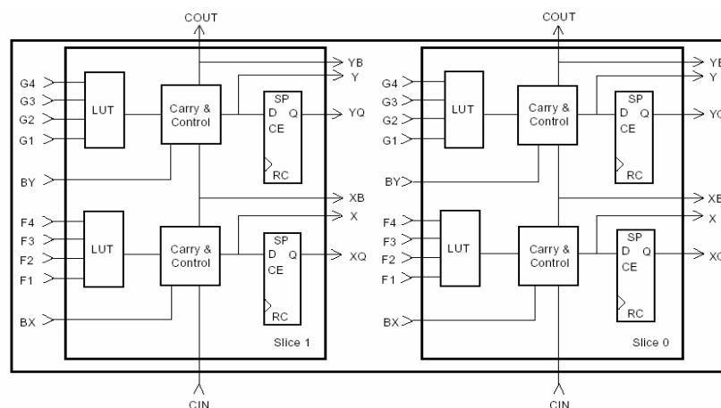
Figure V.2 Structure d'un élément logique.
