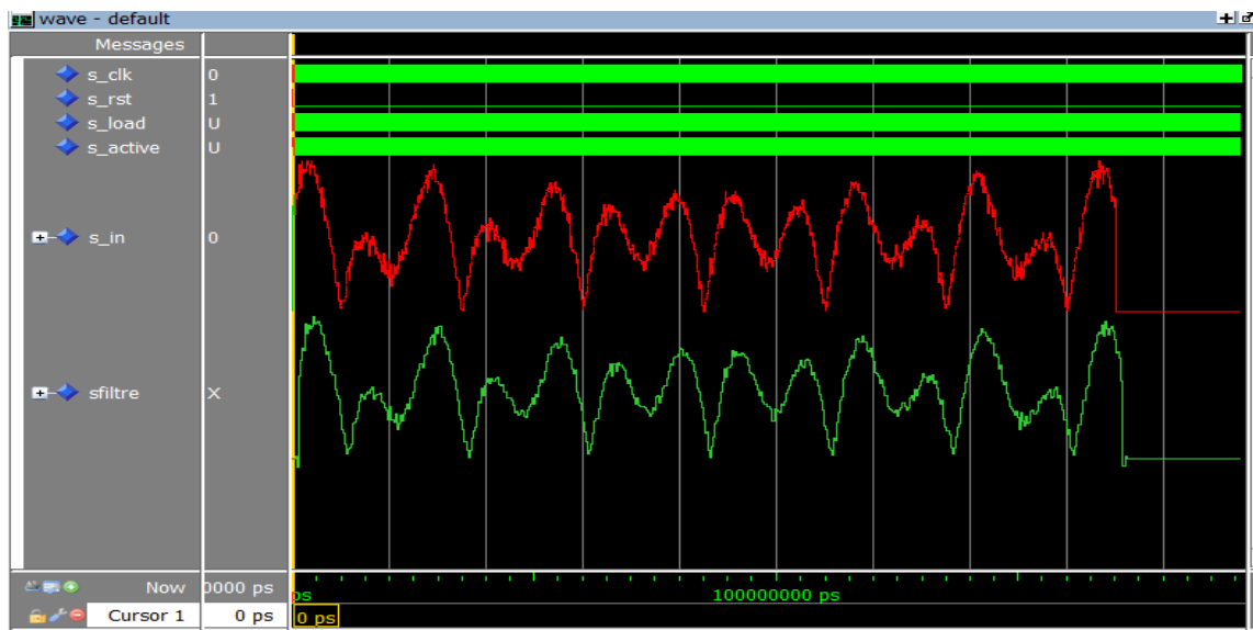
Figure V.12 Résultat de simulation avec Modelsim. Signal bruité (en haut) , signal filtré ou approximation (en bas).
