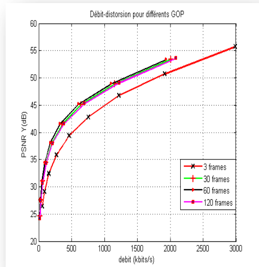
Figure IV.12(d) Courbes R-D pour différents GOP.
