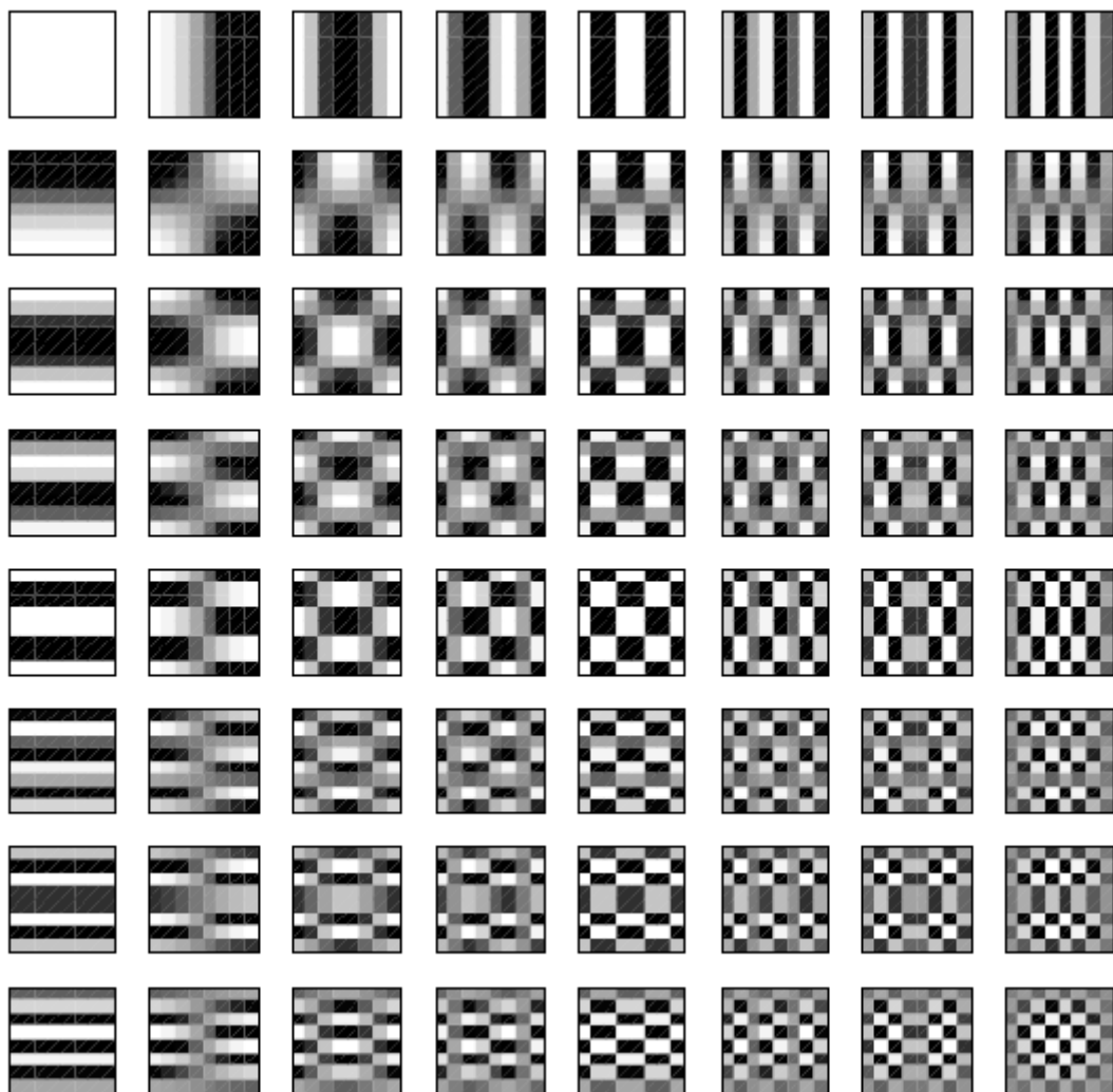
Figure III.3 Les images de base de la DCT 8x8.
