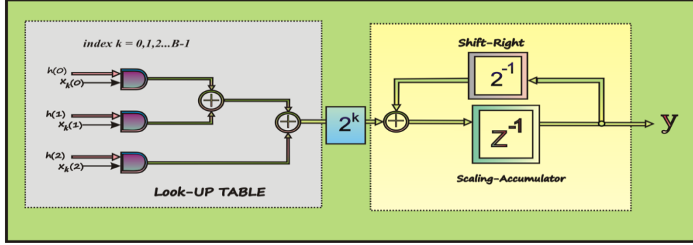
Figure V.5 Structure du noyau d'un multiplieur à base d'arithmétique distribuée.
