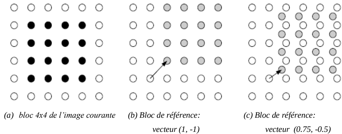
Figure II.12 Exemple de prédiction entière et sous-pixélique.
