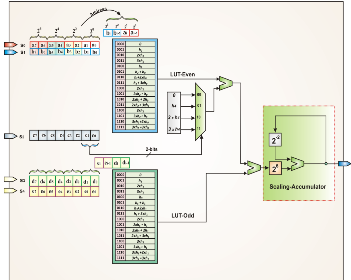
Figure V.10 Diagramme bloc de l'architecture à base de MDA.
