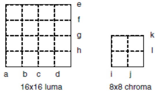
Figure II.17 Les bords à filtrer dans un macrobloc.
