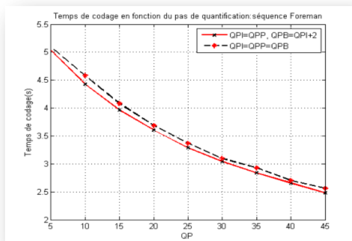
Figure IV.7(c) Temps de codage (QPI=QPP=QPB) et Temps de codage (QPI=QPP=QPB-2)(cas de 3 frames)
