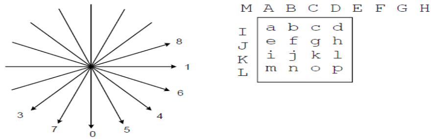
Figure II.6 Récapitulation des modes de prédiction d'un bloc 4x4.
