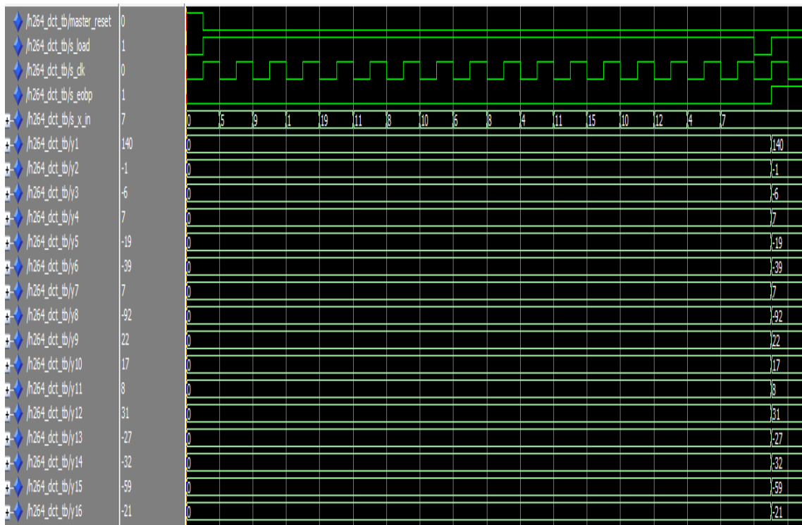
Figure V.23.b Résultat de la simulation de la DCT 2D entière 4x4 (un bloc 4x4)
