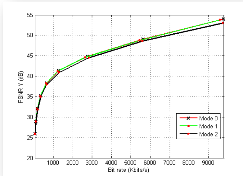
Courbe débit-distorsion
