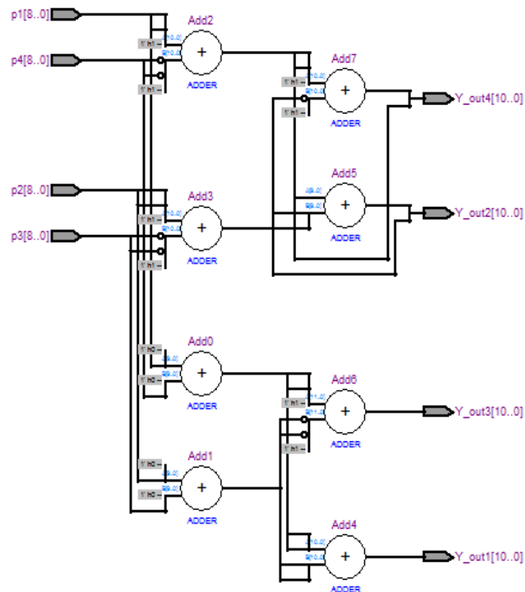
Figure V.30 Vue RTL du circuit DCT 4x4 1D
