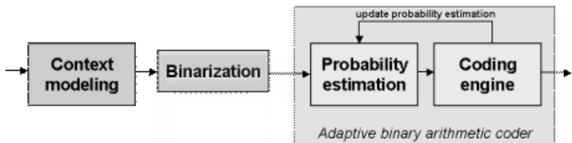
Figure II.8 Schéma synoptique du codage CABAC [55]
