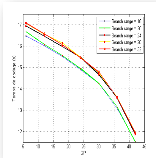
Figure IV.11(c) Temps de codage pour différents search range (séquence Football)
