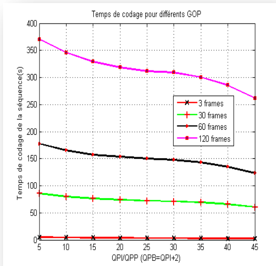
Figure IV.12(c) Temps de codage en fonction du pas de quantification pour différents GOP.
