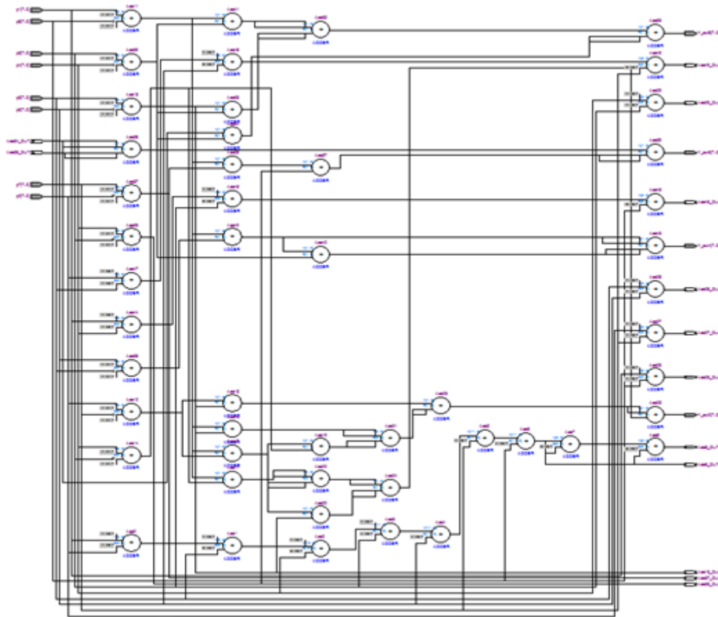
Figure V.33 Vue RTL du circuit DCT 8x8 classique 1D (partie 2/2)
