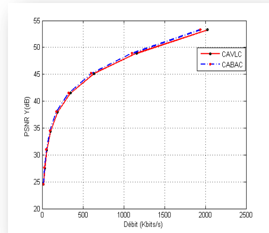
Figure IV.9(d) PSNR en fonction du débit (CABAC vs CAVLC)
