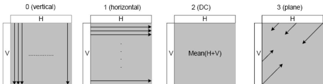
Figure II. 4 Modes d'intra-prédiction d'un bloc de luminance 16x16.
