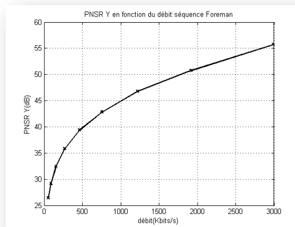
Figure IV.5(c) PSNR de Y en fonction du débit
