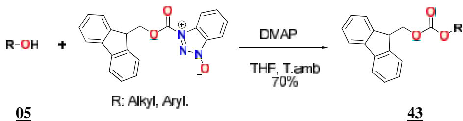
Schéma 34: Protection O-Fmoc par 1,1-bis[6-(trifluorométhyl)benzotriazolyl] carbonate (BTBC)
