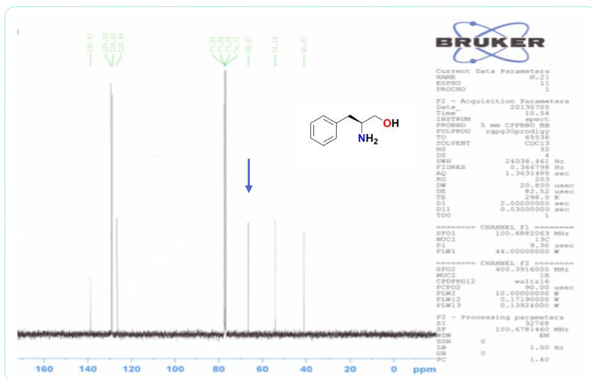
Figure 57: Spectre RMN 13 C de l'acido alcool phénylalanine ( 164-a )
