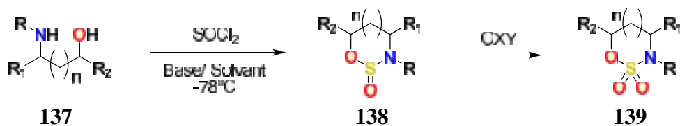
Schéma 55 : Synthèse de sulfamidates à partir de l'intermédiaire cyclosulfamidite
