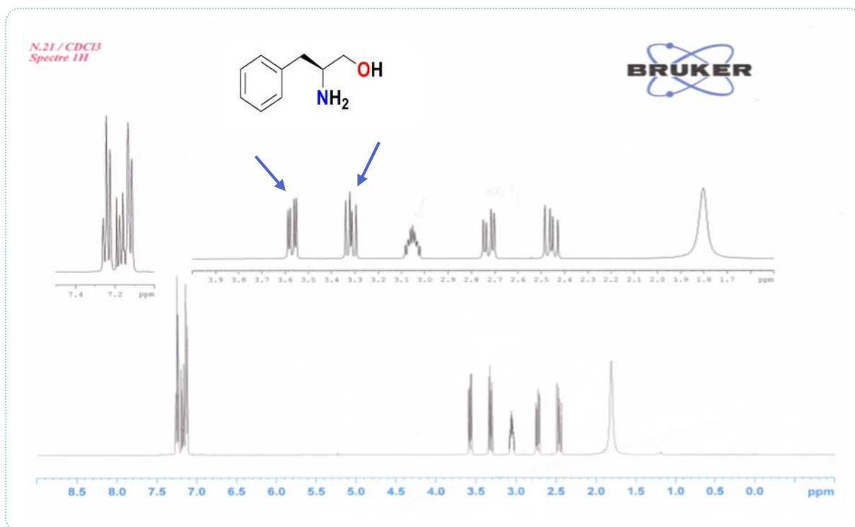
Figure 56: Spectre RMN 1 H de l'acido alcool phénylalanine ( 164-a )
