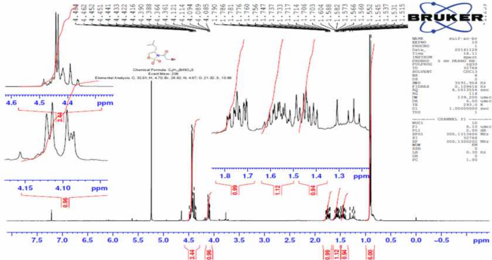
Specre RMN du ^1\text{H} : Composé 172-b.
