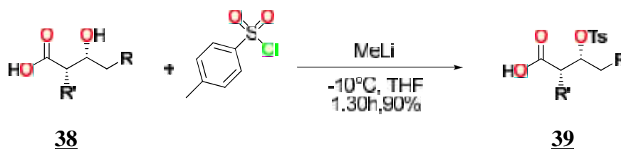
Schéma 31 : Tosylation de la fonction hydroxyle à basse température.
