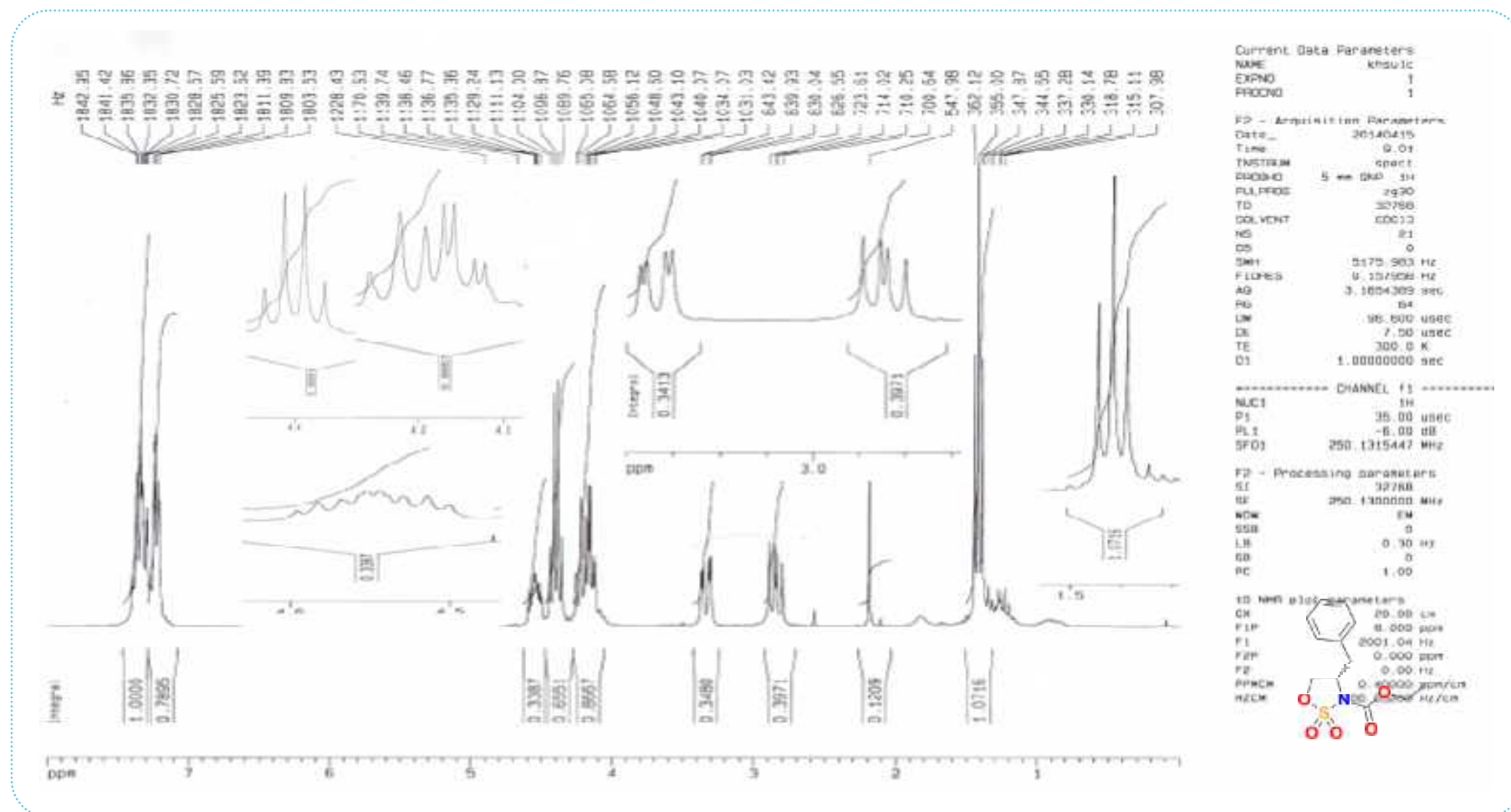
Spectre RMN du ^1\text{H} : Composé 168-a .
