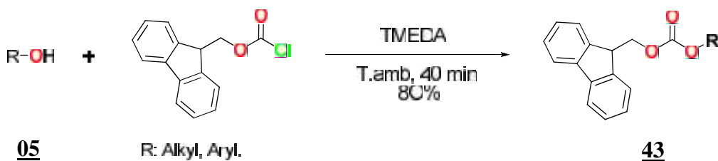
Schéma 33 : Protection de la fonction hydroxyle avec 9-fluorenylméthoxycarbonyl
