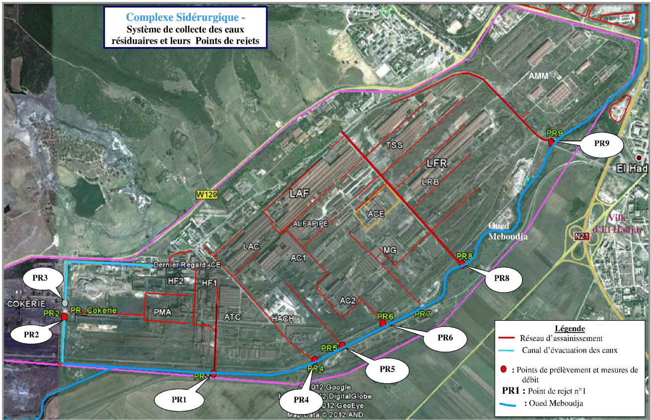
Figure 67 : Situation géographique et Système de collecte des eaux résiduaires- Complexe sidérurgique
