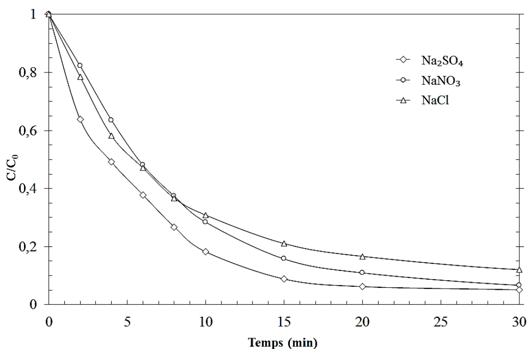
Figure III-4 : Effet de la nature de l'électrolyte support sur la dégradation de l'OG par le procédé électro-Fenton (Conditions expérimentales : [OG] 0 = 0,04 mM ; [Fe 2+ ] 0 = 0,03 mM ; [électrolyte] = 0,05 M ; pH = 3 ; T = 20 ± 1 °C ; V = 150 mL ; I = 100 mA).
