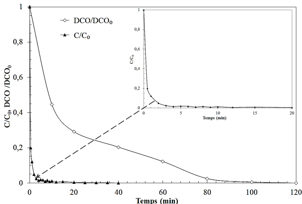
Figure II-14 : Dégradation et variation de la DCO d'une solution de l'OG lors du traitement par le réactif de Fenton (Conditions expérimentales : [OG]_0 = 0,04 \text{ mM} ; [Fe^{2+}]_0 = 0,12 \text{ mM} ; [H_2O_2]_0 = 0,4 \text{ mM} ; T = 30 \pm 1 \text{ }^\circ\text{C} ; \text{pH} = 3,5 ; V_{\text{agitation}} = 240 \text{ tr.min}^{-1} ).
