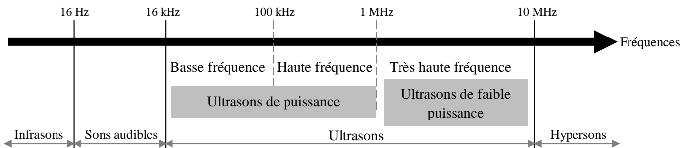
Figure I-8 : Classification des ultrasons en fonction de leur fréquence et de leur puissance [96, 97, 98].
