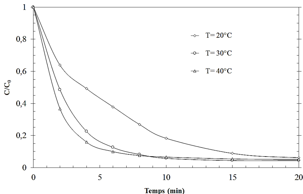
Figure III-10 : Variation de la cinétique de dégradation électrochimique de l'OG en fonction de la température (Conditions expérimentales : [\text{OG}]_0 = 0,04 \text{ mM} ; [\text{Fe}^{2+}]_0 = 0,03 \text{ mM} ; \text{pH} = 3 ; [\text{Na}_2\text{SO}_4] = 0,05 \text{ M} ; T = (20-40) \pm 1^\circ\text{C} ; V = 150 \text{ mL} ; I = 100 \text{ mA} ).
