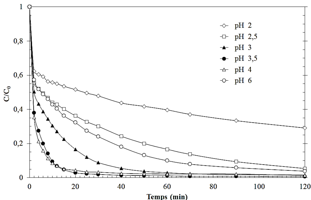
Figure II-6 : Évolution de la cinétique de dégradation de l'OG par le procédé Fenton en fonction du pH initial (Conditions expérimentales : [\text{OG}]_0 = 0,04 mM ; [\text{Fe}^{2+}]_0 = 0,05 mM ; [\text{H}_2\text{O}_2]_0 = 0,2 mM ; T = 30 \pm 1 °C ; \text{pH} = 2-6 ; V_{\text{agitation}} = 240 tr.min -1 ).
