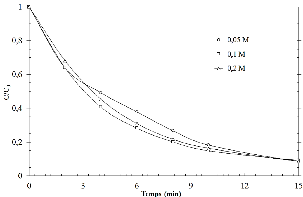
Figure III-5 : Effet de la concentration de l'électrolyte support sur la dégradation de l'OG par le procédé électro-Fenton (Conditions expérimentales : [OG]_0 = 0,04 mM ; [Fe^{2+}]_0 = 0,03 mM ; [Na_2SO_4] = 0,05-0,2 M ; pH = 3 ; T = 20 \pm 1 °C ; V = 150 mL ; I = 100 mA).
