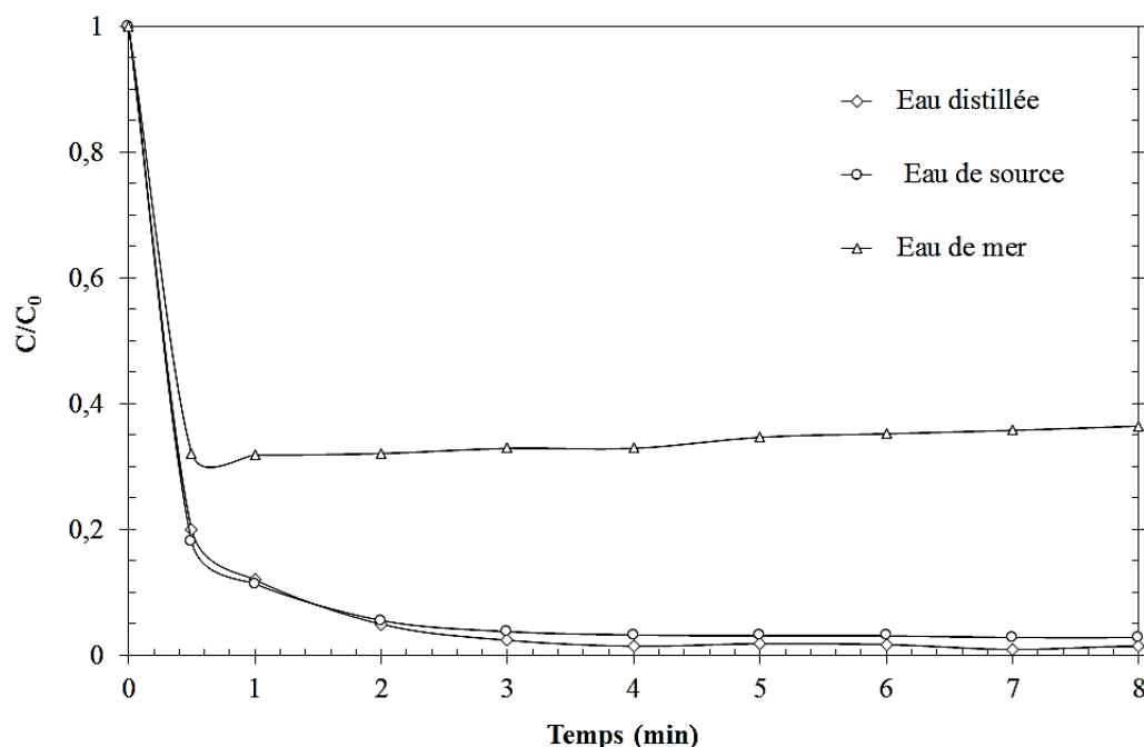
Figure II-15 : Dégradation de l'OG dans l'eau distillée, l'eau de source naturelle et l'eau de mer par le réactif de Fenton (Conditions expérimentales : [\text{OG}]_0 = 0,04 \text{ mM} ; [\text{Fe}^{2+}]_0 = 0,12 \text{ mM} ; [\text{H}_2\text{O}_2]_0 = 0,4 \text{ mM} ; T = 30 \pm 1 \text{ }^\circ\text{C} ; \text{pH} = 3,5 ; V_{\text{agitation}} = 240 \text{ tr.min}^{-1} ).
