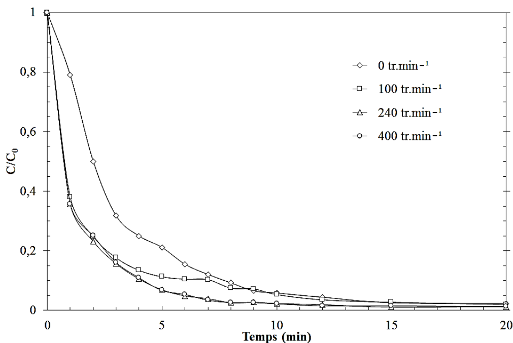
Figure II-8 : Variation de la cinétique de dégradation de l'OG par le procédé Fenton en fonction de la vitesse d'agitation (Conditions expérimentales : [OG]_0 = 0,04 mM ; pH = 3,5 ; [Fe^{2+}]_0 = 0,05 mM ; [H_2O_2]_0 = 0,2 mM ; T = 30 \pm 1 °C ; V_{agitation} = 0-400 tr.min -1 ).
