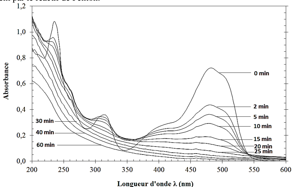
Figure II-13 : Changements dans les spectres d'absorption UV-visible de l'OG au cours de traitement par le réactif de Fenton (Conditions expérimentales : [OG] 0 = 0,04 mM ; [Fe 2+ ] 0 = 0,12 mM ; [H 2 O 2 ] 0 = 0,4 mM ; T = 30 ± 1 °C ; pH = 3,5 ; V agitation = 240 tr.min -1 ).
