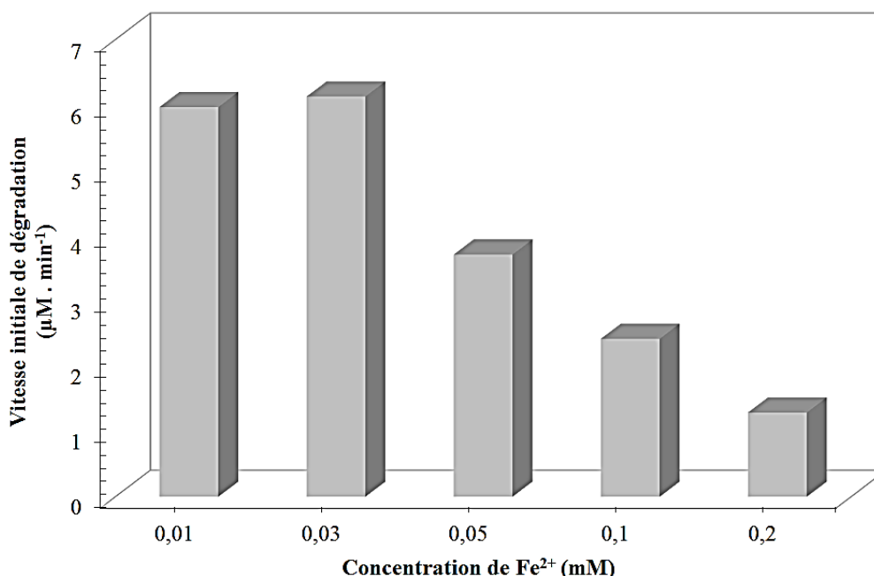
Figure III-9 : Effet de la concentration initiale de \text{Fe}^{2+} sur la vitesse initiale de dégradation électrochimique de l'OG (Conditions expérimentales : [\text{OG}]_0 = 0,04 mM ; [\text{Fe}^{2+}]_0 = 0,01-0,2 mM ; pH = 3 ; [\text{Na}_2\text{SO}_4] = 0,05 M ; T = 20 \pm 1 °C ; V = 150 mL ; I = 100 mA).
