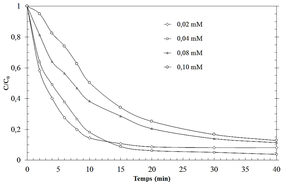
Figure III-11 : Effet de la concentration initiale de l'OG sur la cinétique de dégradation (Conditions expérimentales : [\text{OG}]_0 = 0,02-0,1 \text{ mM} ; [\text{Fe}^{2+}]_0 = 0,03 \text{ mM} ; \text{pH} = 3 ; [\text{Na}_2\text{SO}_4] = 0,05 \text{ M} ; T = 20 \pm 1^\circ\text{C} ; V = 150 \text{ mL} ; I = 100 \text{ mA} ).
