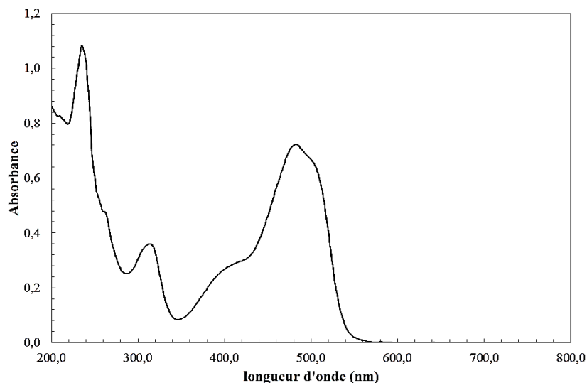
Figure II-2 : Spectre d'absorption UV-visible de l'Orange G en solution aqueuse
