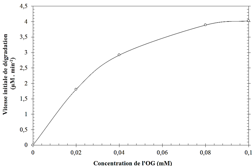
Figure III-12 : Variation de la vitesse initiale de dégradation en fonction de la concentration initiale de l'OG (Conditions expérimentales : [OG]_0 = 0,02-0,1 mM ; [Fe^{2+}]_0 = 0,03 mM ; pH = 3 ; [Na_2SO_4] = 0,05 M ; T = 20 \pm 1 °C ; V = 150 mL ; I = 100 mA).
