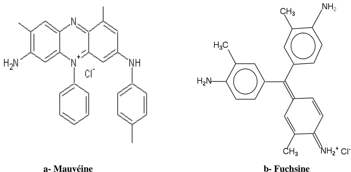
Figure I-1 : Structure chimique de la Mauvéine (a) et de la Fuchsine (b) [4]
