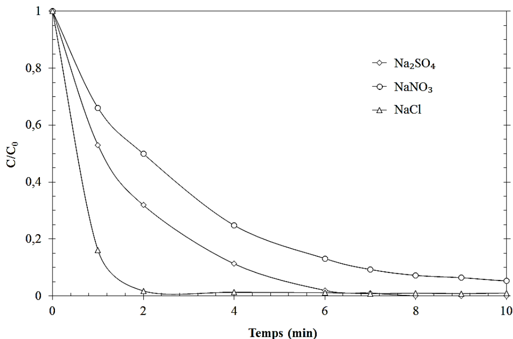
Figure IV-13 : Effet de la nature de l'électrolyte support sur la dégradation de l'OG par le procédé sono-électro-Fenton (Conditions expérimentales : [OG]_0 = 0,04 mM ; [Fe^{2+}]_0 = 0,05 mM ; T = 20 \pm 1 °C ; I = 100 mA ; pH = 3 ; [électrolyte] = 0,05 M ; V = 150 mL ; puissance ultrasonore = 15 W ).
