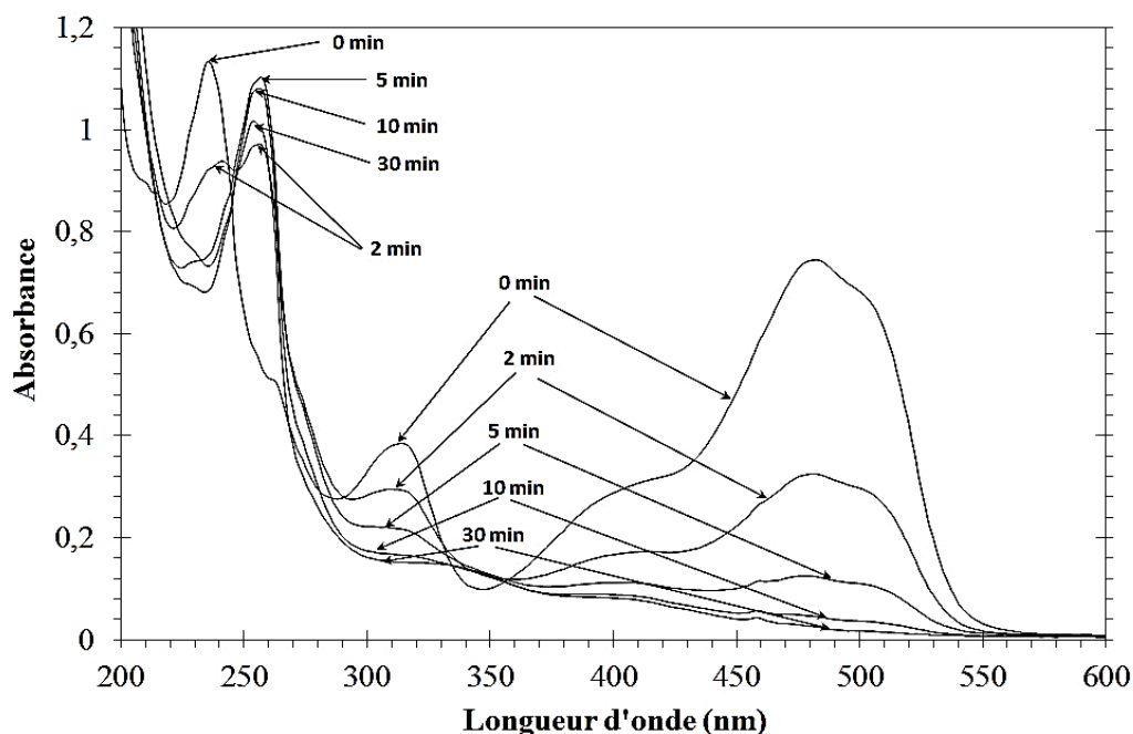
Figure IV-5 : Suivi des spectres d'absorption UV-visible de l'OG lors du traitement par le procédé sono-électro-Fenton (Conditions expérimentales : [OG]_0 = 0,04 mM ; V = 150 mL ; puissance ultrasonore = 15 W ; [Fe^{2+}]_0 = 0,05 mM ; pH = 3 ; [Na_2SO_4] = 0,05 M ; T = 20 \pm 1 °C ; I = 100 mA).
