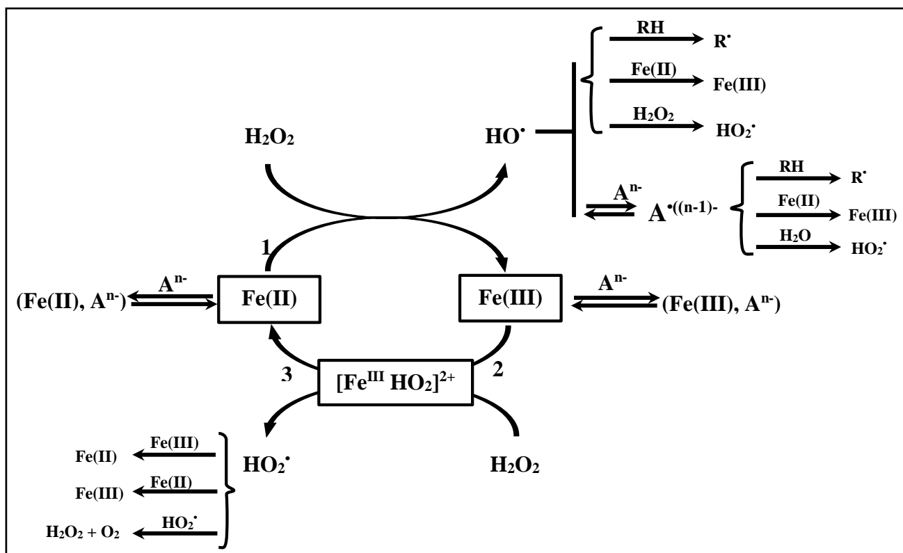
Figure I-5 : Schéma réactionnel simplifié du système Fenton en milieu acide A n- : anion inorganique (Cl - , SO 4 2- , H 2 PO 4 - /HPO 4 2- , etc....), RH : composé organique [71].
