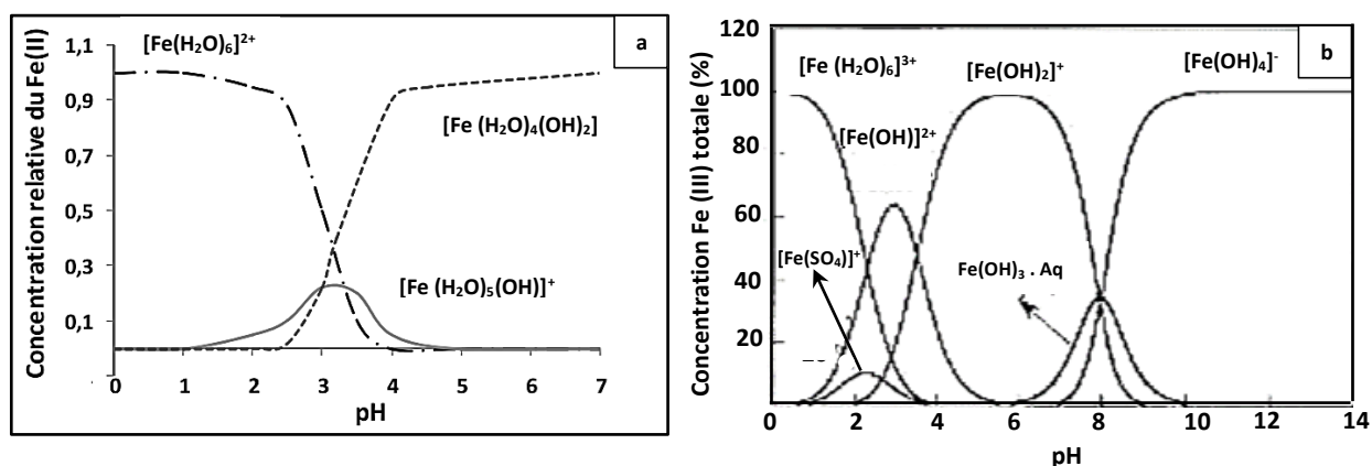
Figure II-7 : Spéciation des espèces de Fe (II) et Fe (III) en fonction du pH à T = 25\text{ }^\circ\text{C} , [\text{Fe}(\text{II})] = [\text{Fe}(\text{III})] = 1\text{ mM} [41, 42]
