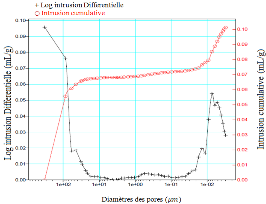
Figure 3.40. Distribution de la taille des pores de micro-béton de résine à base de fibre de verre obtenue par PIM.
