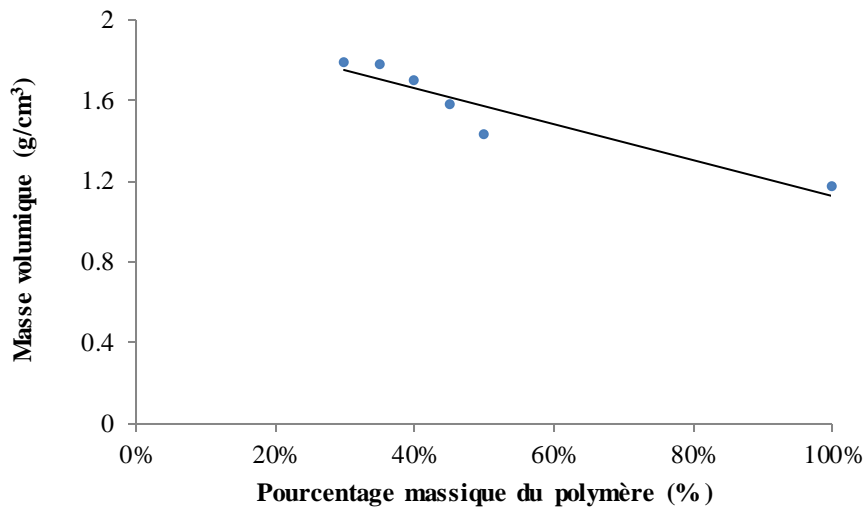
Figure 3.4. Evolution de la masse volumique du mortier de résine en fonction du pourcentage du polyester avec sable fin.
