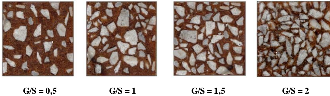
Figure 3.30. Morphologie de rupture des micro-bétons de résine pour les différents rapports G/S.
