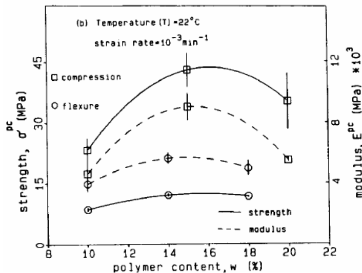
Figure 1.12. Résistances en Fonction de la quantité de polymère [61].
