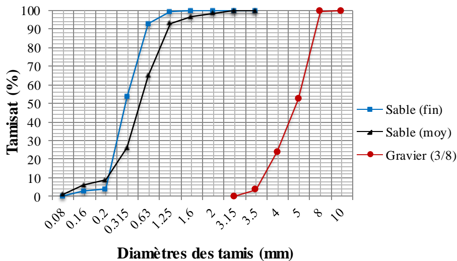
Figure 2.7. Courbes granulométriques des granulats.
