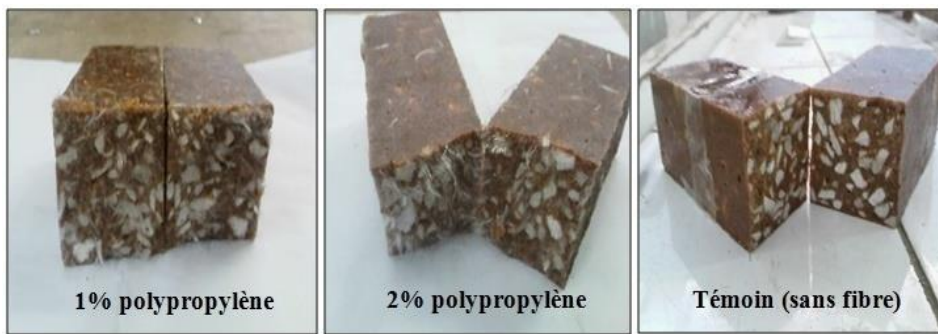
Figure 3.43. Mode de rupture des éprouvettes en flexion de béton de résine fibré.
