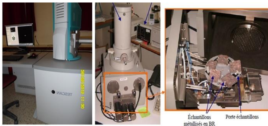
Figure 2.18. Microscope électronique à balayage et porte échantillons.
