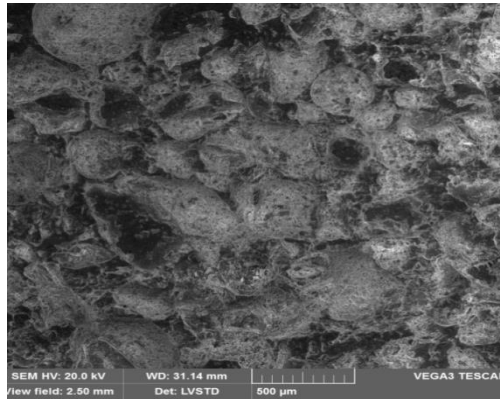
Figure 3.23. Micrographie MEB de mortier de résine optimal (80% sable fin et 20% sable moyen avec 35% de résine) agrandies 100x.
