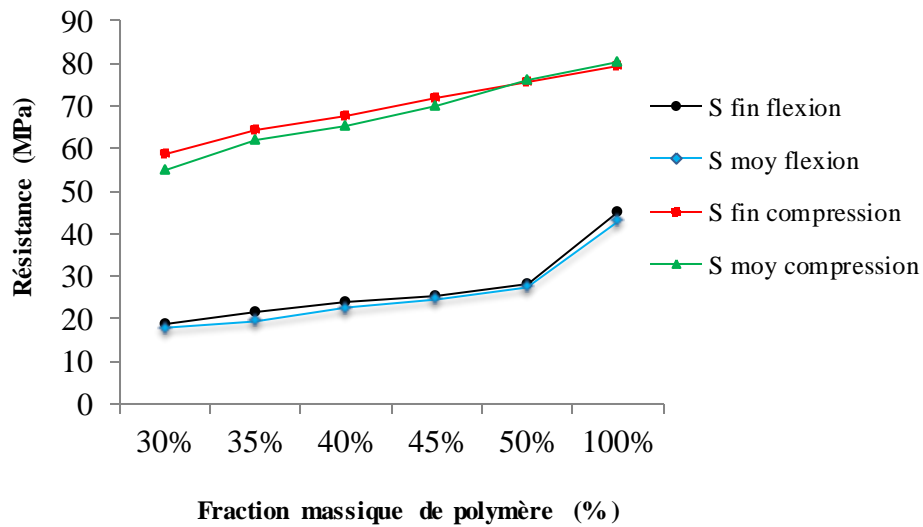
Figure 3.7. Influence de pourcentage de résine sur les résistances mécaniques traction par flexion et compression.
