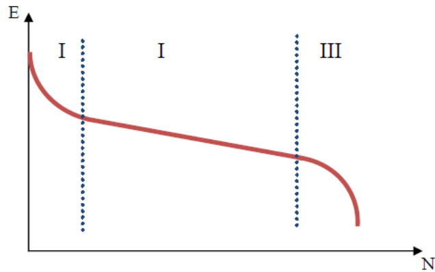
Figure 1.19. Evolution du module d'élasticité et distinction de trois phases différentes dans un essai de fatigue [97].
