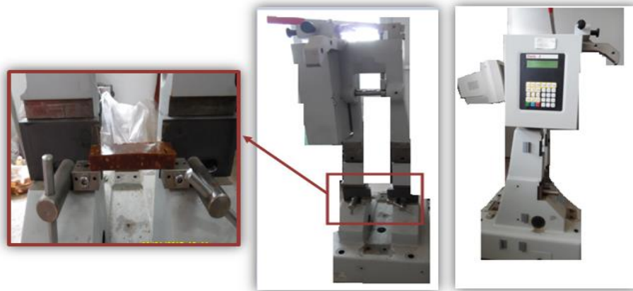
Figure 2.14. Machine d'essai Charpy avec affichage numérique.
