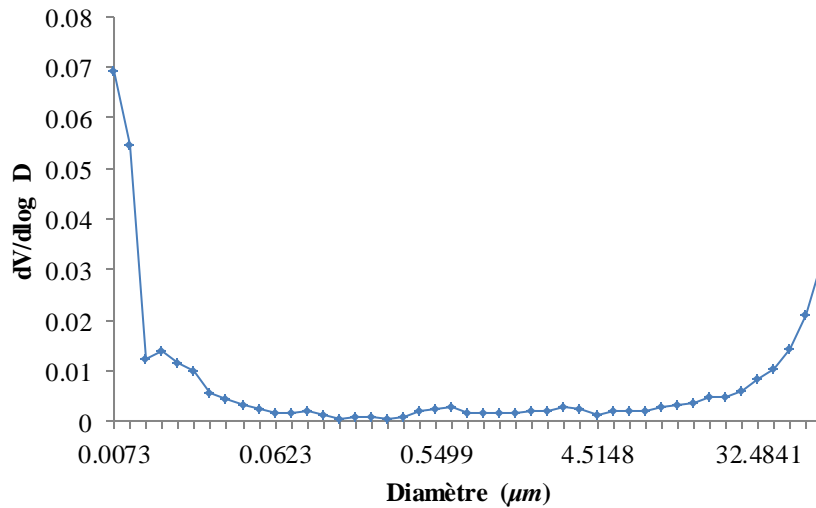
Figure 3.20. Distribution des pores de mortier de résine optimal.
